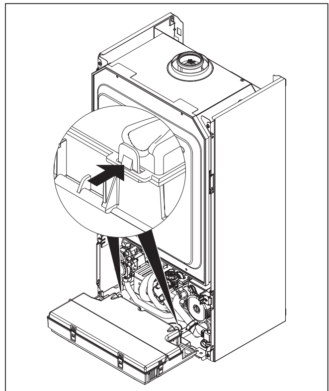
Fig. 5.7 Abrir la pared trasera de la caja de distribución
