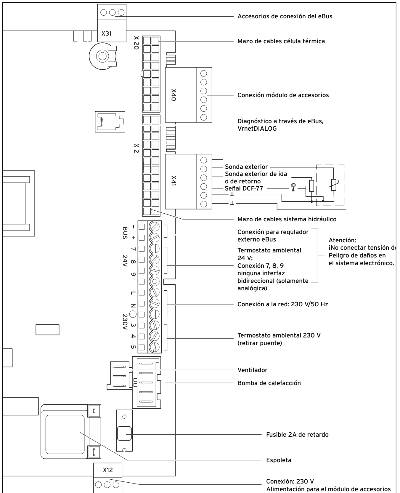
Fig. 5.9 Plan de conexiones turboTEC plus/turboTEC pro
