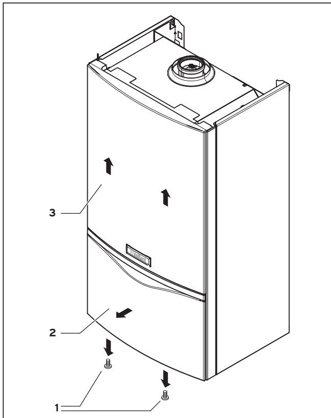
Fig. 4.6 Desmontar el revestimiento frontal del aparato (en esta figura: turboTEC plus)
