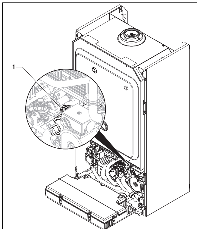
Fig. 7.4 Ajustar válvula del conducto de derivación
