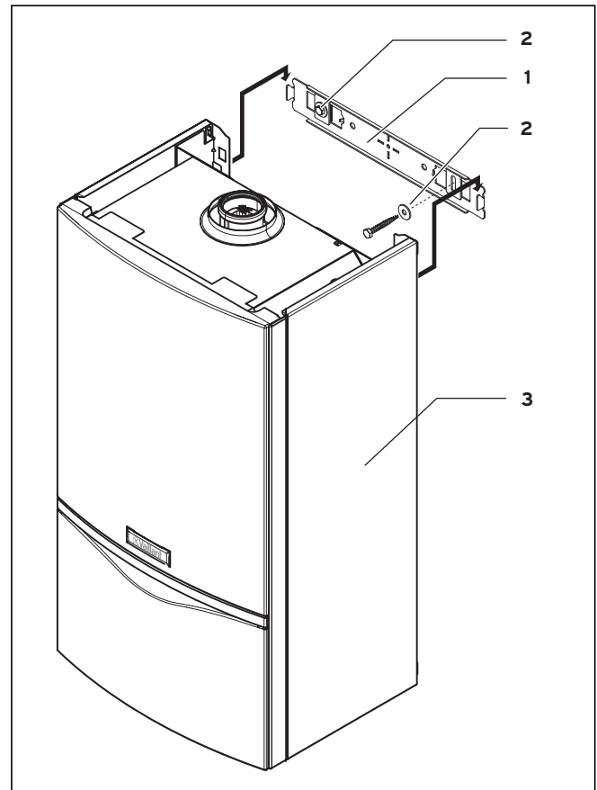
Fig. 4.5 Colgar el aparato (en esta figura: turboTEC plus)
