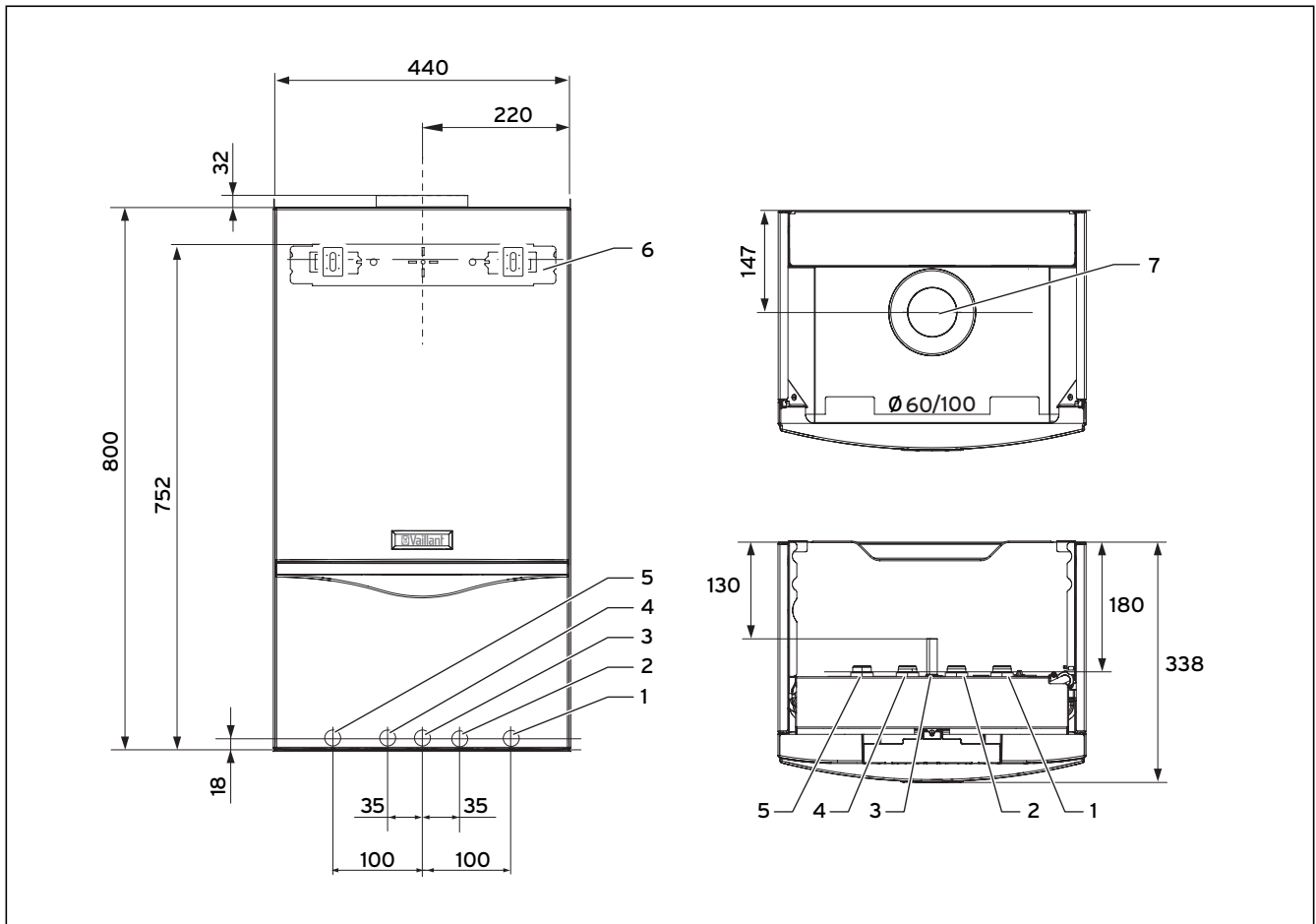
Fig. 4.2 Medidas de conexión en mm (en esta figura: turboTEC plus)
