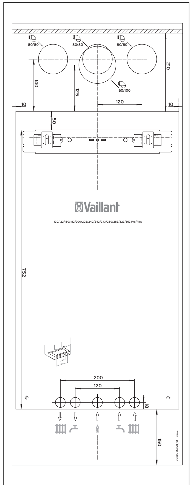
Fig. 4.4 Plantilla de montaje
