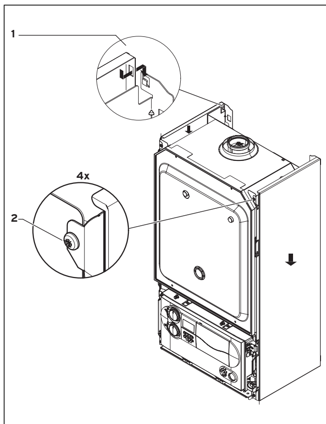
Fig. 4.8 Montar el revestimiento lateral del aparato
