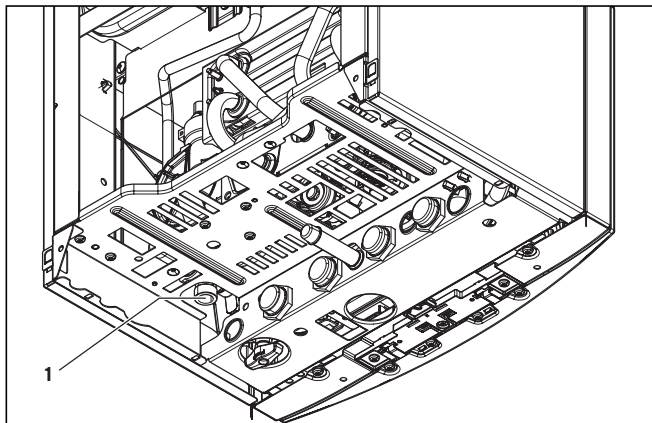
Fig. 5.4 Salida de la válvula de seguridad
