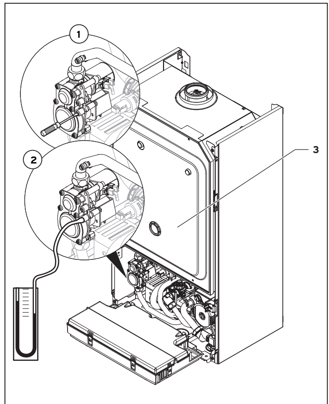
Fig. 6.4 Comprobar la presión de conexión
