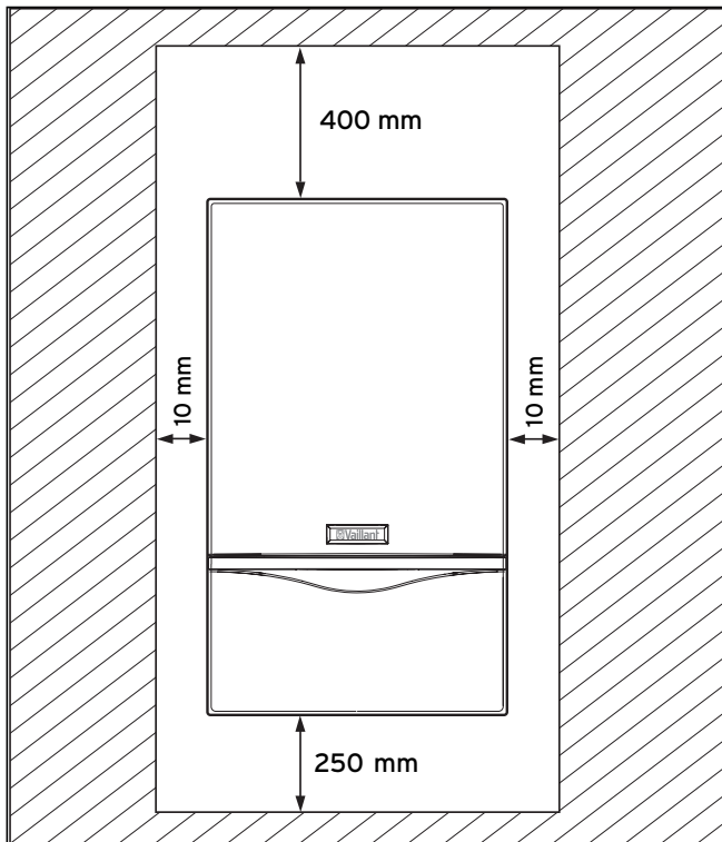
Figura 4.3 Distancias mínimas necesarias/espacios libres para el montaje (en esta figura: turboTEC plus)
