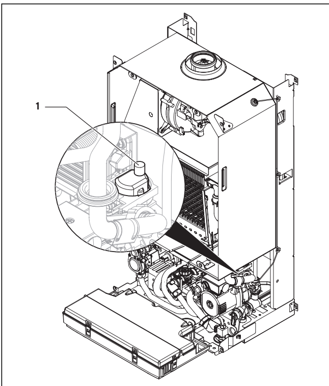
Fig. 6.1 Purgador rápido
