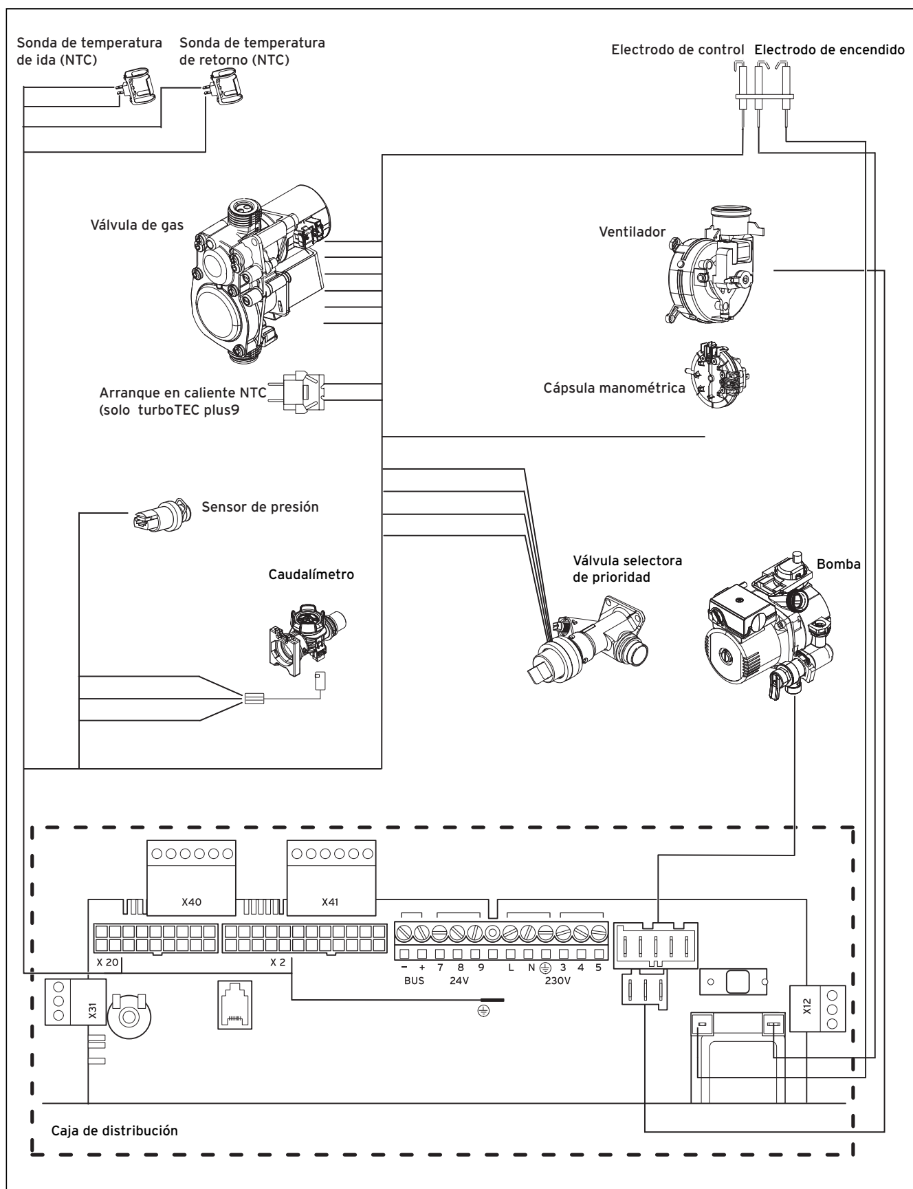
Fig. 5.10 Plan de cableado turboTEC plus/turboTEC pro
