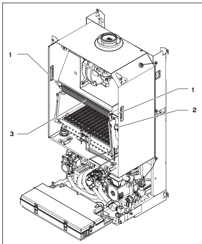
Fig. 8.2 Limpieza del intercambiador de calor primario con desmontaje (suciedad severa)
