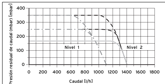
Fig. 7.3 Curva característica de la bomba
