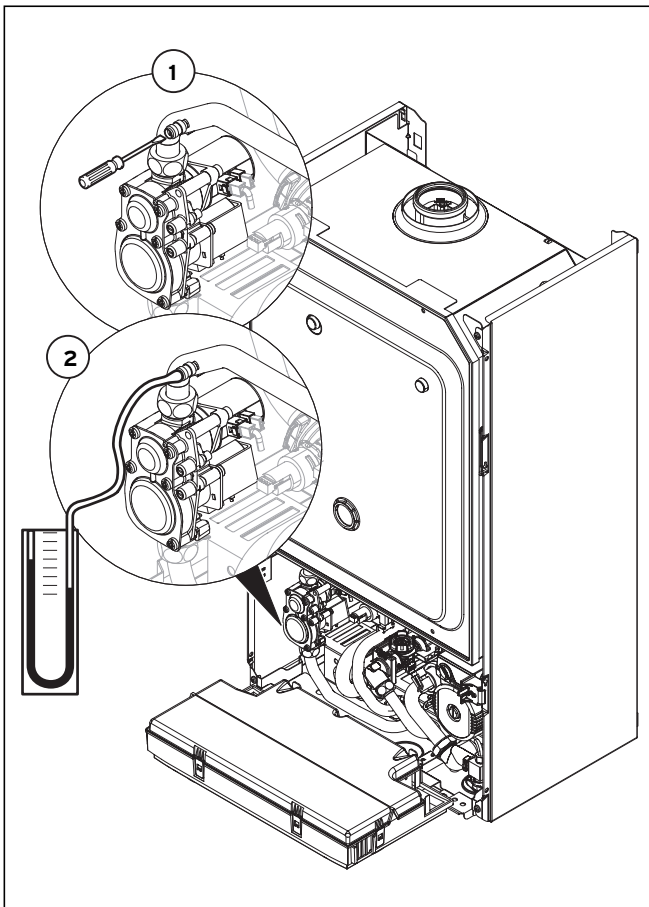
Fig. 6.5 Comprobar la carga nominal
