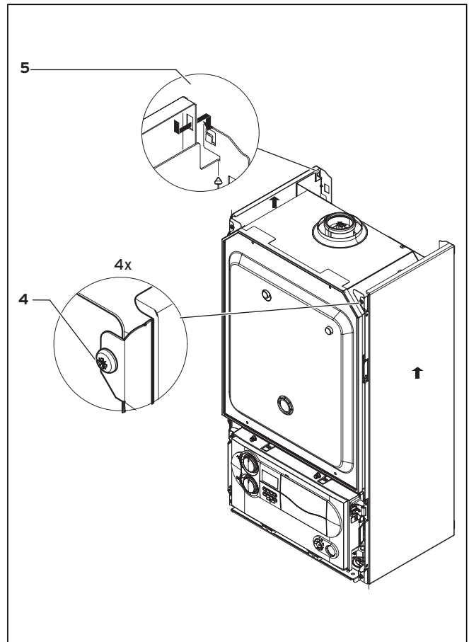
Fig. 4.7 Desmontar el revestimiento lateral del aparato
