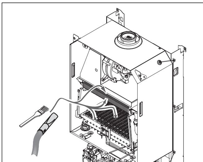
Fig. 8.1 Limpieza del quemador y del intercambiador de calor primario sin desmontar las piezas (suciedad leve)
