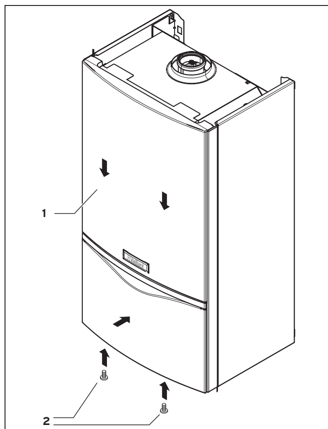
Fig. 4.9 Montar carcasa del aparato (en esta figura: turboTEC plus)
