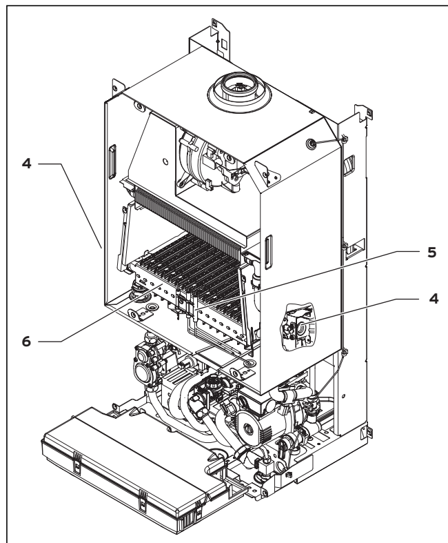
Fig. 8.3 Limpieza del quemador con desmontaje (suciedad severa)
