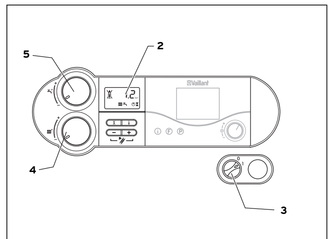
Fig. 6.2 Controlar la presión de llenado de la instalación de calefacción (en esta figura: turboTEC plus)
