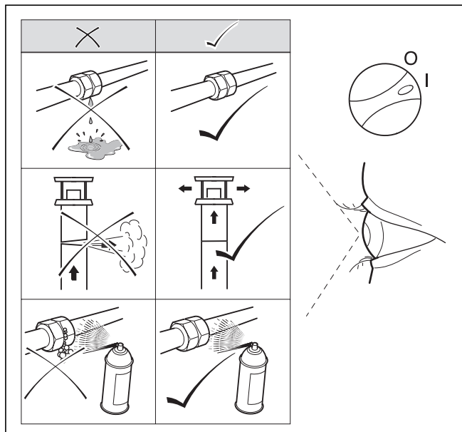
Fig. 8.4 Comprobar la función
