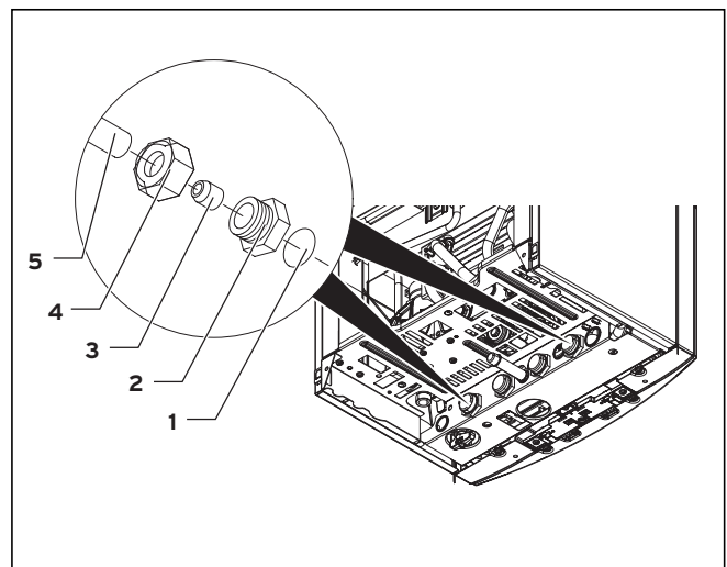
Fig. 5.3 Montar el avance y el retroceso de la calefacción
