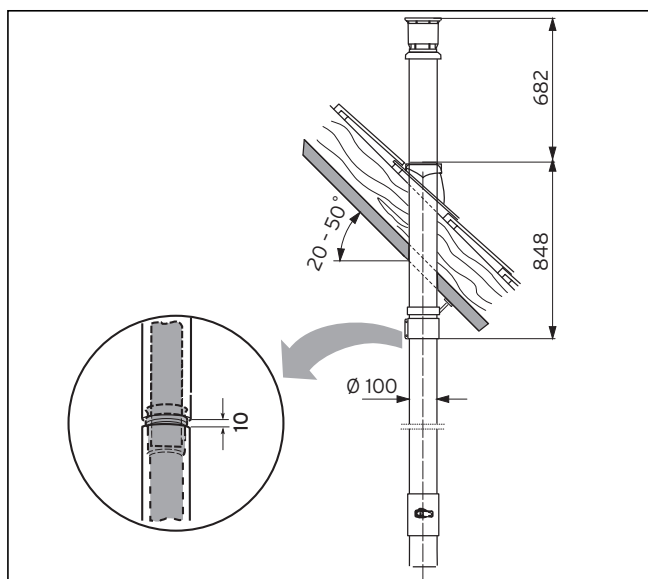
Fig. 5.5 Ejemplo de montaje: Salida vertical a través del tejado
