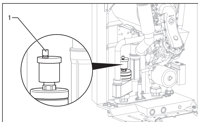
Fig. 8.2 Purgador rápido
