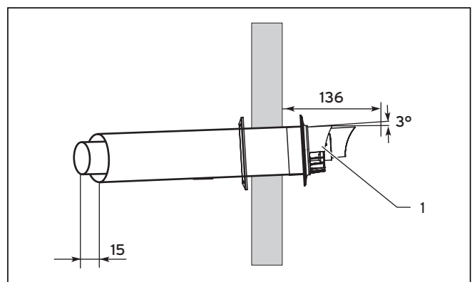
Fig. 6.6 Salida horizontal a través de la pared
