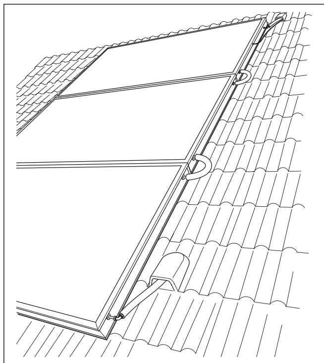
Fig. 2.4 Campo del colector de 3 HelioPLAN SRD 2.3 en montaje sobre tejado
