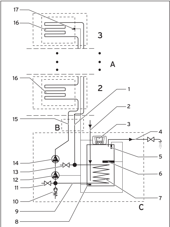
Fig. 2.3 Componentes principales del sistema HelioSet con acumulador S-FE 350 SE P (esbozo básico sin accesorios de conexión)
