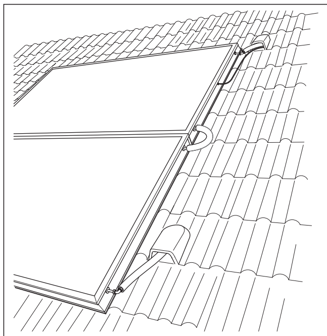
Fig. 2.5 Campo del colector de 2 HelioPLAN SRD 2.3 en montaje sobre tejado
