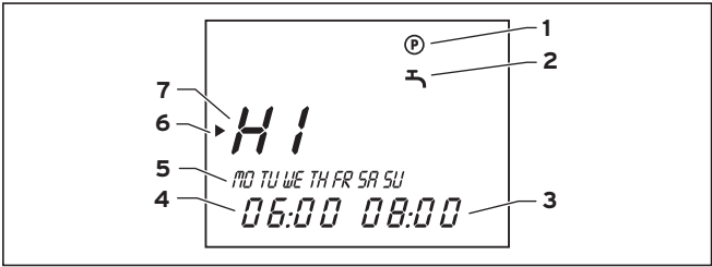
Fig. 4.5 Pantalla niveau de programmation
