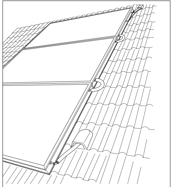
Fig. 2.6 Campo del colector de 3 HelioPLAN SRD 2.3 en montaje sobre tejado
