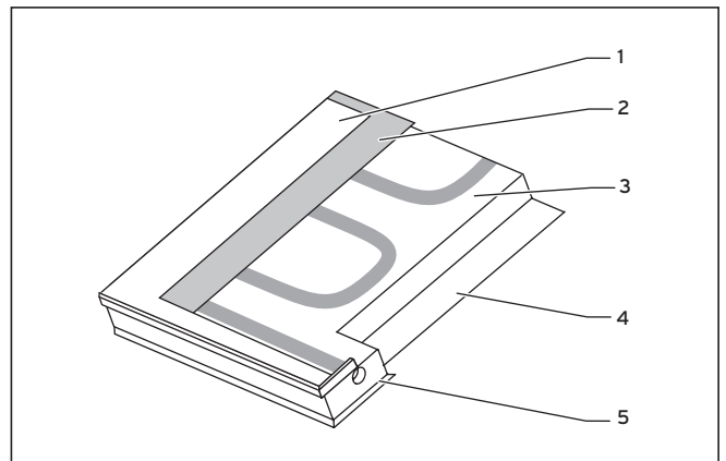
Fig. 2.7 Corte transversal del colector plano Saunier Duval HelioPLAN SRD 2.3
