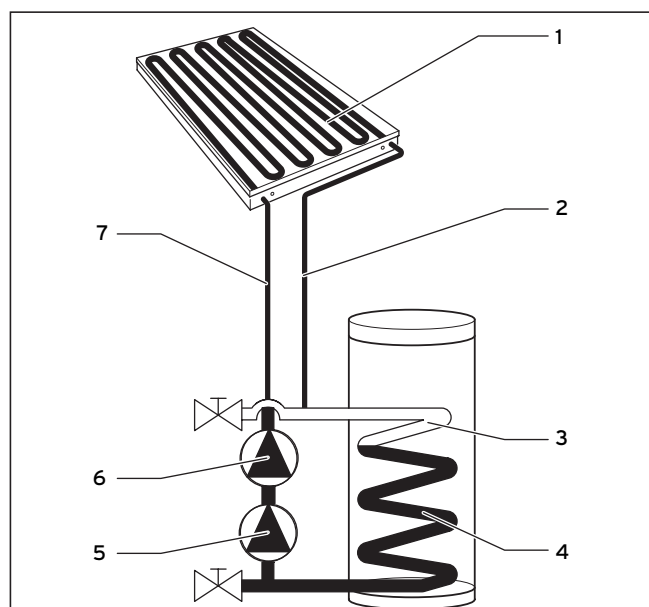
Fig. 2.2 Reparto del líquido solar con bomba/s del colector en funcionamiento
