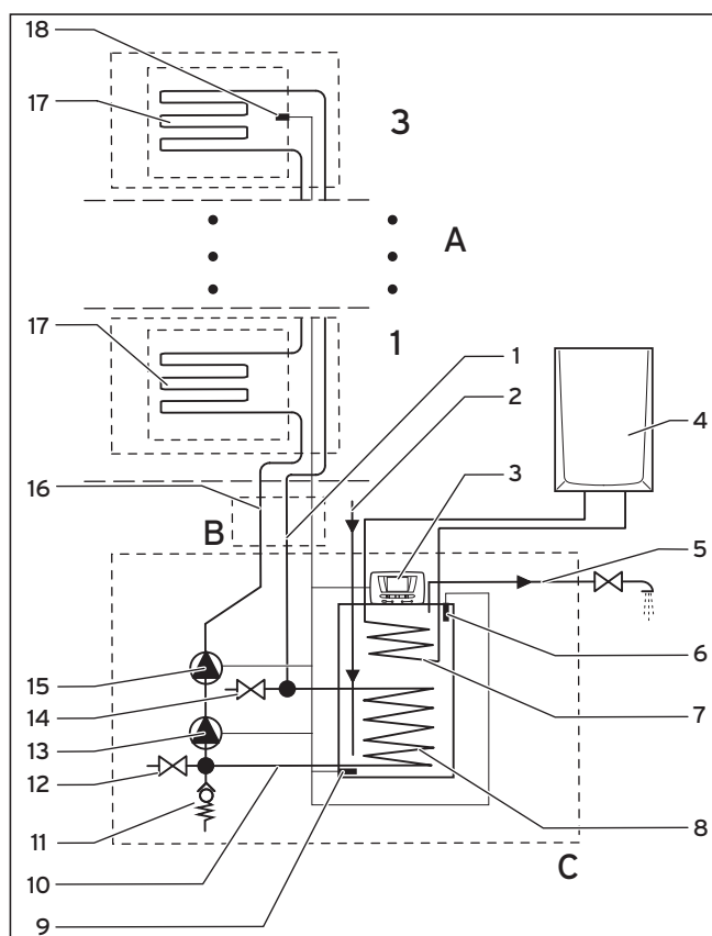
Fig. 2.3 Componentes principales del sistema HelioSet con acumulador S-FE 250/3 SC P (esbozo básico sin accesorios de ventilación)
