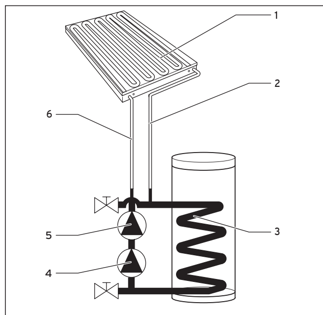
Fig. 2.1 Reparto del líquido solar durante el periodo de inactividad de la/s bomba/s del colector
