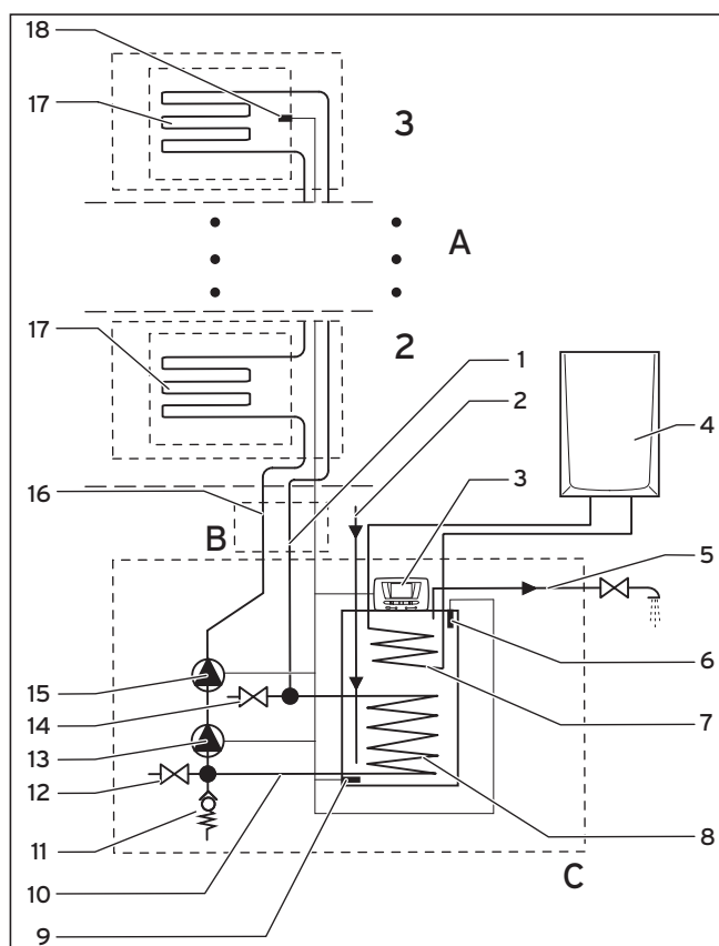
Fig. 2.3 Componentes principales del sistema HelioSet con acumulador S-FE 350/3 SC P (esbozo básico sin accesorios de ventilación)
