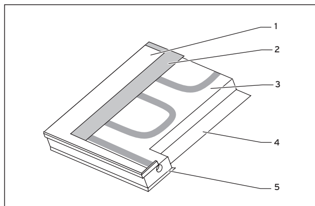
Fig. 2.6 Corte transversal del colector plano Saunier Duval HelioPLAN SRD 2.3
