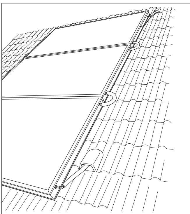
Fig. 2.5 Campo del colector de 3 HelioPLAN SRD 2.3 en montaje sobre tejado
