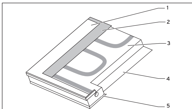
Fig. 2.6 Corte transversal del colector plano HelioPLAN SRD 2.3 de Saunier Duval
