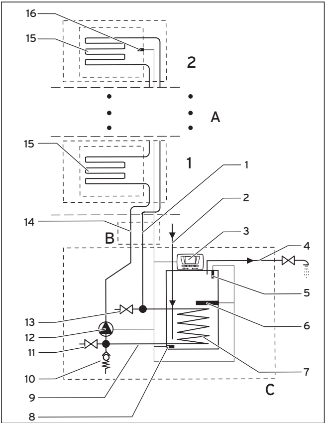
Fig. 2.3 Componentes principales del sistema HelioSet con acumulador S-FE 150 SE (esbozo básico sin accesorios de conexión)
