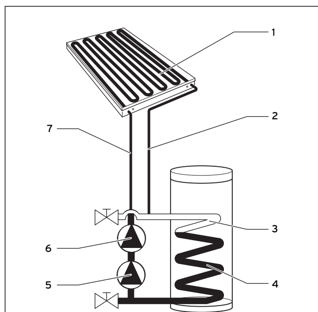
Fig. 2.2 Reparto del líquido solar durante el periodo de actividad de la/s bomba/s del colector
