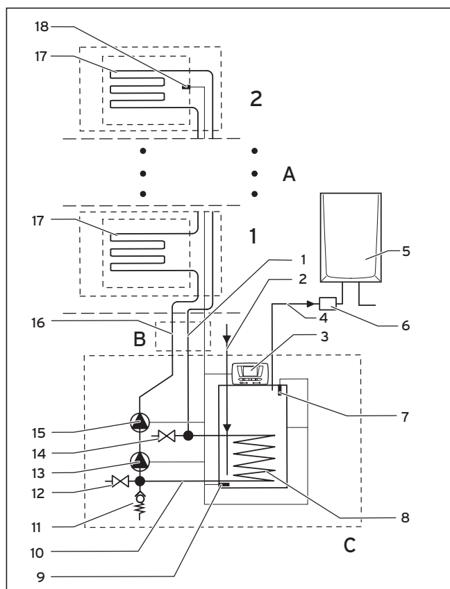
Fig. 2.4 Componentes principales del sistema HelioSet con acumulador S-FE 150/3 S P (esbozo básico sin accesorios de ventilación)
