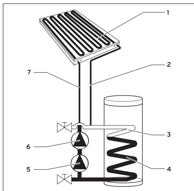
Fig. 2.3 Reparto del líquido solar con bomba del colector en funcionamiento
