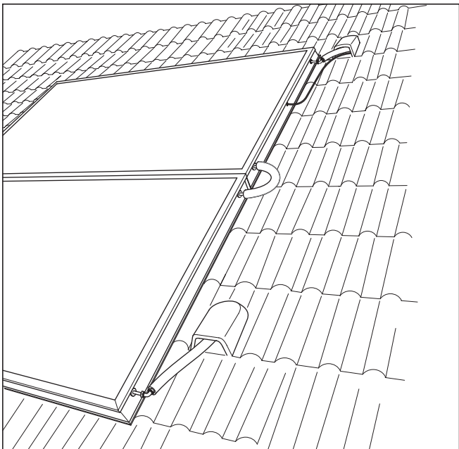
Fig. 2.5 2er Kollektorfeld HelioPLAN in Aufdachmontage
