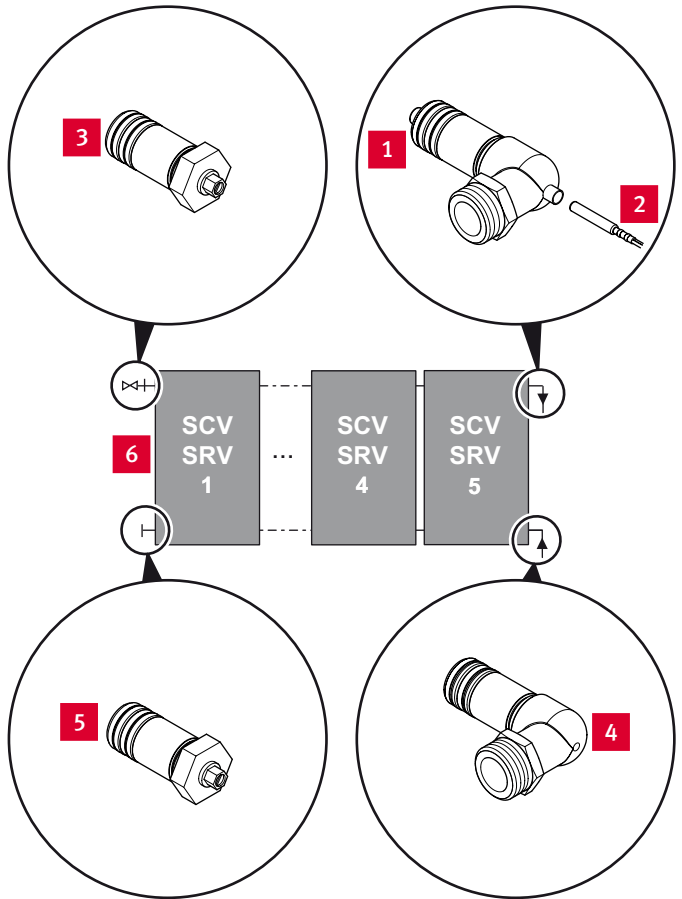
SCV - SRV conexión de entrada y salida de líquido por la derecha
