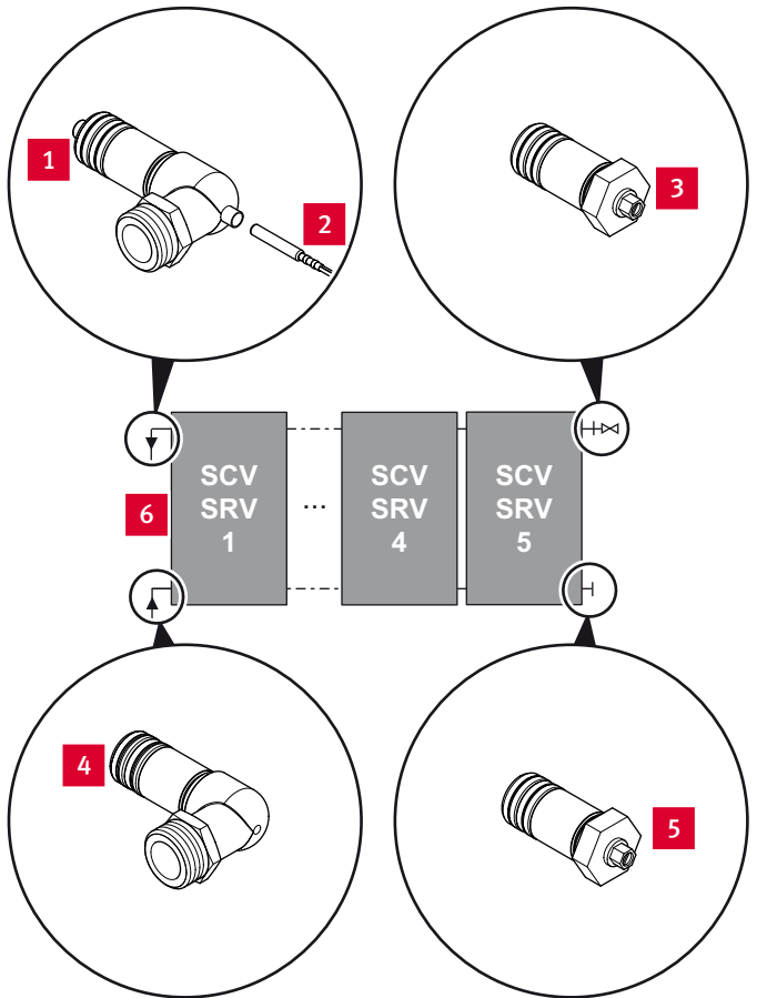
SCV - SRV conexión de entrada y salida de líquido por la izquierda
