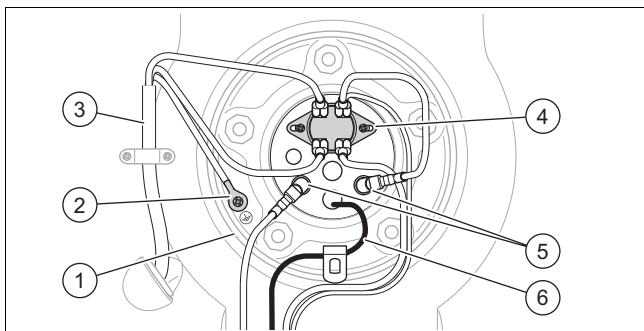
1 Brida 2 Conexión a tierra 3 Cable de alimentación eléctrica 4 Elemento de calentamiento 5 Sensor de temperatura 6 Limitador de temperatura de seguridad
