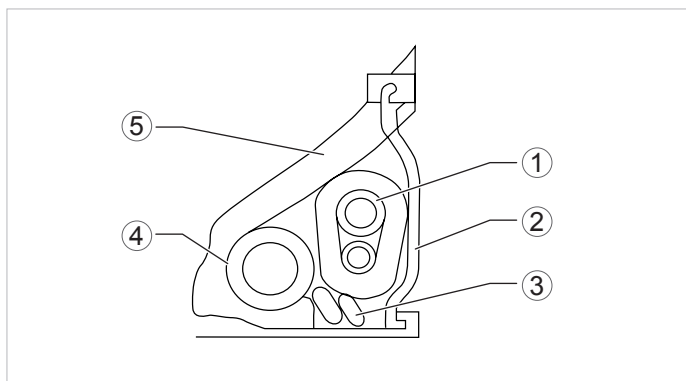
Rys. 9.11 Kładzenie rur.
