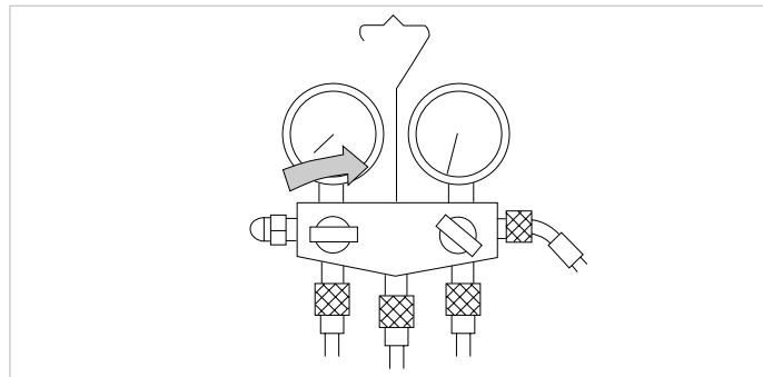
Abb. 12.4 Ablesen des Niederdruckmanometers mit geschlossenem Ventil (Dichtigkeitsprüfung) .
