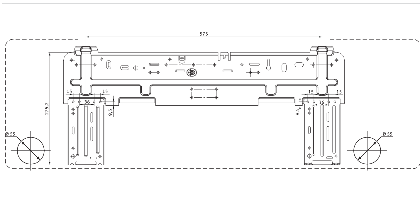
Fig. 9.8 Piastra di sostegno per l'unità 17-065 NWI.
