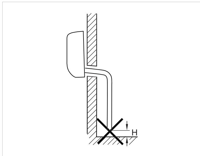
Fig. 9.4 Distanza minima dal pavimento.
