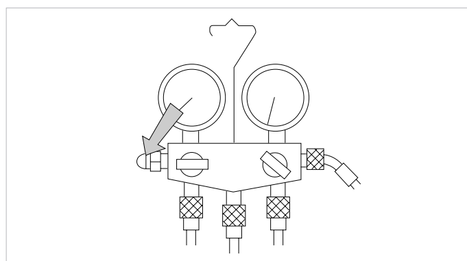
Rys. 12.3 Odczytywanie manometru niskociśnieniowego z otwartym dolnym zaworem.
