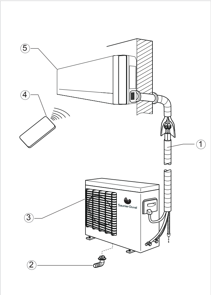
Abb. 5.1 Gerätekomponenten.
