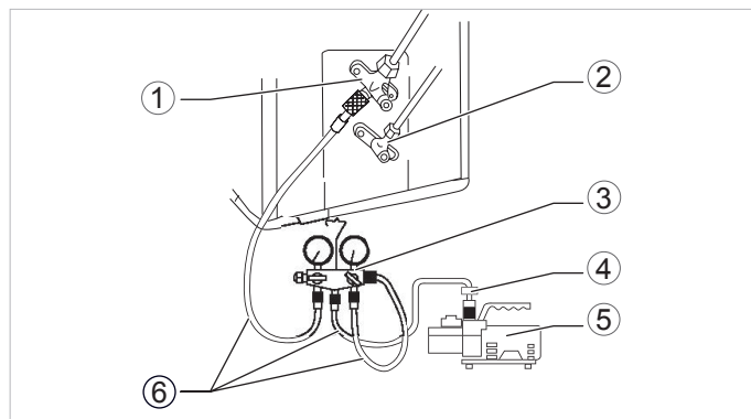
Abb. 12.2 Evakuierung der Installation
