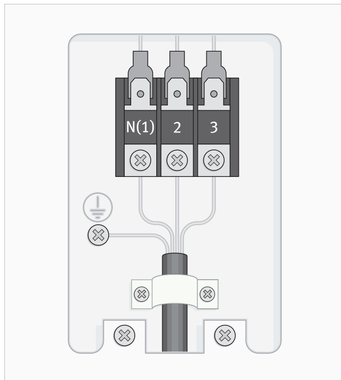
Rys. 11.2 Podłączenie zasilania elektrycznego jednostki zewnętrznej.
