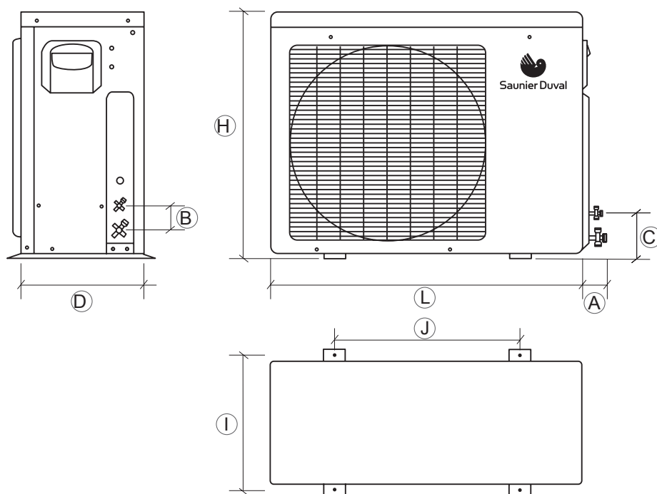
Rys. 5.3 Wymiary jednostki zewnętrznej.
