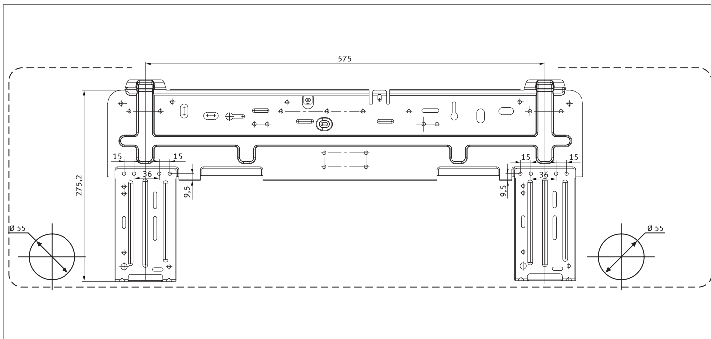
Rys. 9.8 Płyta montażowa dla modelu 17-065 NWI.
