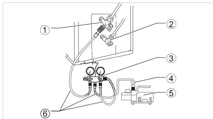
Fig. 12.2 Spurgo dell'impianto.
