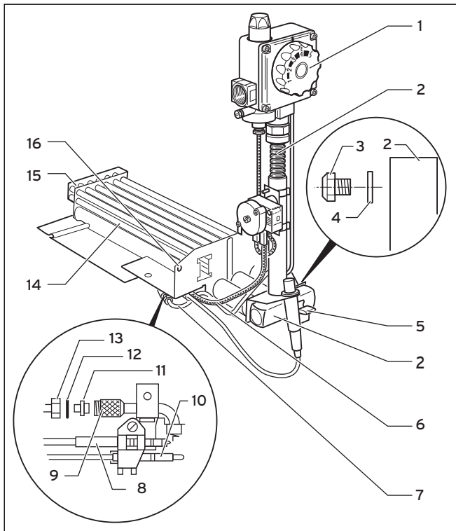
7.3 Desmontar el quemador y el mechero piloto, cambiar las boquillas del quemador y del mechero piloto
