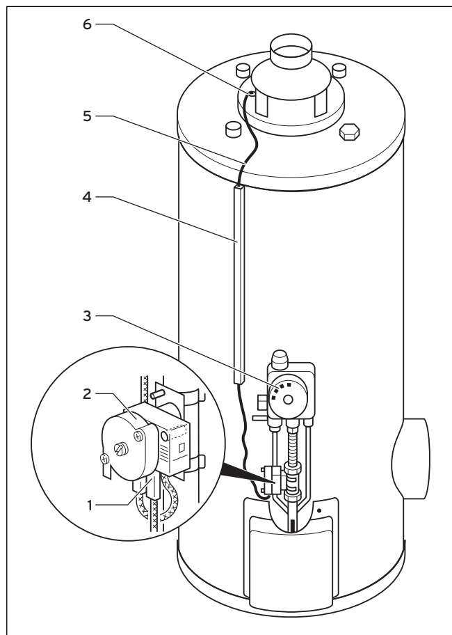
5.6 Montar el sensor de salida de gases
