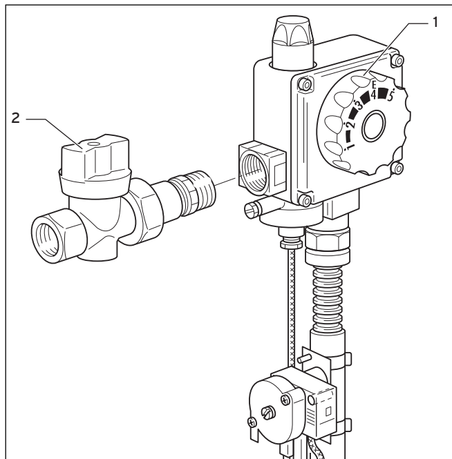
5.2 Establecer la conexión de gas
