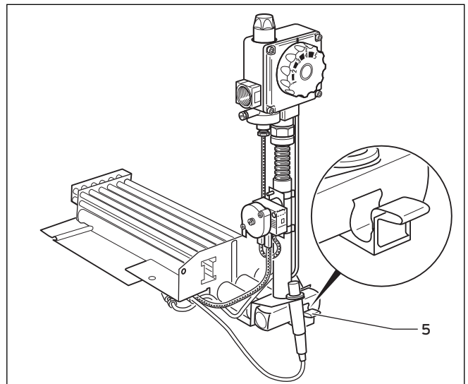
7.4 Montar la pinza en la tubería de distribución de gas correctamente
