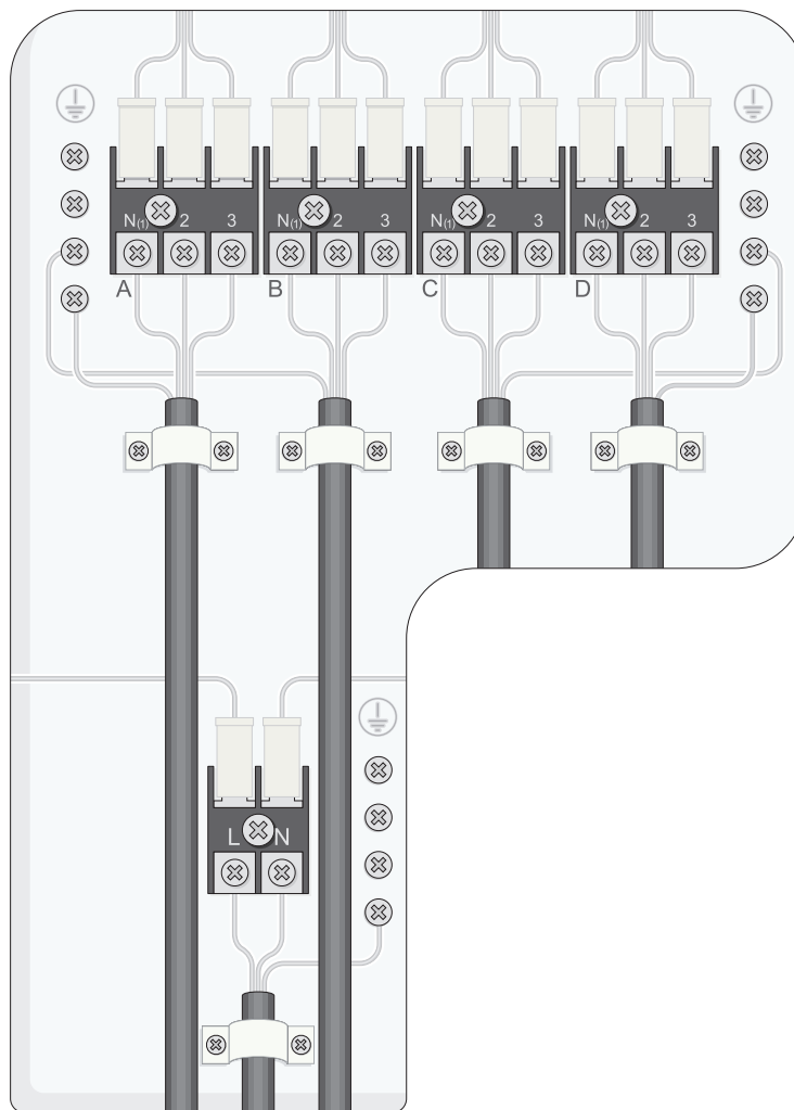
Fig. 11.2 Conexión eléctrica de la unidad exterior.
