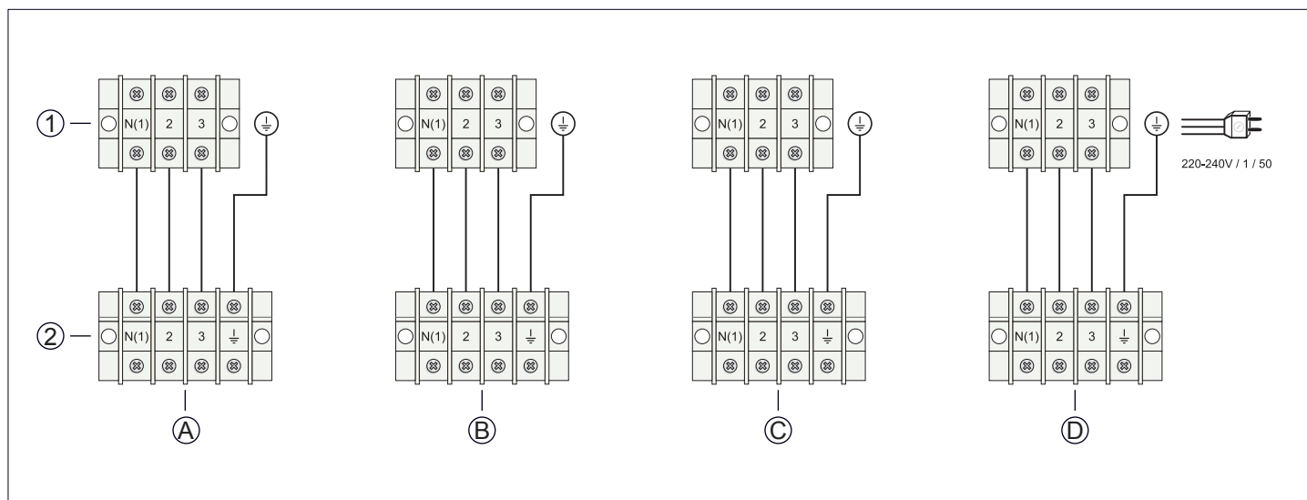
Fig. 11.3 Esquema eléctrico de interconexión entre la unidad exterior e interior.
