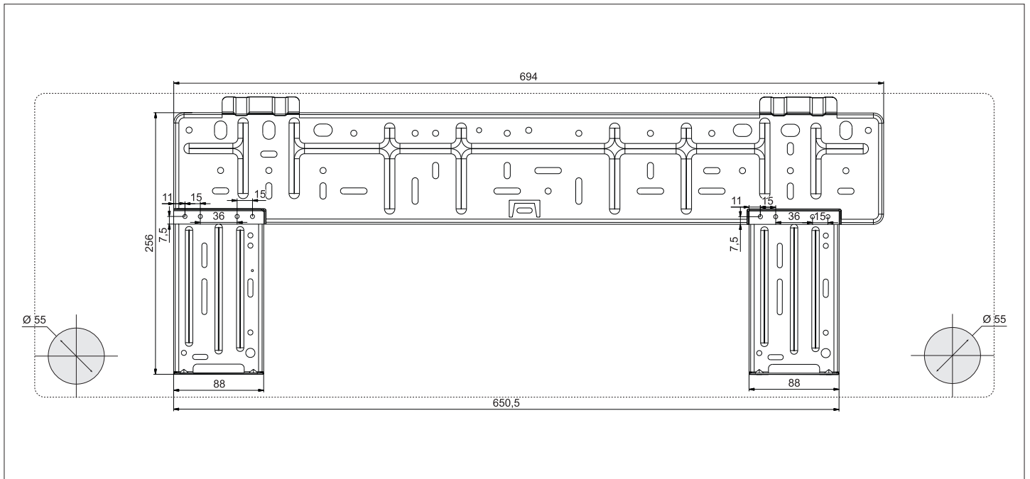
Fig. 9.8 Placa de montaje para 17-050 NMWI.
