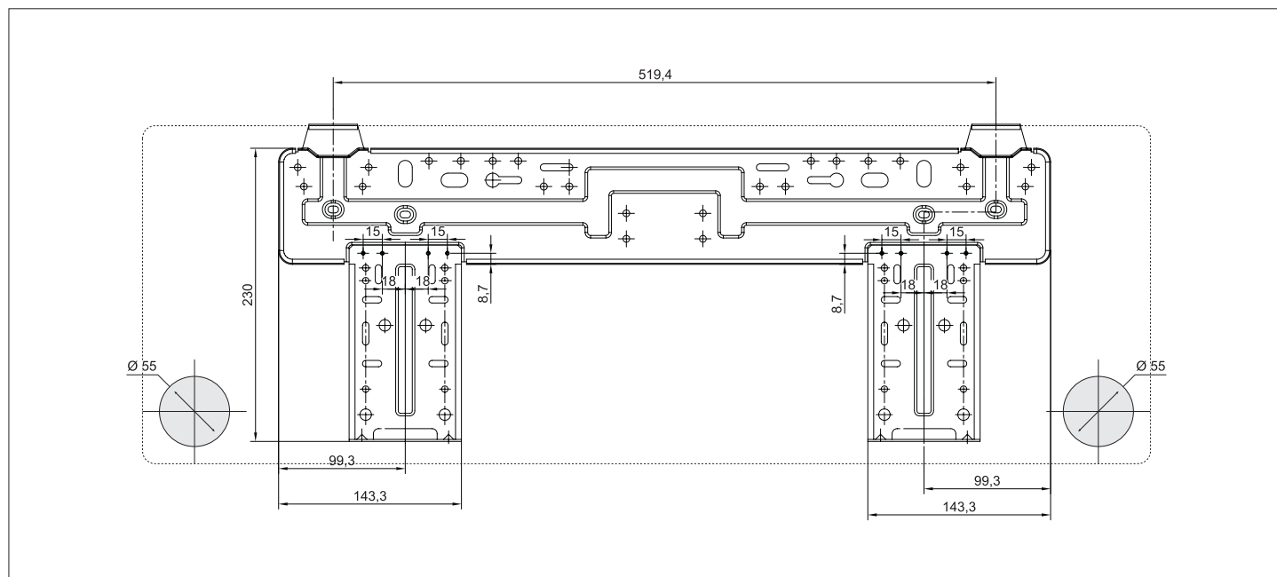
Fig. 9.6 Placa de montaje para 17-025 NMWI.
