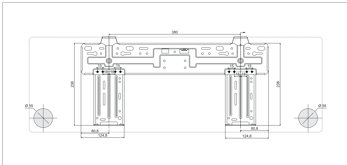
Fig. 9.7 Placa de montaje para 17-035 NMWI.
