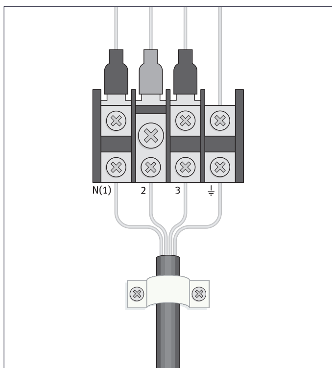
Fig. 11.1 Conexión eléctrica de la unidad interior.
