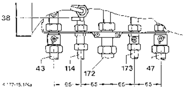
Figura 6 Montaje - plantilla de conexión, terminada
