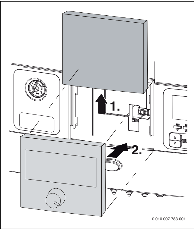
Fig. 29 Retirar la cubierta y montar el controlador
