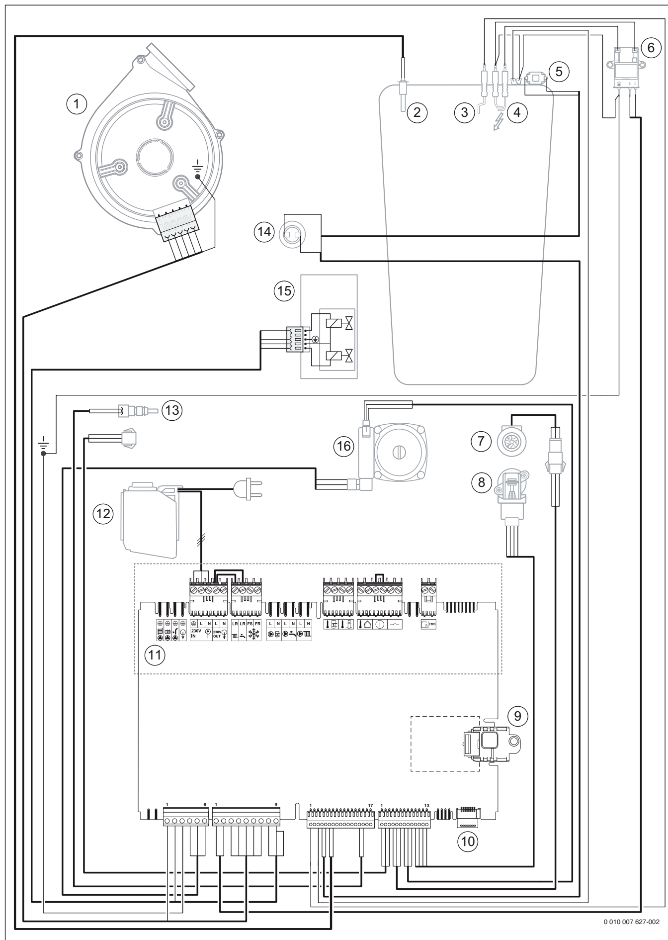
Fig. 72 Cableado eléctrico
