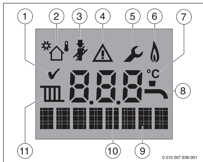
Fig. 35 Indicaciones del display
