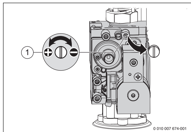
Fig. 40 Retirar el precinto
