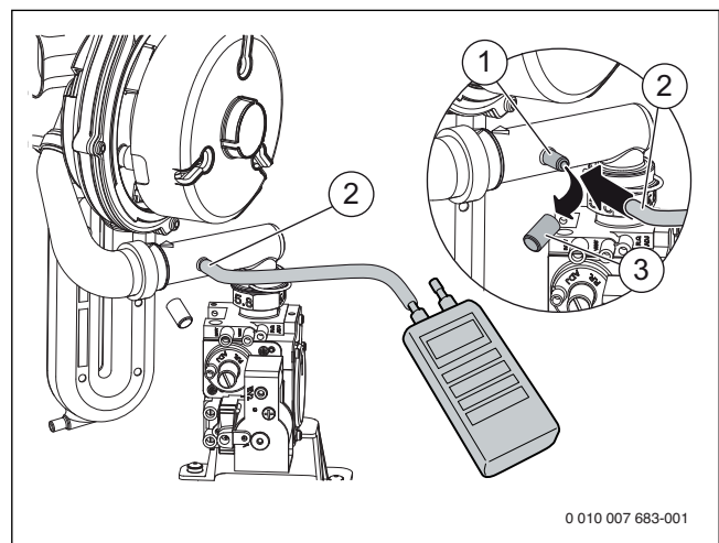
Fig. 47 Boquilla de medición para la presión del ventilador
