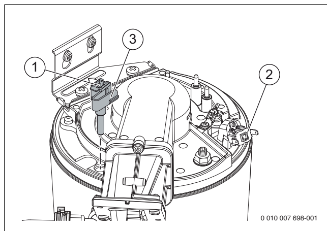
Fig. 50 Desmontar la sonda de la temperatura de impulsión
