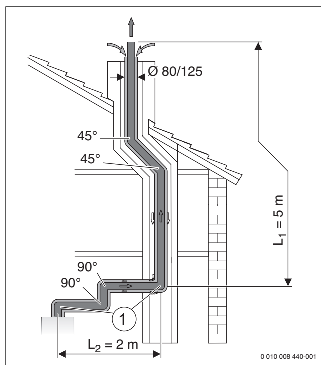
Fig. 16 Situación de montaje de una evacuación de gases según C 33
