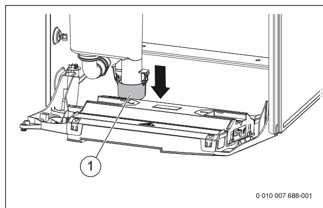
Fig. 59 Retirar la tapa del sifón de condensado
