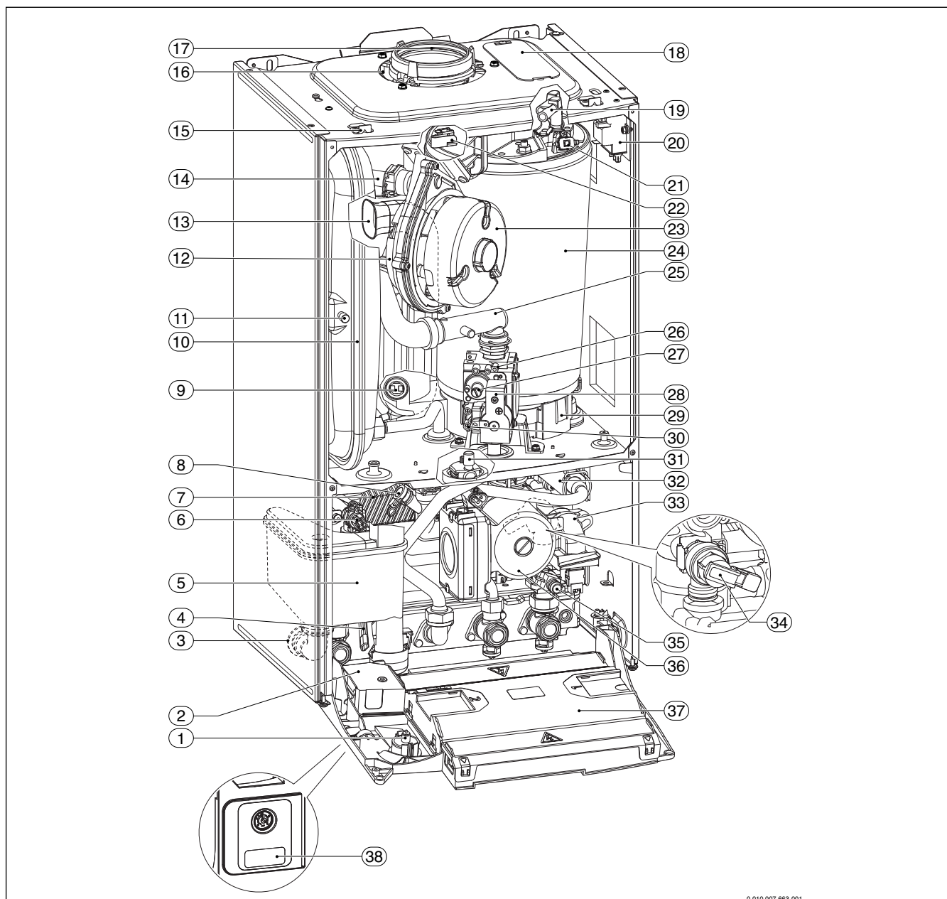
Fig. 3 Visión general del producto
