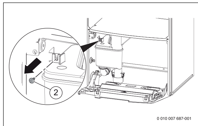
Fig. 60 Soltar el tornillo en el sifón de condensado
