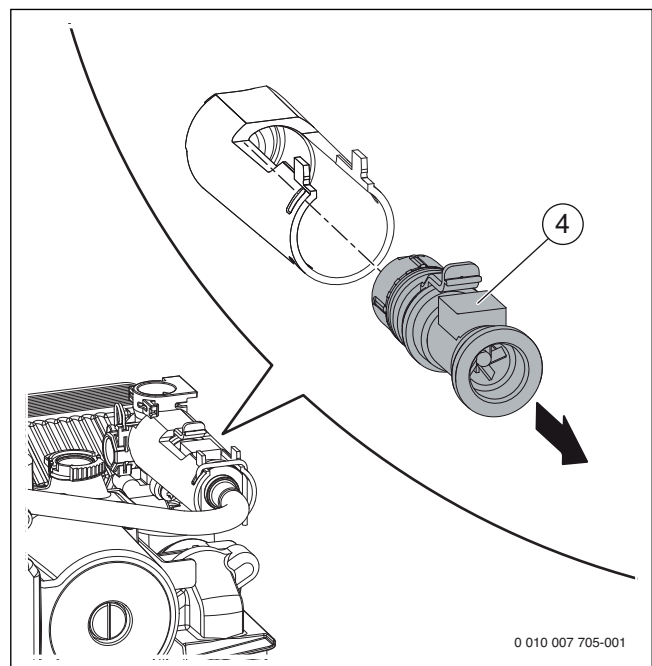
Fig. 64 Desmontar la turbina de la carcasa
