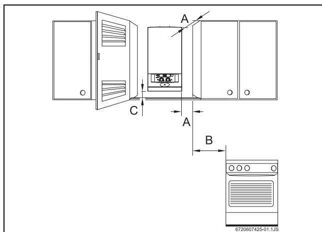
Fig. 6 Separaciones mínimas
