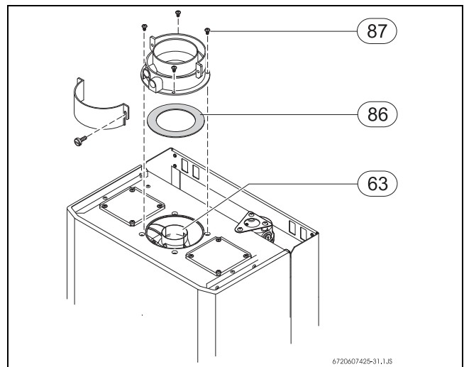
Fig. 13 Montaje del anillo de estrangulación
