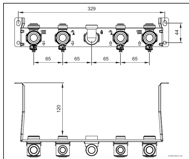
Fig. 8 Conexiones hidráulicas
