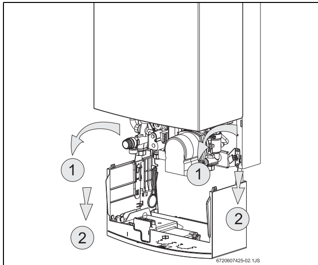
Fig. 30 Posición de servicio para acceso a la parte hidráulica y eléctrica
