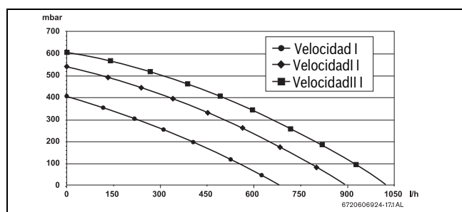
Fig. 5 Curva característica da bomba
