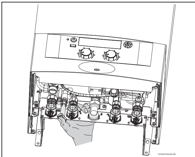
Fig. 14 Llave de llenado
