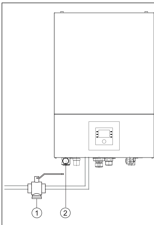
Fig. 6 Unidad interior ACB
