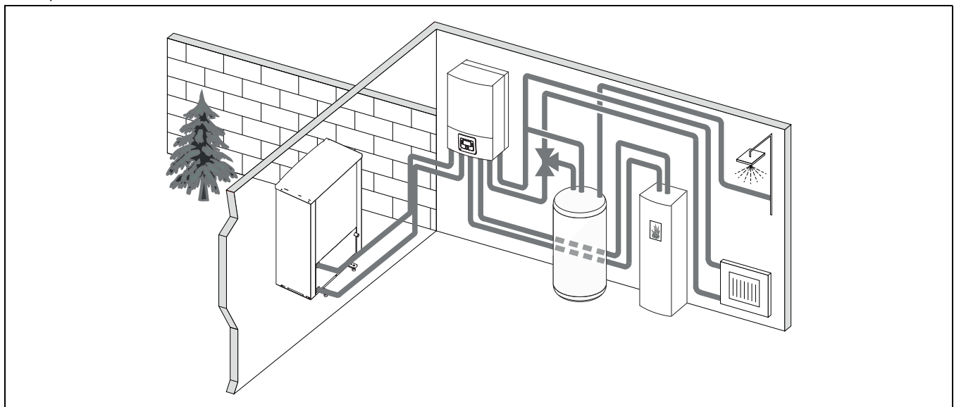
Fig. 3 Bomba de calor Supraeco Hydro SAO-2, unidad interior ACB sin calefacción eléctrica, acumulador externo de agua caliente y calefacción eléctrica externa
