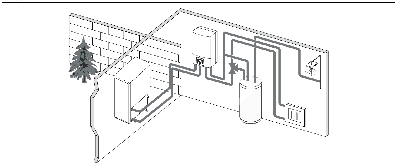
Fig. 3 Bomba de calor Supraeco Hydro SAO-2, unidad interior ACE con calefacción eléctrica y acumulador de agua caliente
