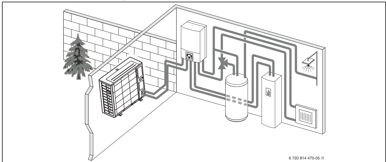
Fig. 2 Bomba de calor unidad exterior, unidad interior ASB sin calefacción eléctrica, acumulador externo de agua caliente y calefacción eléctrica externa
