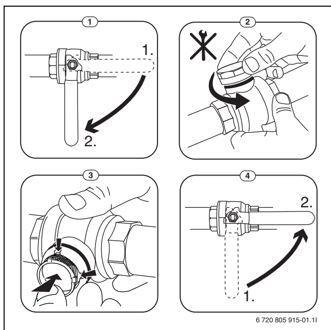
Fig. 6 Limpieza de filtro
