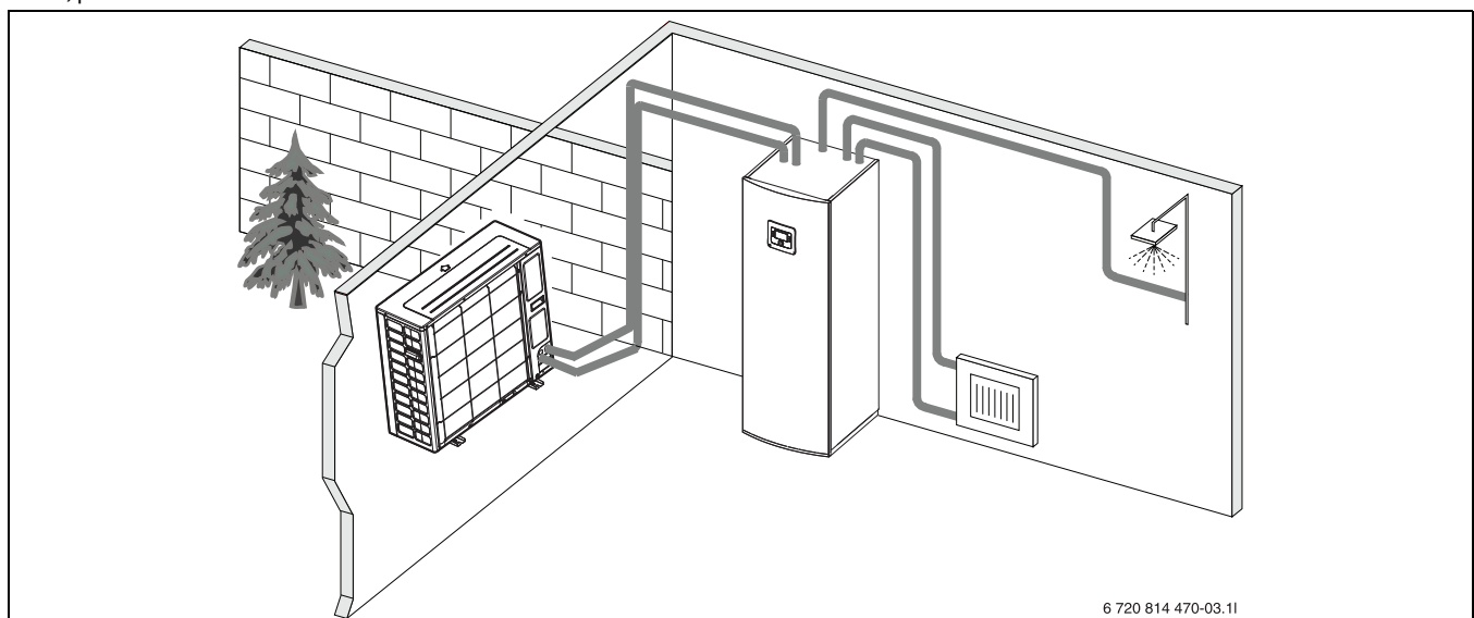
Fig. 2 Bomba de calor unidad exterior, unidad interior ASM/ASMS con acumulador de agua caliente integrado y calefacción eléctrica
