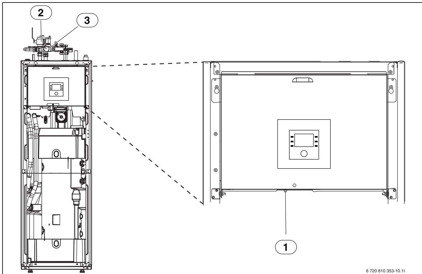
Fig. 5 Unidad interior ASM / ASMS
