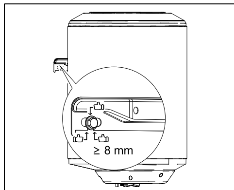
Fig. 7 Instalación en posición vertical (montaje mural)
