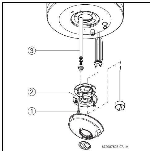
Fig. 14 Acceso a la zona interior e identificación de las partes
