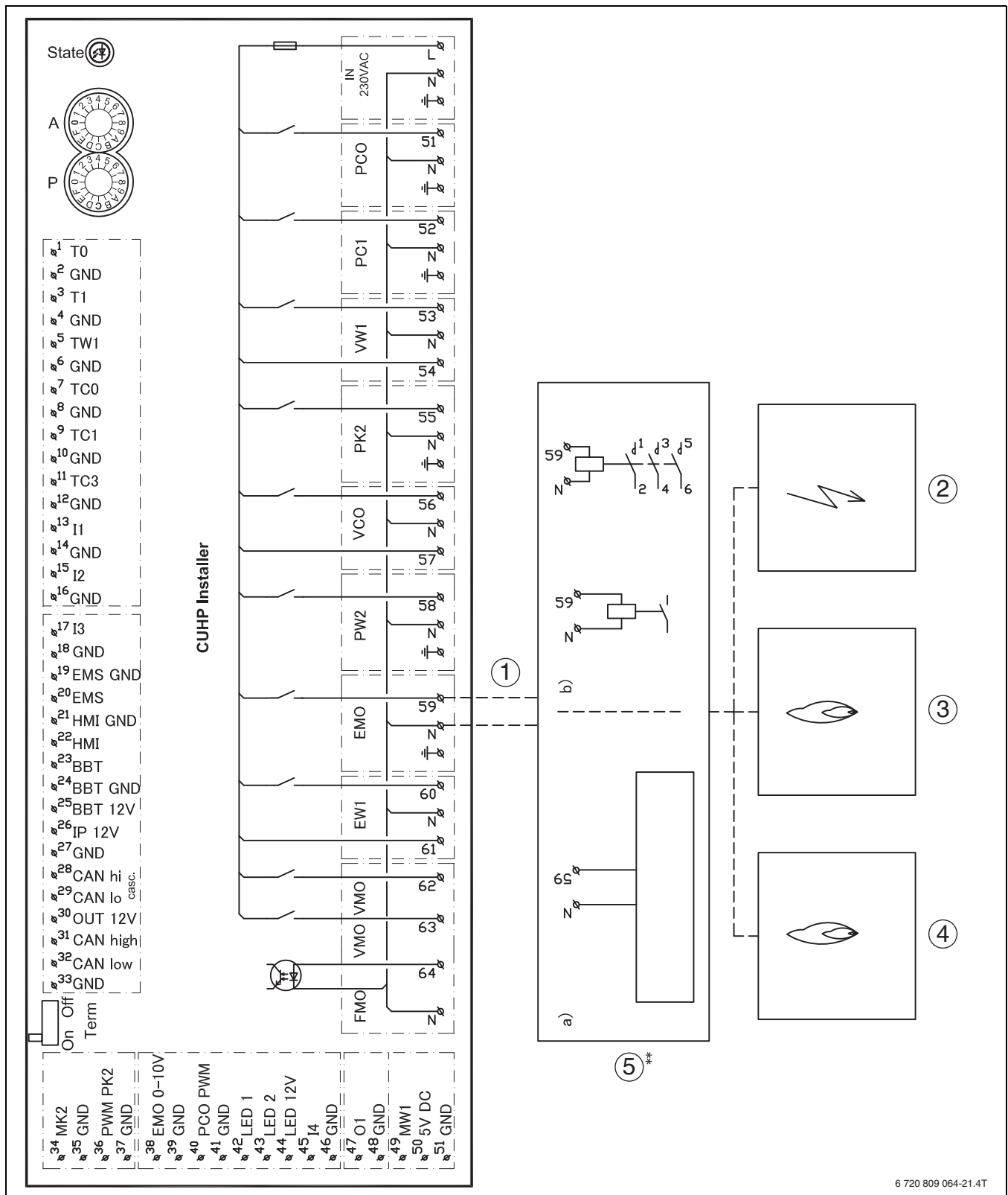
Fig. 32 Esquema de conexión para módulo de instalación, inicio/parada con calefactor externo
