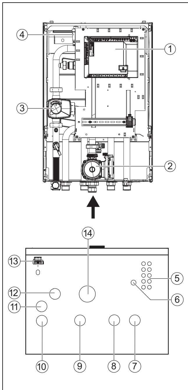
Fig. 3 Componentes y conexiones de tubo de la unidad interior con mezcladora para calefactor externo
