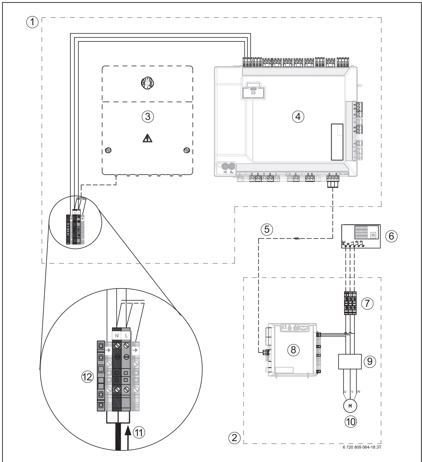
Fig. 29 Bomba de calor monofásica y unidad interior con calefactor externo
