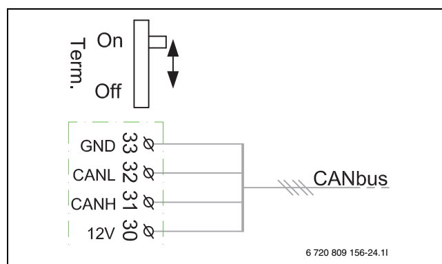
Fig. 9 Terminación CAN-BUS
