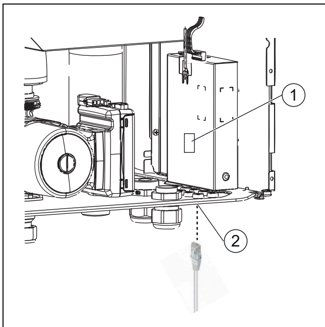
Fig. 24 Módulo IP
