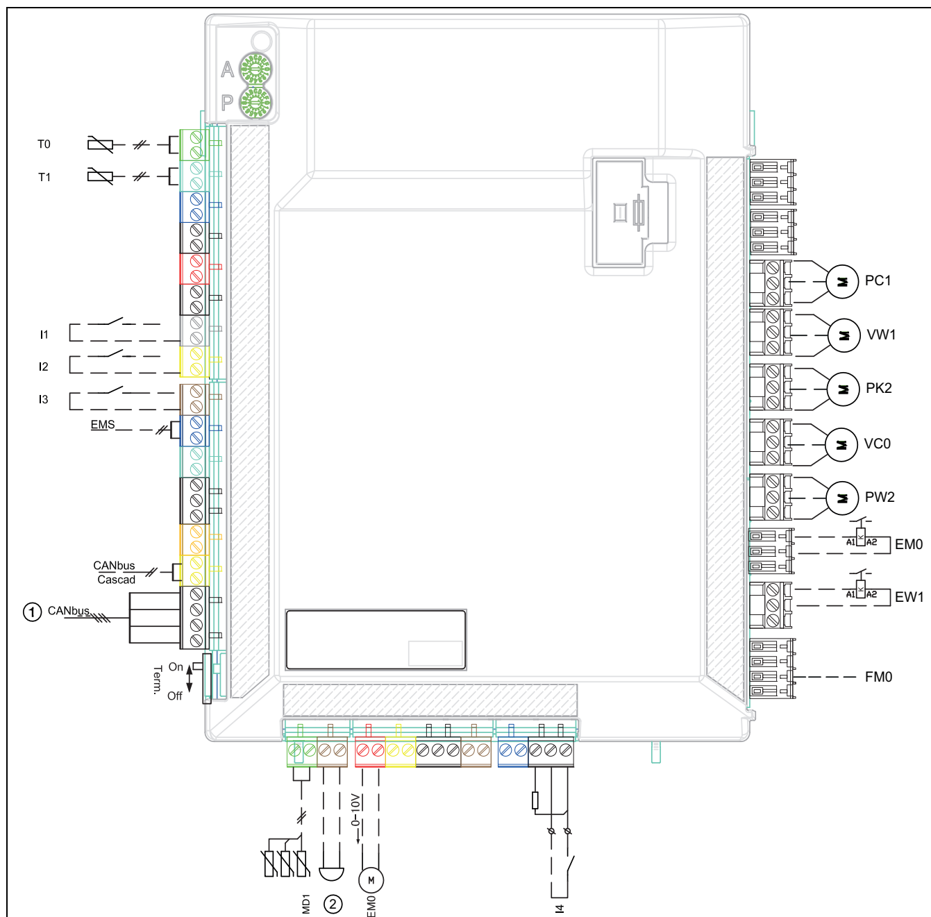
Fig. 12 Conexiones módulo de instalación
