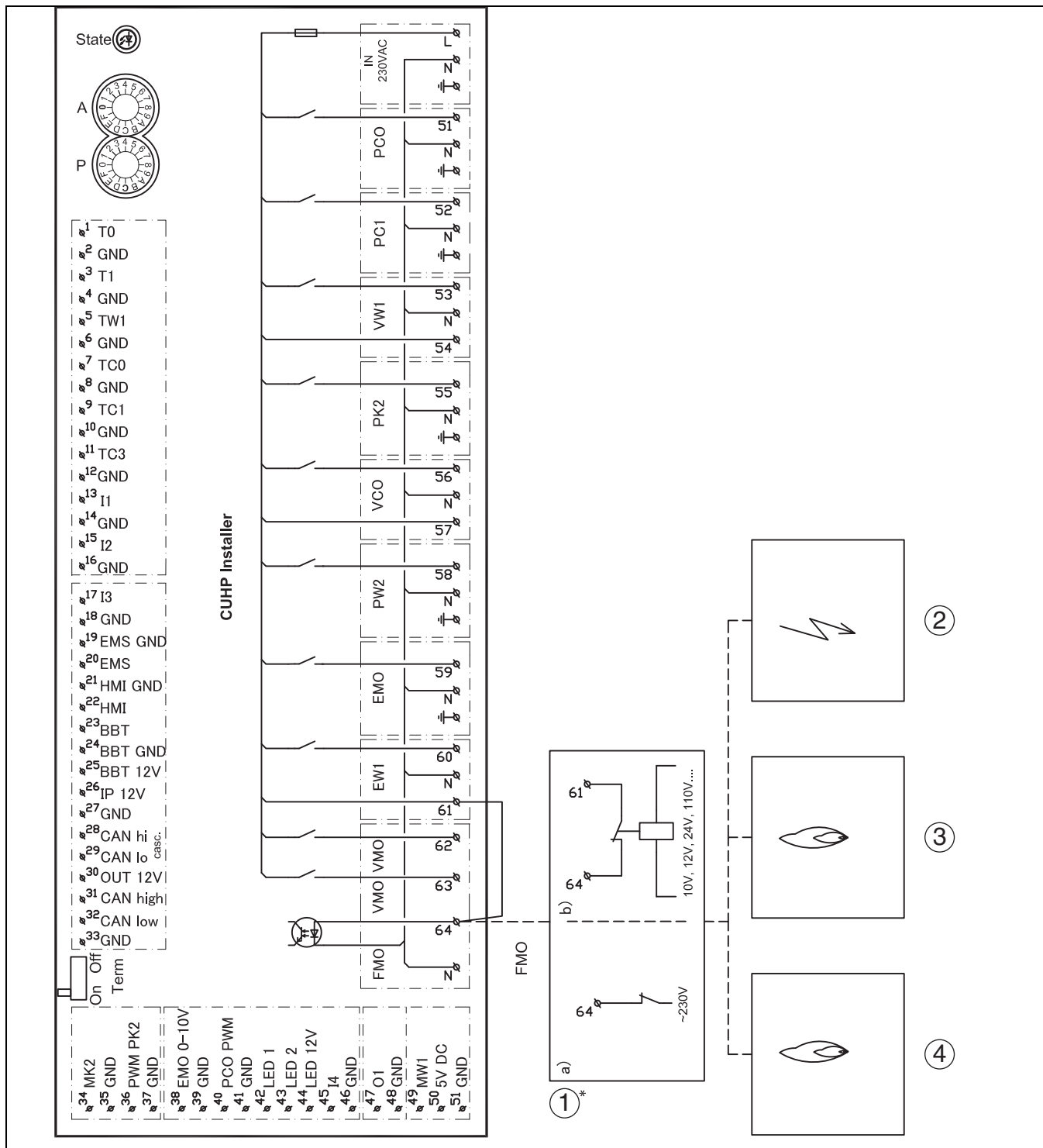
Fig. 33 Esquema de conexiones para módulo de instalación, alarma del calentador adicional externo
