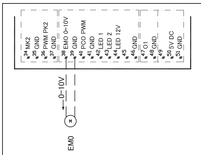
Fig. 13 Activación 0 hasta 10V para calefacción eléctrica
