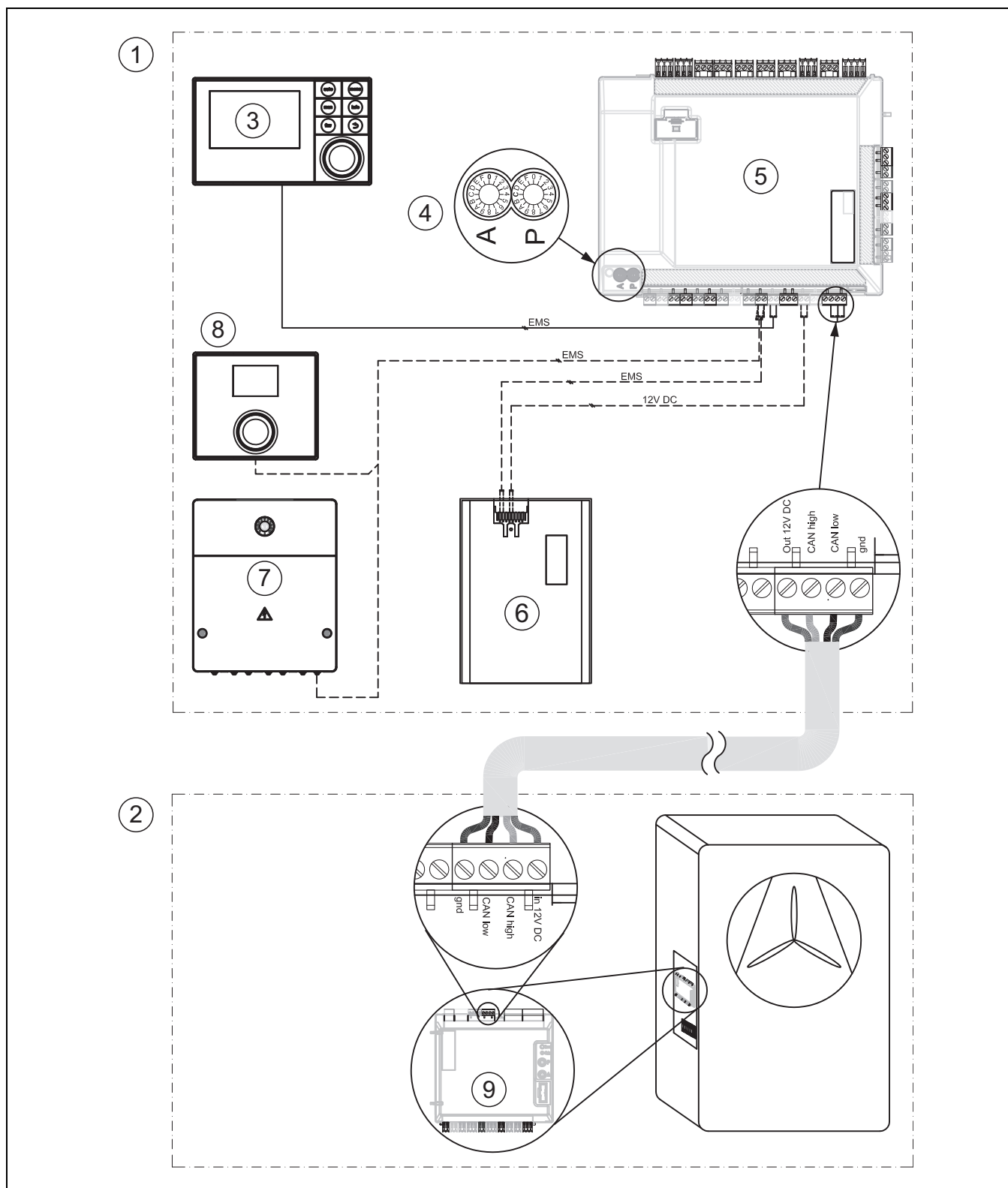
Fig. 28 Unidad interior con mezclador para calefacción eléctrica externa - vista general CAN-/EMS-BUS
