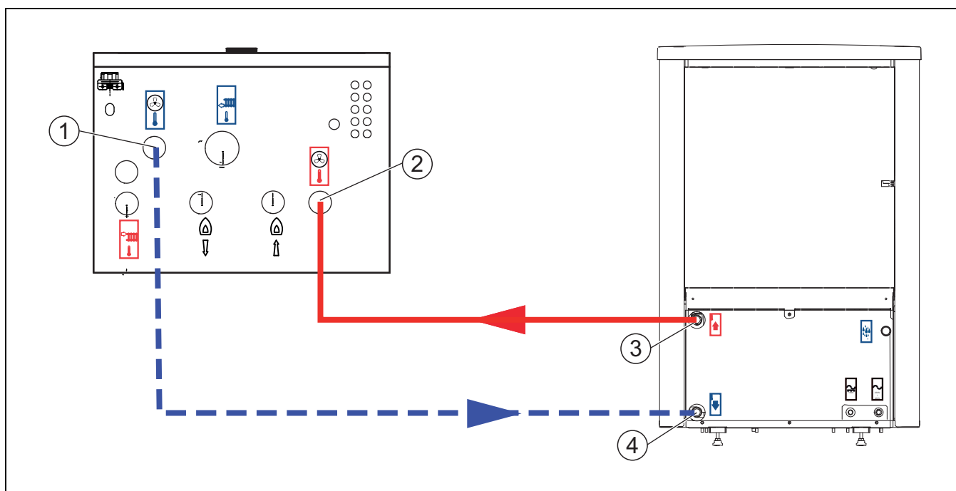
Fig. 6 Conexión de la unidad interior a la bomba de calor
