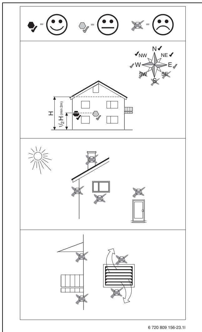
Fig. 10 Ubicación de la sonda de temperatura exterior
