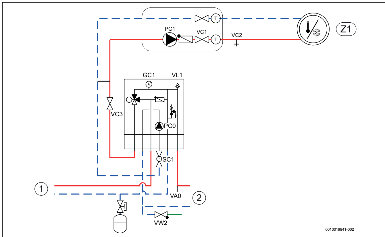
Fig. 8 Unidad interior con calefacción externa y sistema de calefacción
