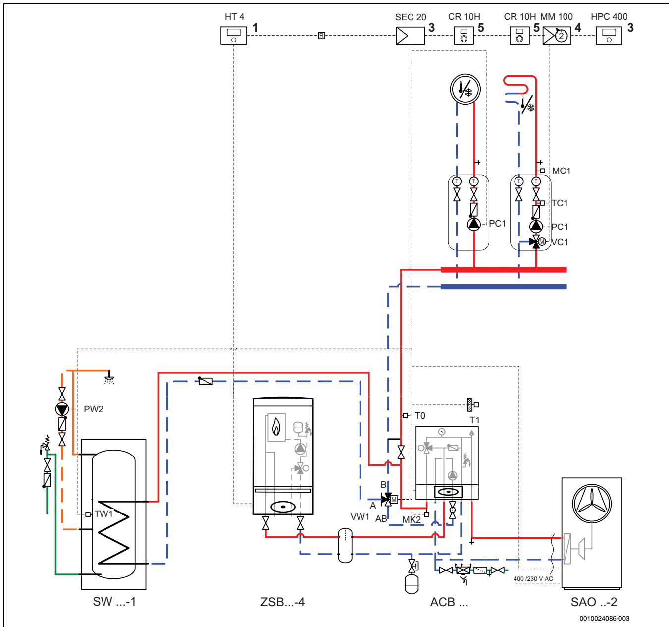
Fig. 27 Calefactor con mezclador con acumulador de agua caliente
