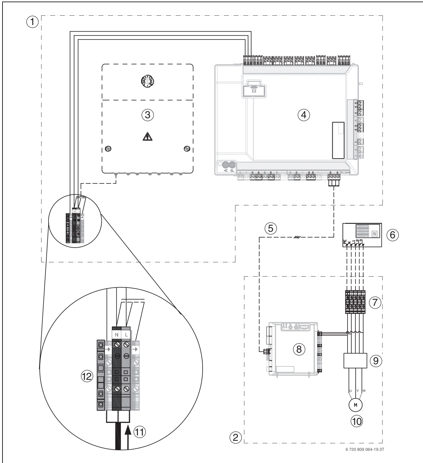
Fig. 30 Bomba de calor trifásica y unidad interior con calefactor externo
