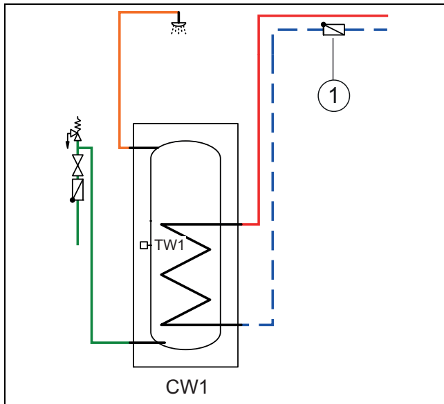
Fig. 18 Acumulador de agua caliente
