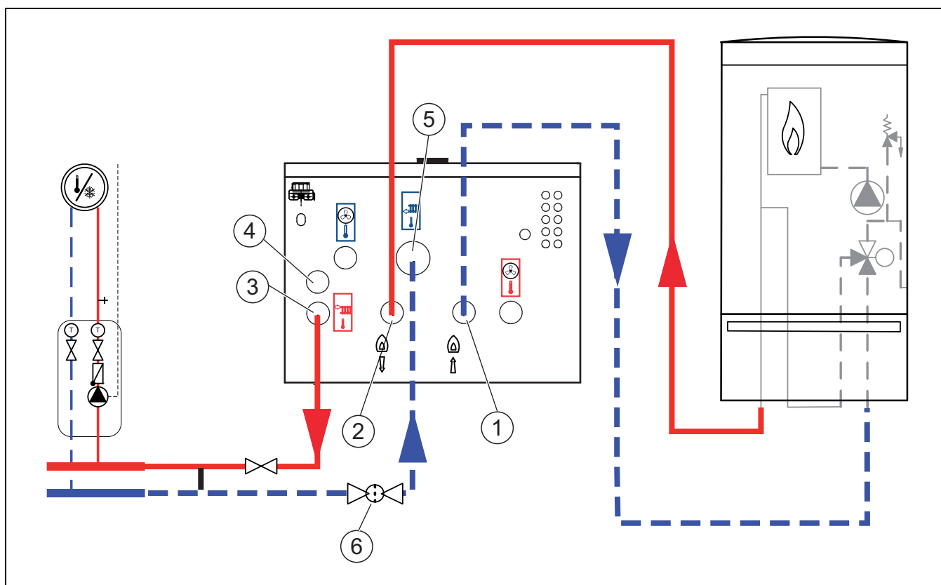
Fig. 7 Conexión de la unidad interior con mezclador para calefacción eléctrica a la instalación de calefacción y a la calefacción eléctrica
