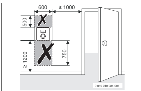
Fig. 5 Lugar de instalación de la unidad de mando
