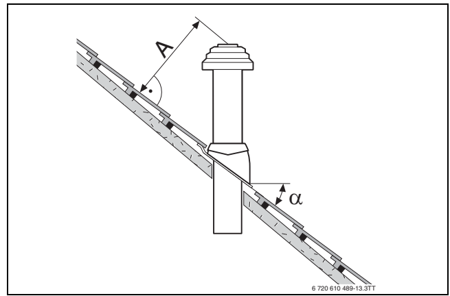
Fig. 7 Distancias e inclinaciones de tejados inclinados
