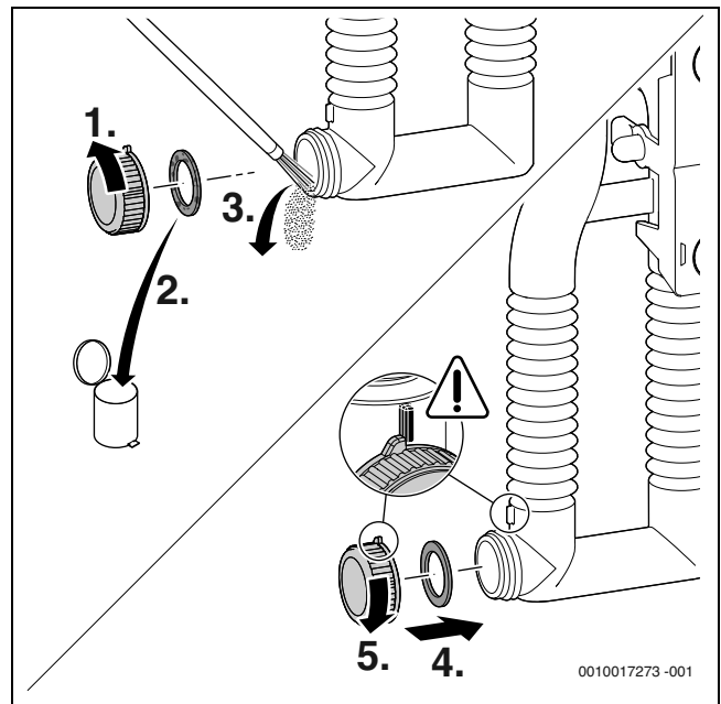
Fig. 53 Limpiar el sifón de condensado
