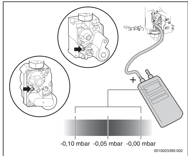
Fig. 37 Inspección de la presión diferencial
