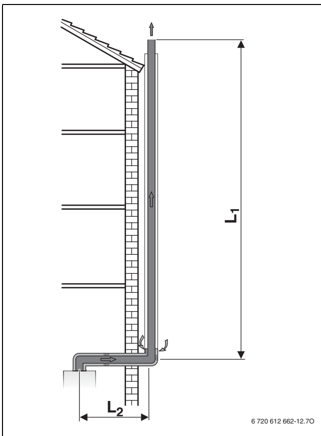
Fig. 17 Evacuación de gases en la fachada según C 53
