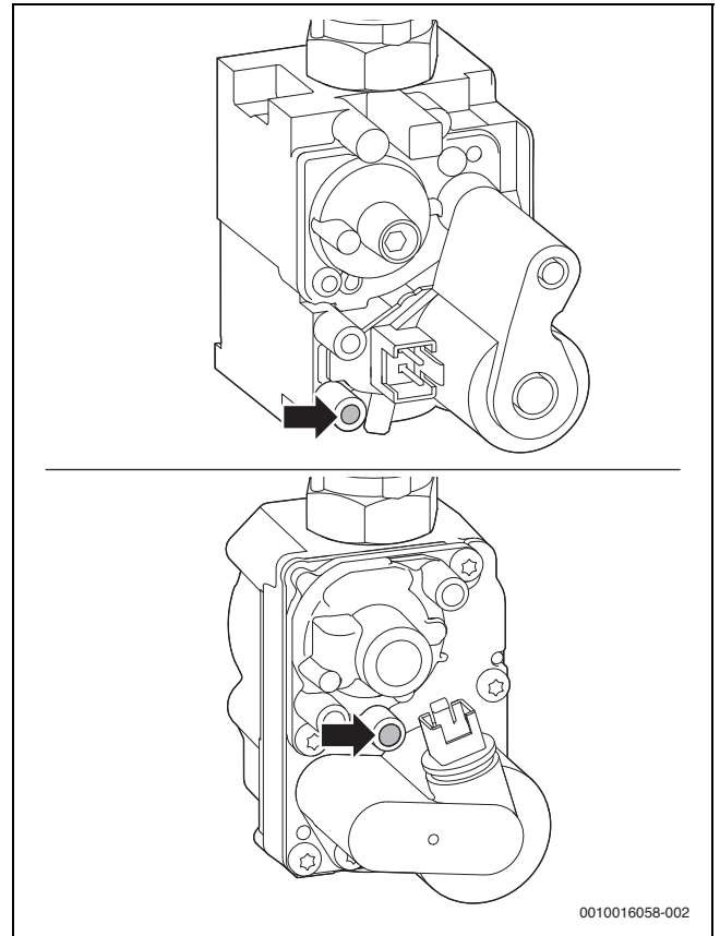
Fig. 40 Boquilla de medición para presión de conexión del gas
