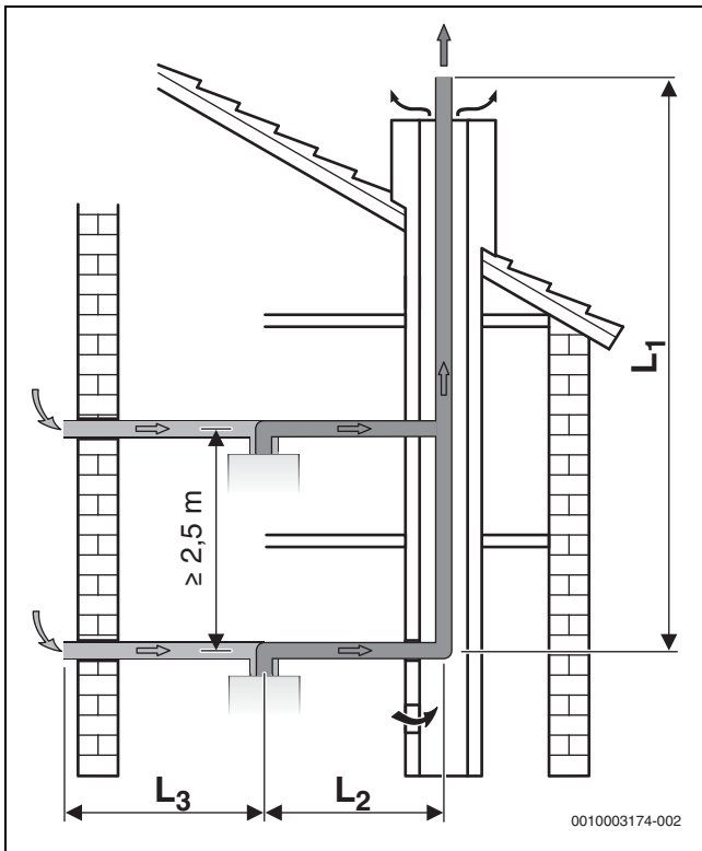
Fig. 20 Conexión múltiple con tubo de entrada de aire según C 83
