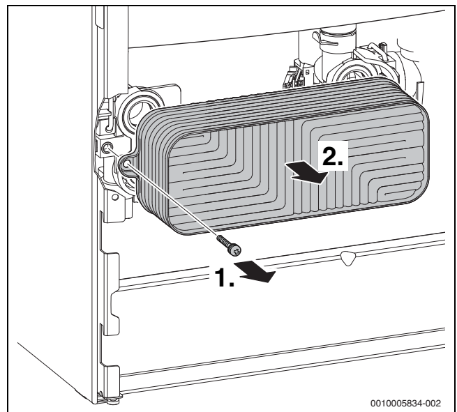
Fig. 60 Desmontar el intercambiador de placas
