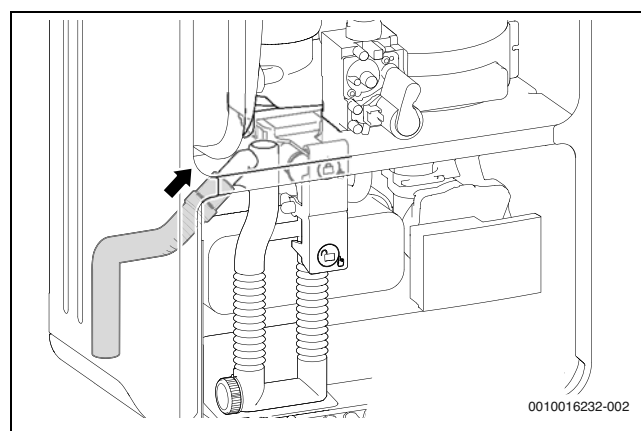
Fig. 26 Montar la manguera en el sifón de condensado
