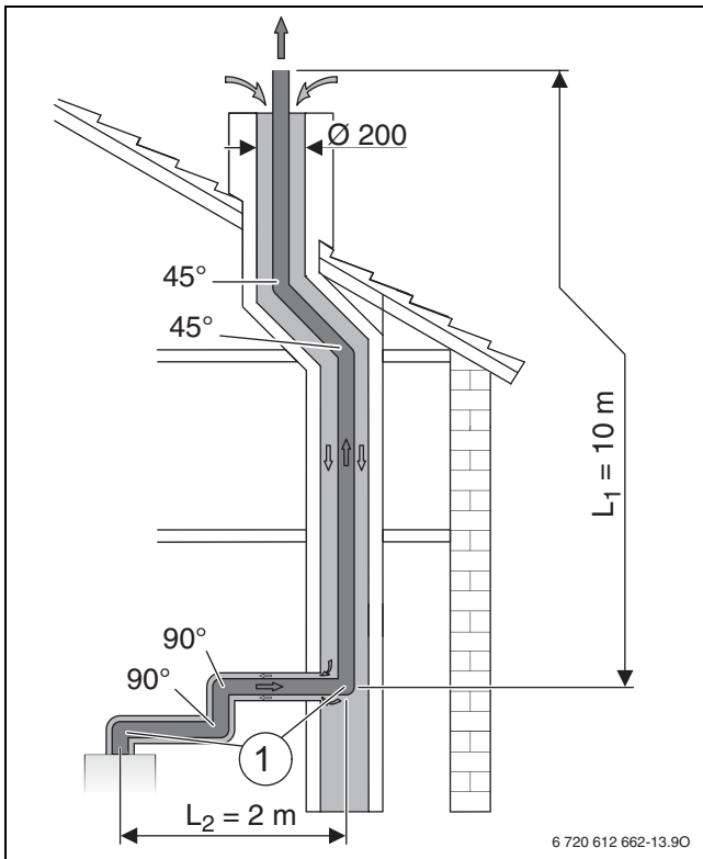
Fig. 18 Situación de montaje de una evacuación de gases en la chimenea según C 93
