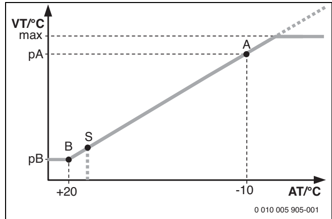
Fig. 74 Curva de calefacción
