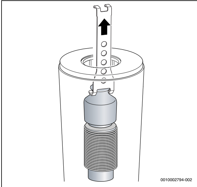
Fig. 47 Extraer los cuerpos expulsores superiores
