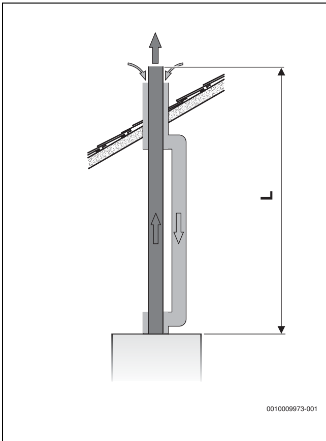
Fig. 16 Evacuación de gases vertical según C 33
