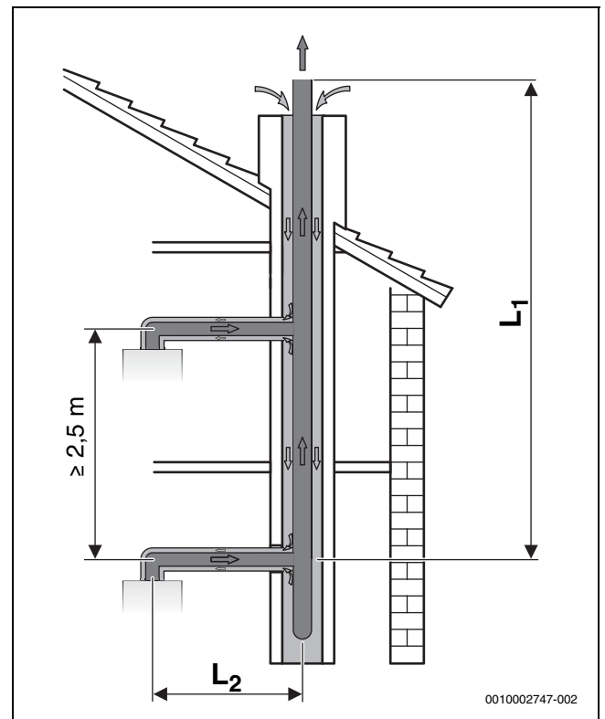
Fig. 19 Conexión múltiple con tubo concéntrico según C 43
