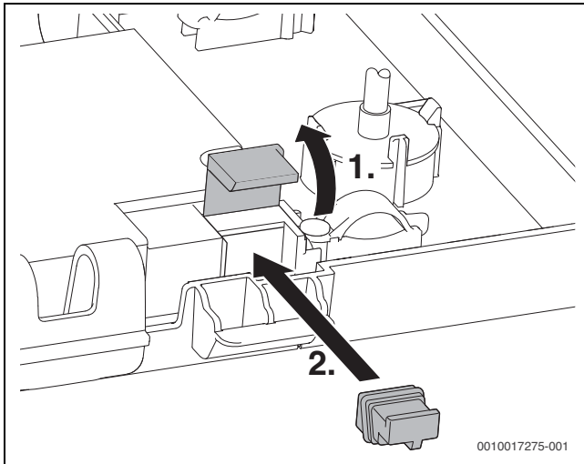
Fig. 69 Colocar el conector codificado
