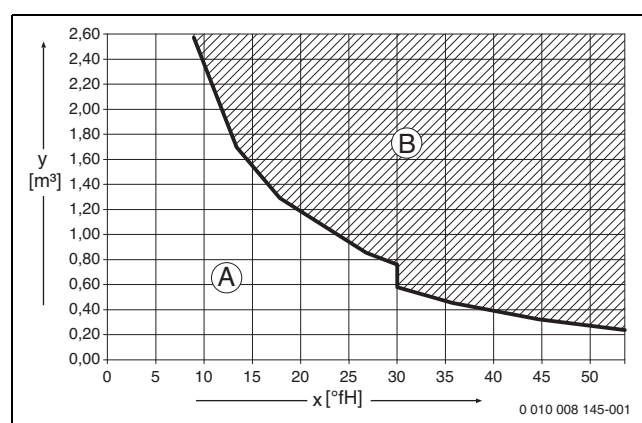
Fig. 22 Requisitos en aparatos < 50 kW de agua de llenado y rellenado en °fH
