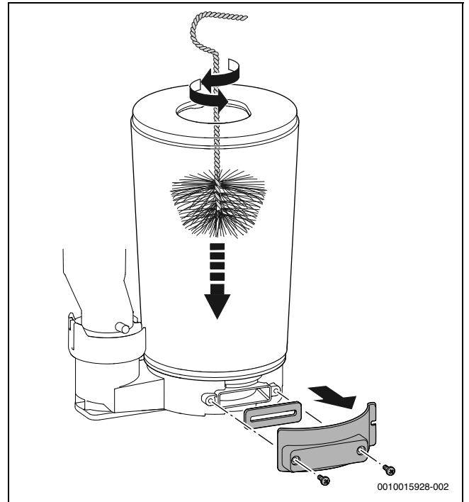
Fig. 49 Limpiar el bloque térmico
