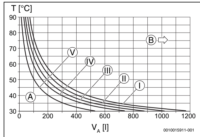
Fig. 23 Líneas características del vaso de expansión
