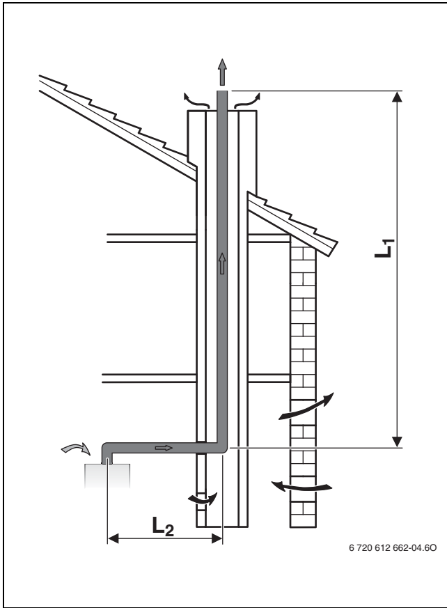
Fig. 8 Evacuación de gases en chimenea según B 23p
