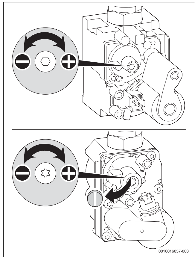
Fig. 38 Retirar el precinto en el tornillo de ajuste
