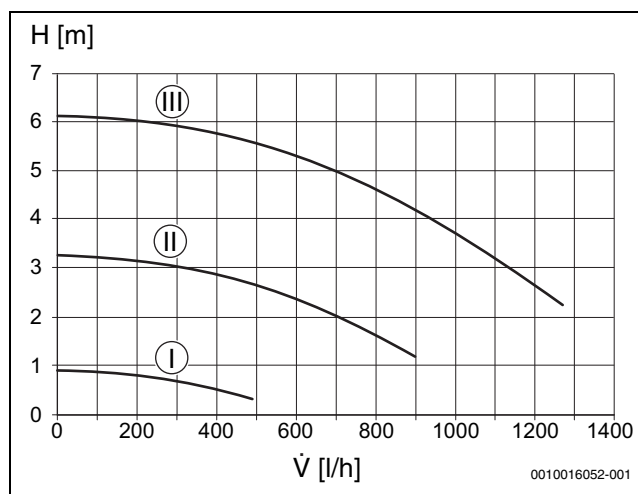
Fig. 34 Curva característica de la bomba de circulación (número constante de revoluciones)
