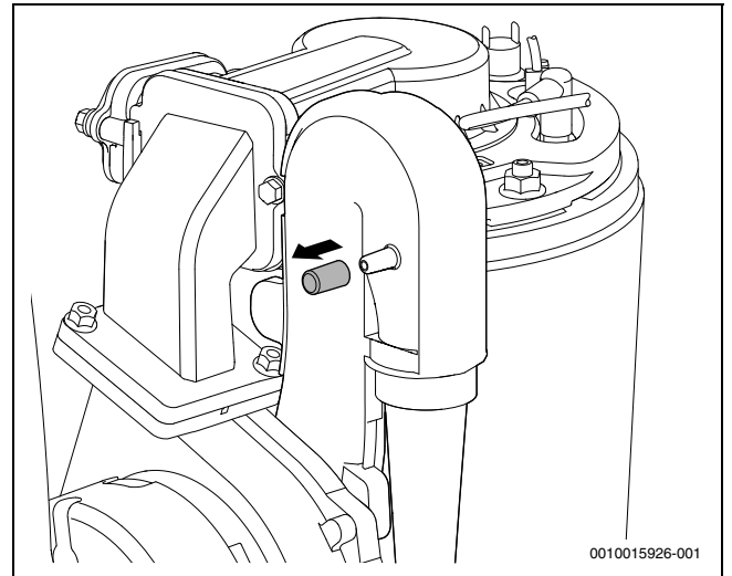
Fig. 42 Boquilla de medición en el dispositivo mezclador
