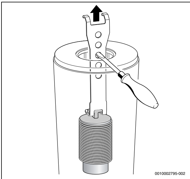
Fig. 48 Extraer los cuerpos expulsores inferiores
