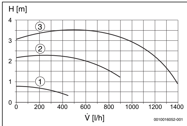
Fig. 36 Curva característica de la bomba de calefacción (presión proporcional)
