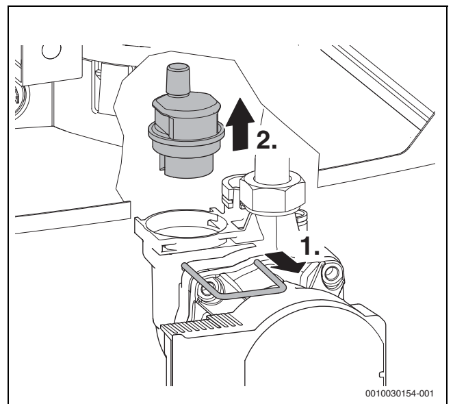
Fig. 64 Desmontar el purgador automático
