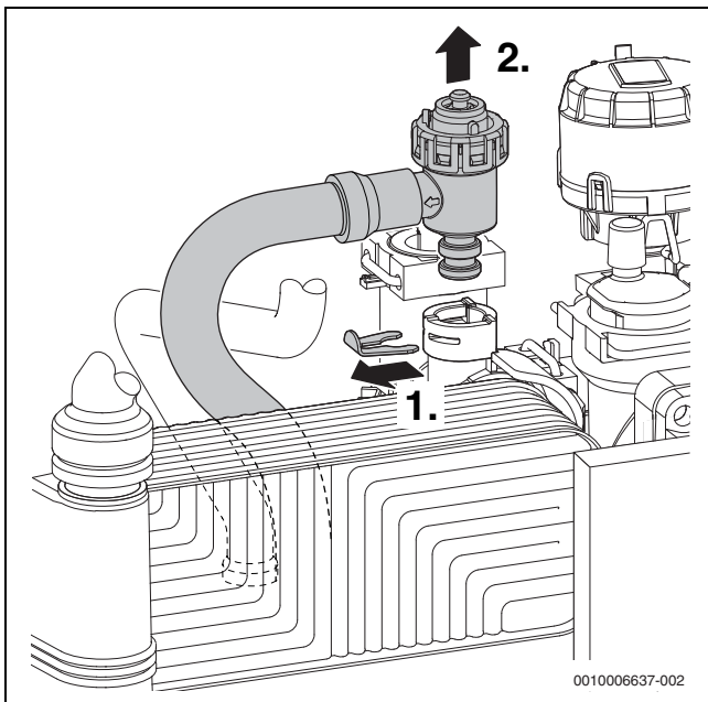
Fig. 58 Retirar la válvula de seguridad (circuito de calefacción)
