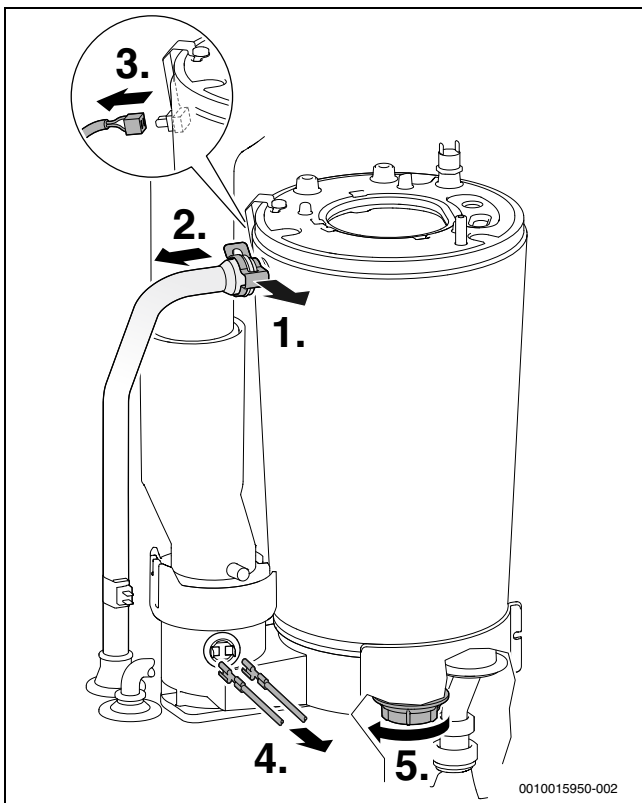
Fig. 66 Soltar el tubo de impulsión y el cable
