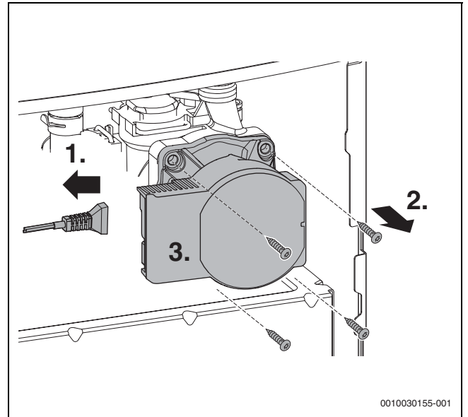
Fig. 63 Desmontar la bomba de agua caliente
