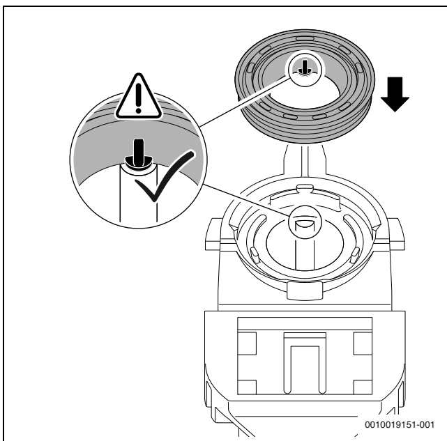
Fig. 55 Ajustar la nueva junta según el sifón de condensados
