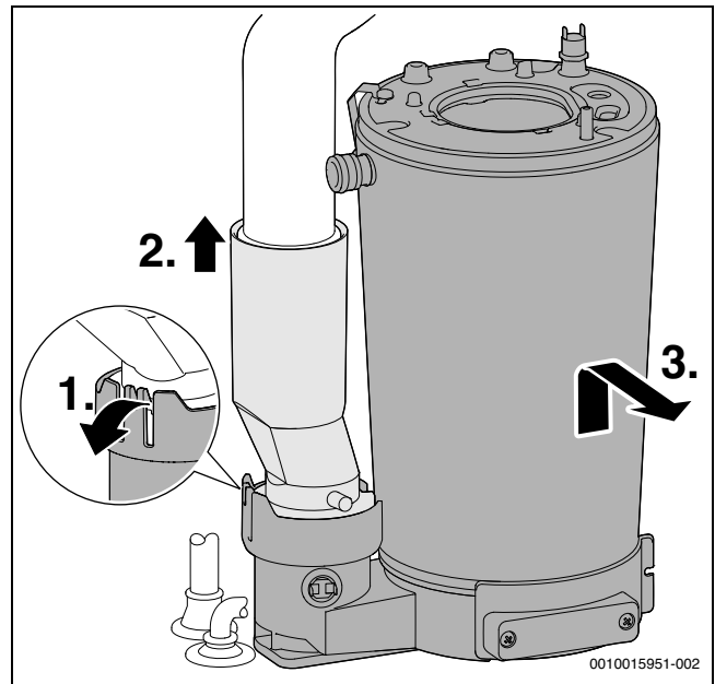
Fig. 67 Desmontar el bloque térmico
