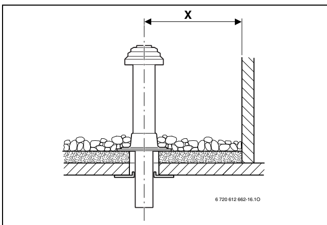
Fig. 6 Distancias en tejados planos
