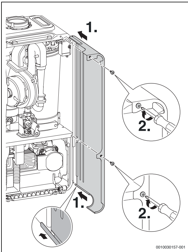
Fig. 70 Colocar nuevamente el revestimiento lateral
