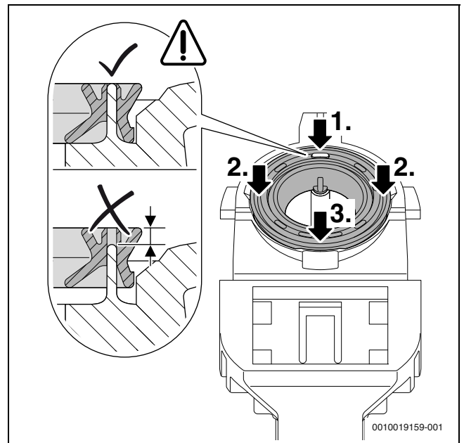
Fig. 56 Aplicar presión en la junta
