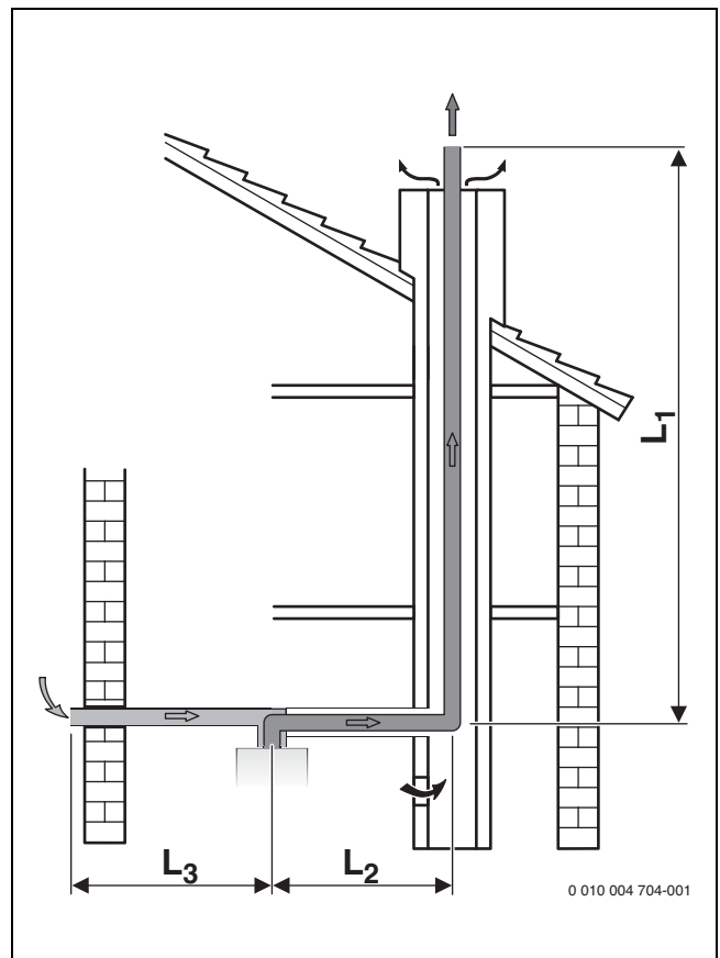
Fig. 11 Evacuación de gases en chimenea según C 53
