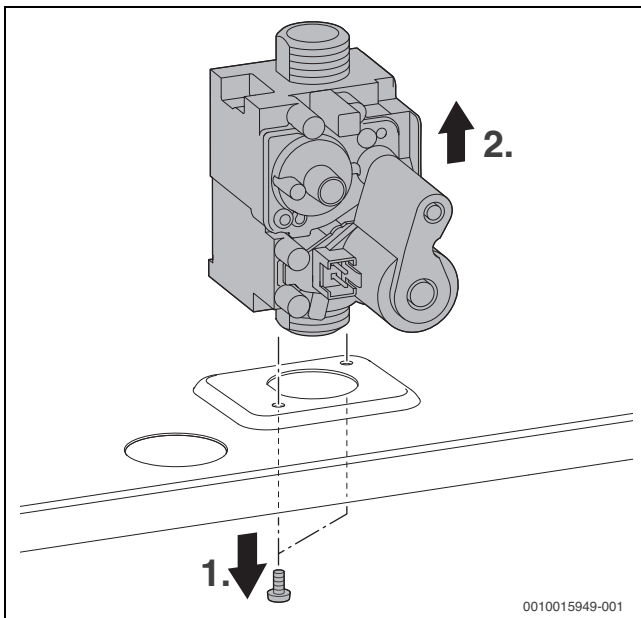
Fig. 62 Desmontar la válvula del gas
