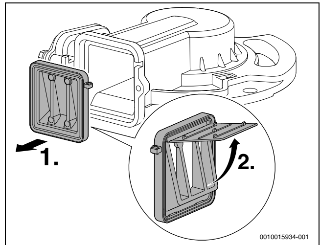
Fig. 45 Tapa antirretorno en la máquina mezcladora
