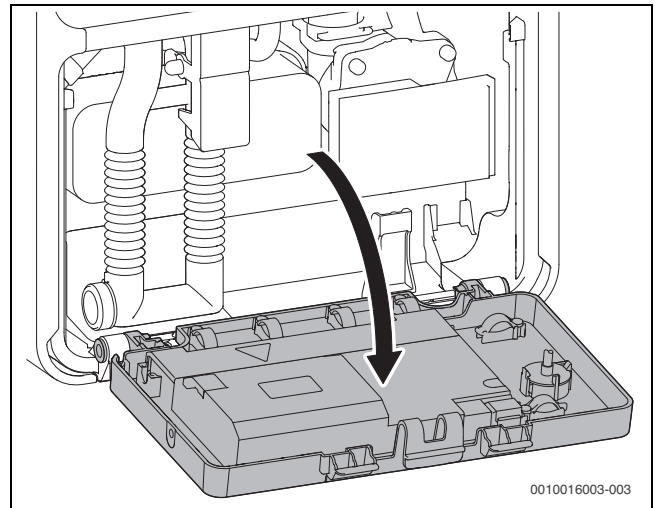
Fig. 28 Plegar la electrónica hacia abajo
