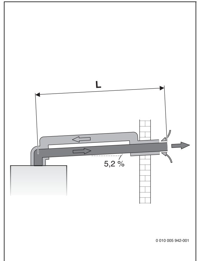
Fig. 14 Evacuación de gases horizontal según C 13
