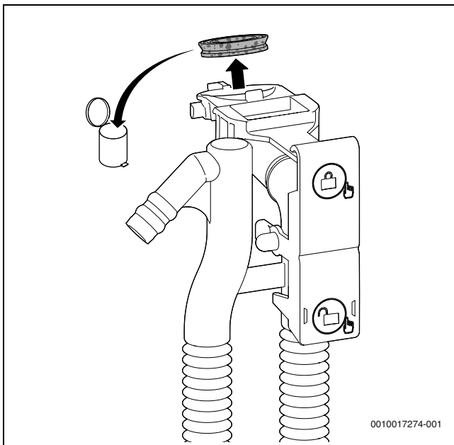
Fig. 54 Retirar la junta en la parte superior del sifón de condensados.
