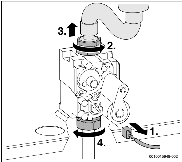
Fig. 61 Retirar el enchufe y las tuercas de racor
