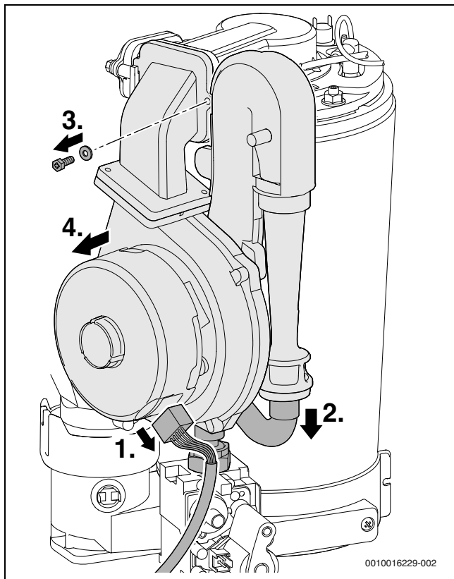
Fig. 43 Desmontar el ventilador con máquina de mezcla
