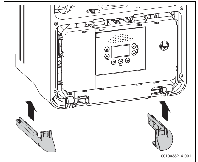
Fig. 71 Colocar el listón lateral de plástico
