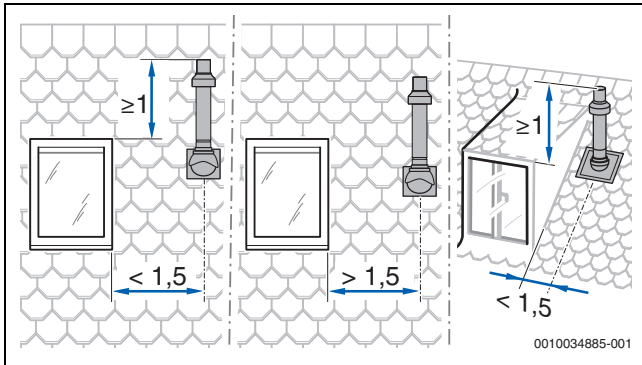
Fig. 5 Distancias mínimas a las ventanas del tejado
