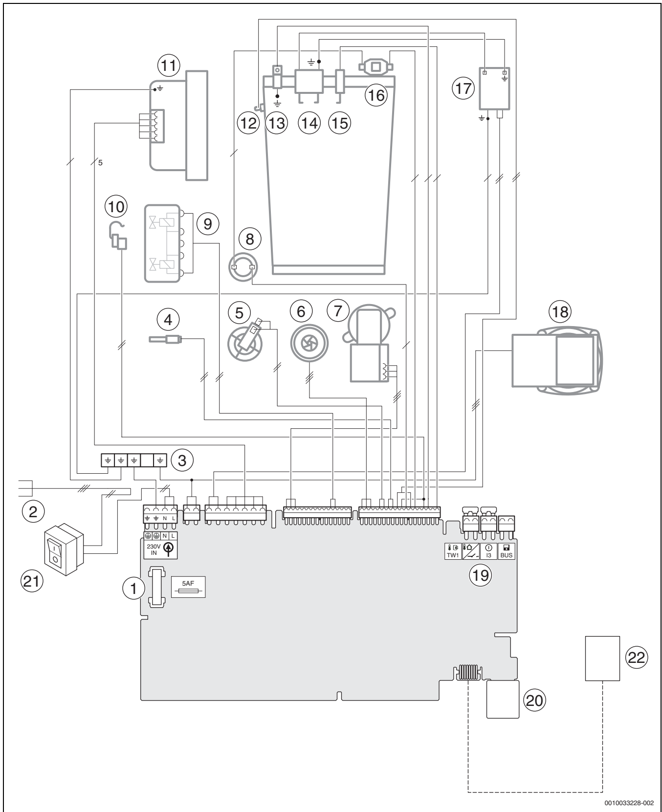
Fig. 73 Cableado eléctrico
