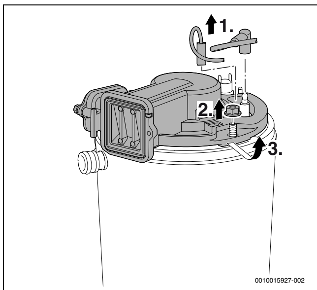
Fig. 44 Soltar la tapa de quemador
