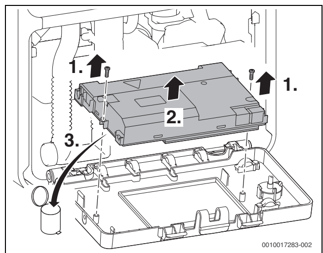
Fig. 68 Cambiar la electrónica del aparato
