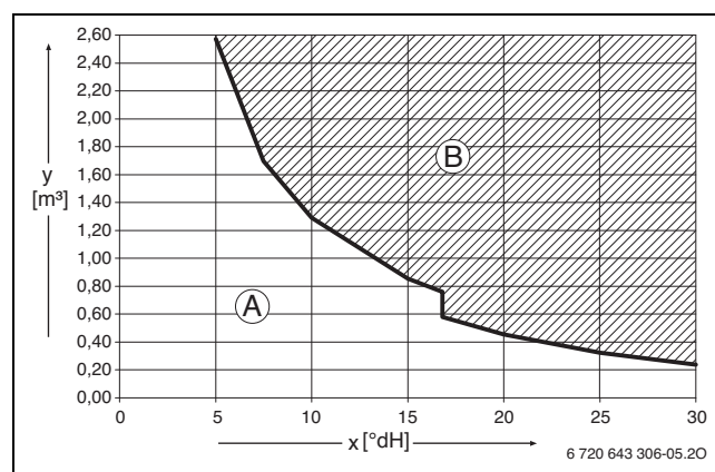
Fig. 21 Requisitos en aparatos < 50 kW de agua de llenado y rellenado en °dH
