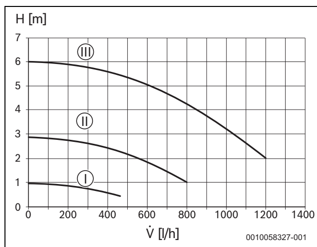
Fig. 35 Cambiar la curva característica de la bomba de circulación (presión constante)
