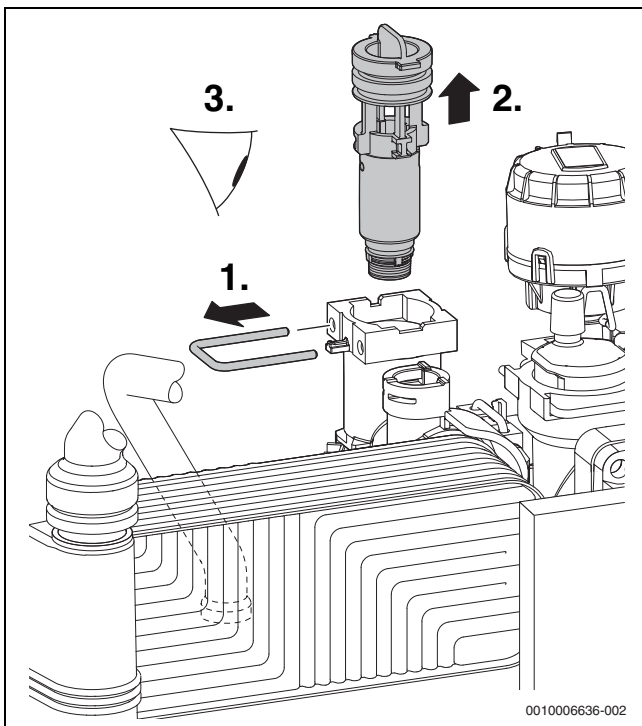
Fig. 59 Controlar el tamiz en el tubo de agua fría
