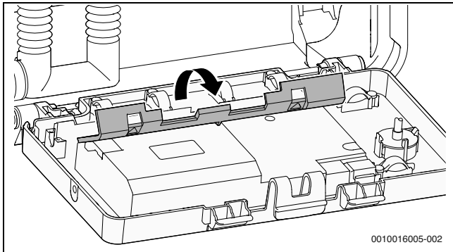
Fig. 29 Desplegar el recubrimiento
