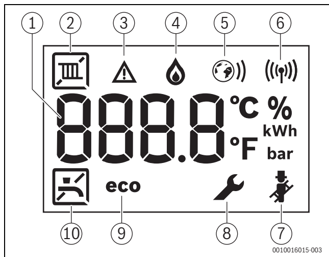
Fig. 32 Indicaciones del display
