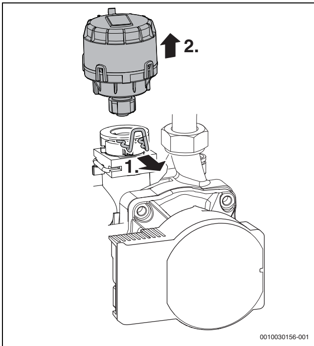
Fig. 65 Desmontar el motor de la válvula de 3 vías
