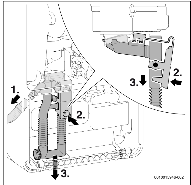
Fig. 52 Desmontar el sifón de condensado
