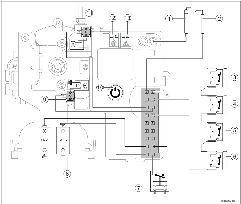
Fig. 27 Esquema eléctrico
