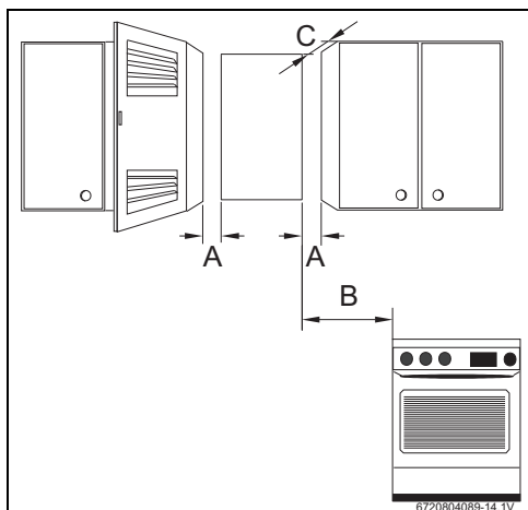
Fig. 19 Distancias mínimas
