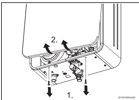
Fig. 24 Retirar la parte frontal
