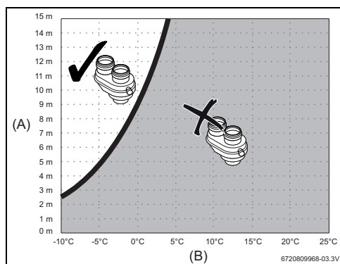
Fig. 10 Conductos separados
