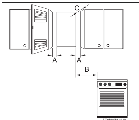
Fig. 12 Distancias mínimas
