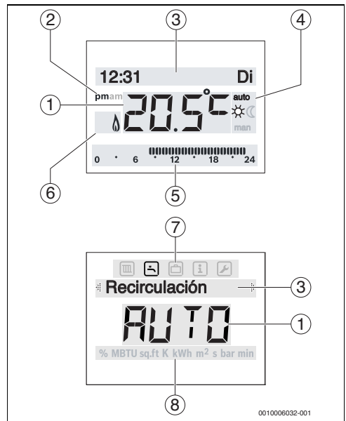
Fig. 2 Símbolos del display (representaciones de ejemplo)
