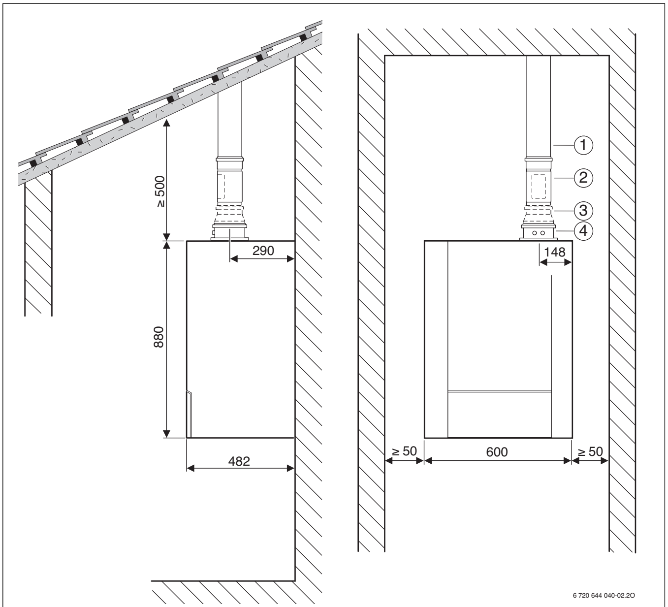
Fig. 8 Tejado inclinado
