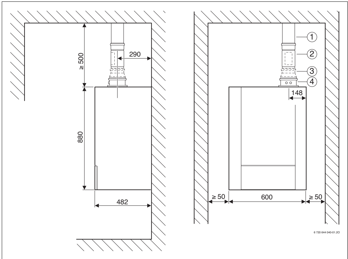
Fig. 7 Tejado plano
