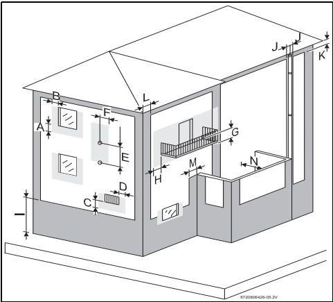
Fig. 13 Distancias mínimas a punto de combustión
