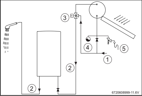
Fig. 11 Sistema solar
