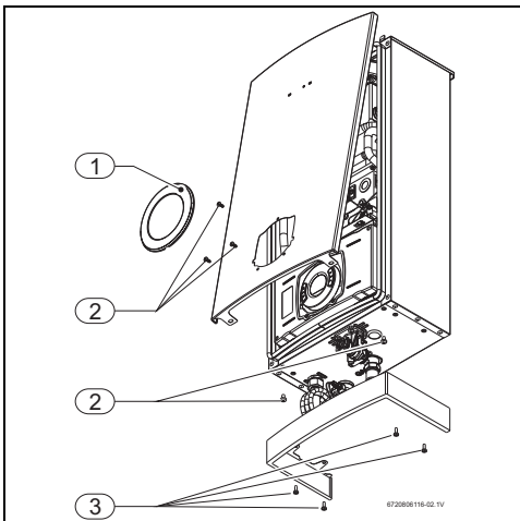
Fig. 19 Retirar la parte frontal
