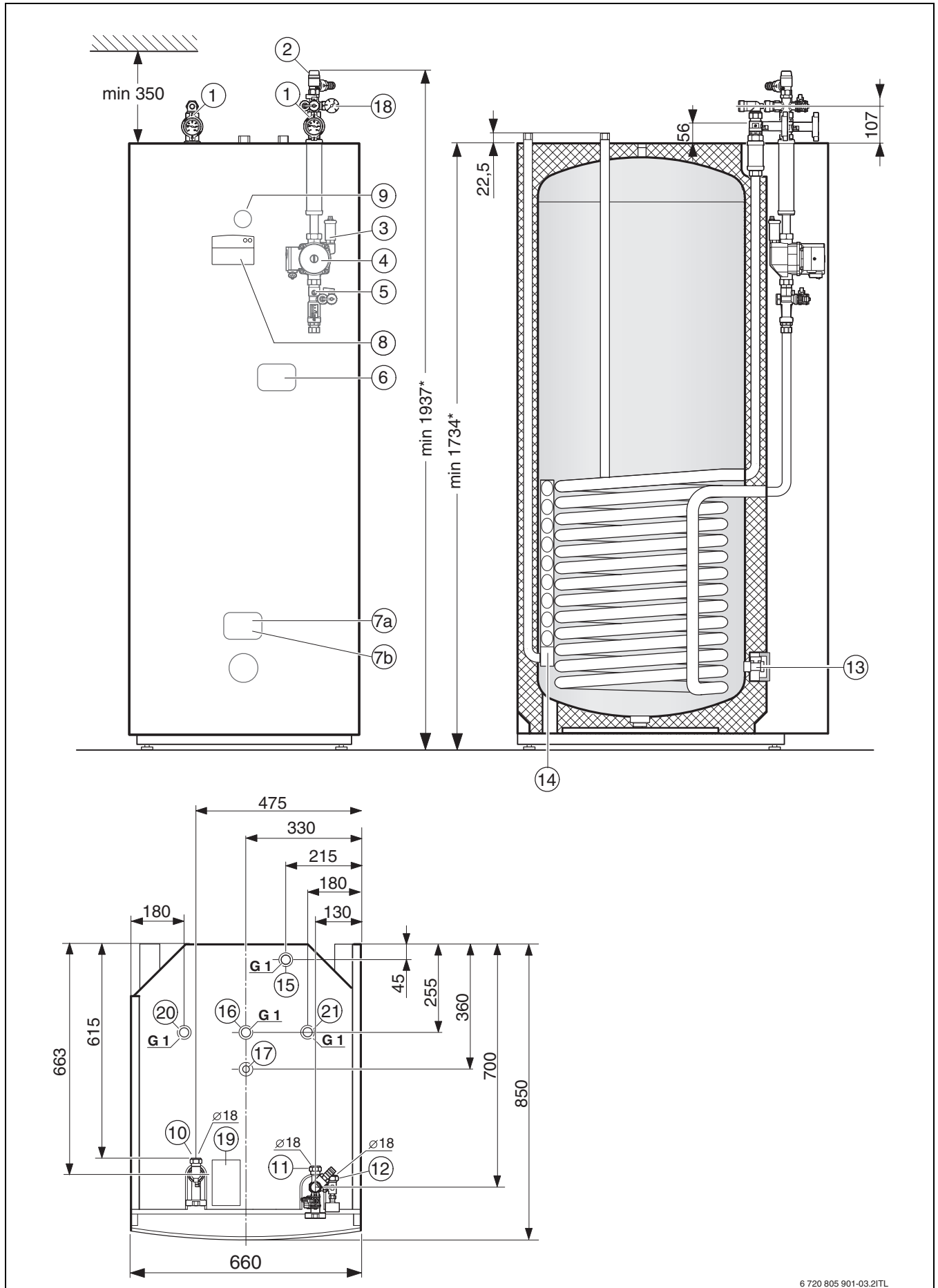
Fig. 2 Dimensiones de construcción y de conexión SP 400 SHU-2
