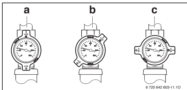
Fig. 21 Dispositivo de cierre con freno por gravedad en el retorno
