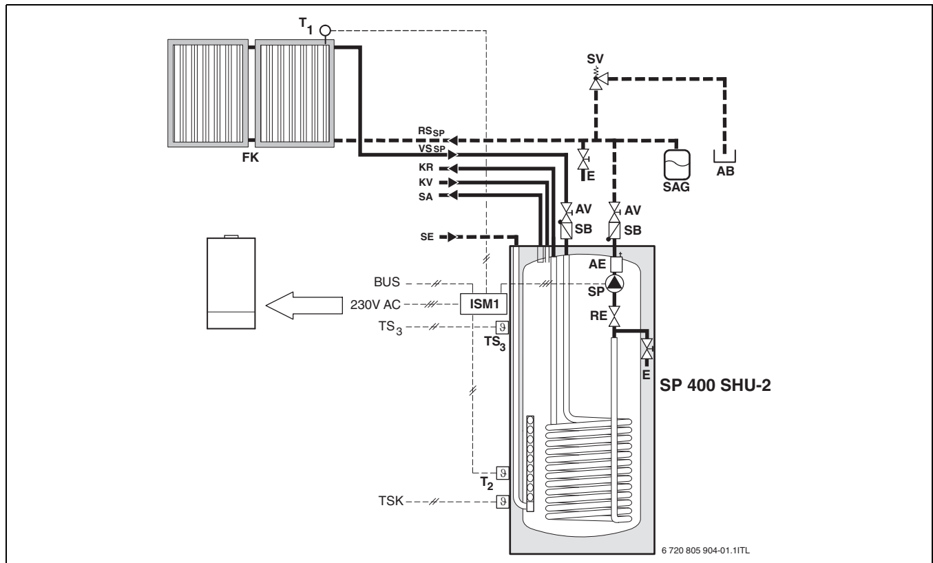
Fig. 5 Instalación solar con SP 400 SHU-2. Esquema de la instalación simplificado (representación correspondiente al montaje y otras posibilidades en los documentos de planificación)
