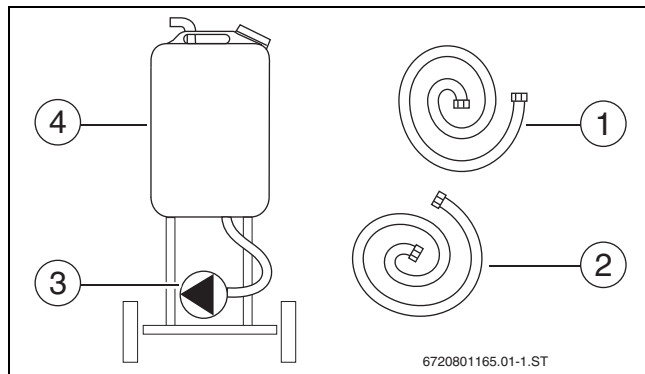
Fig. 18 Componentes de un dispositivo de relleno
