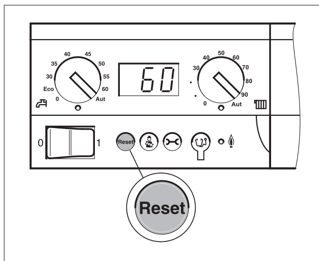
Fig. 9 Puesta a cero de la avería mediante la tecla "Reset"
