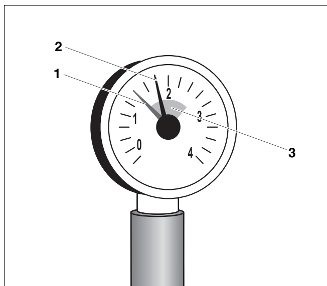
Fig. 7 Manómetro para instalaciones cerradas
