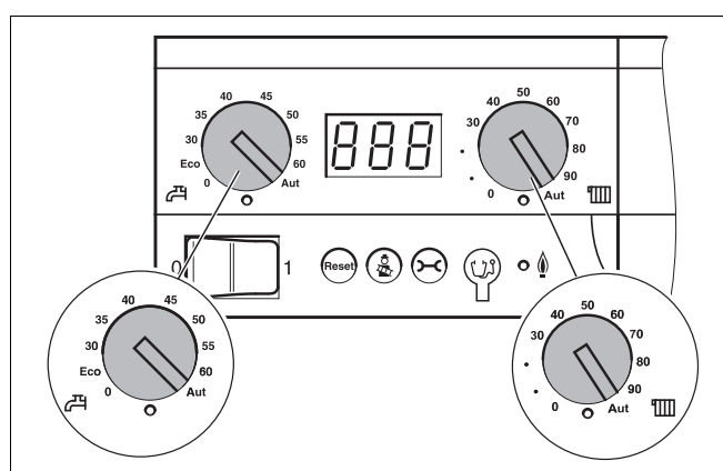
Fig. 3 Ajuste del aparato de regulación
