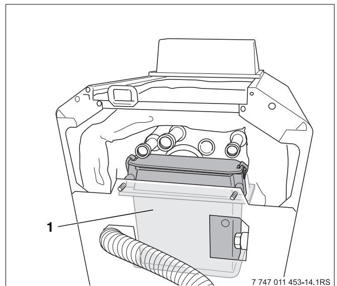
Fig. 2 Vista posterior Suprapur-O KUB 22...35 (representación sin aislamiento térmico)
