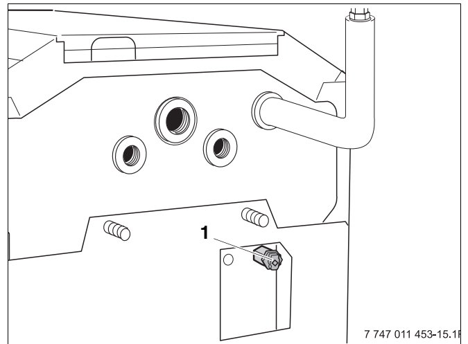
Fig. 8 Purgar el intercambiador de calor
