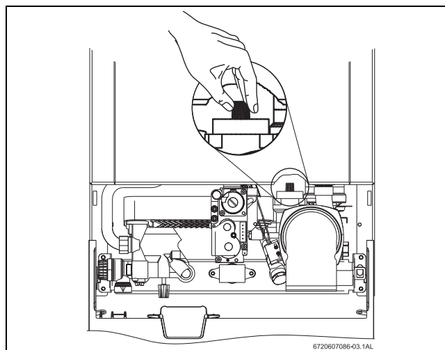
Fig. 14 Purgador automático
