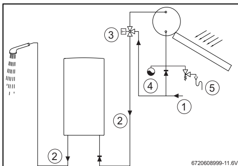
Fig. 18 Instalación solar
