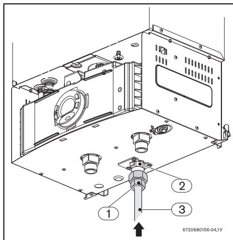
Fig. 22 Conexión del tubo de gas
