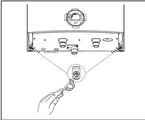
Fig. 19 Retirar los dos tornillos
