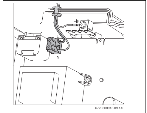
Fig. 33 Conexiones del cable de alimentación
