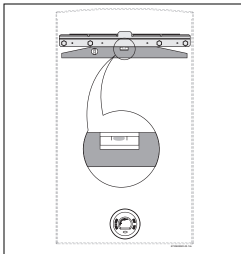
Fig. 18 Fijar la barra de fijación
