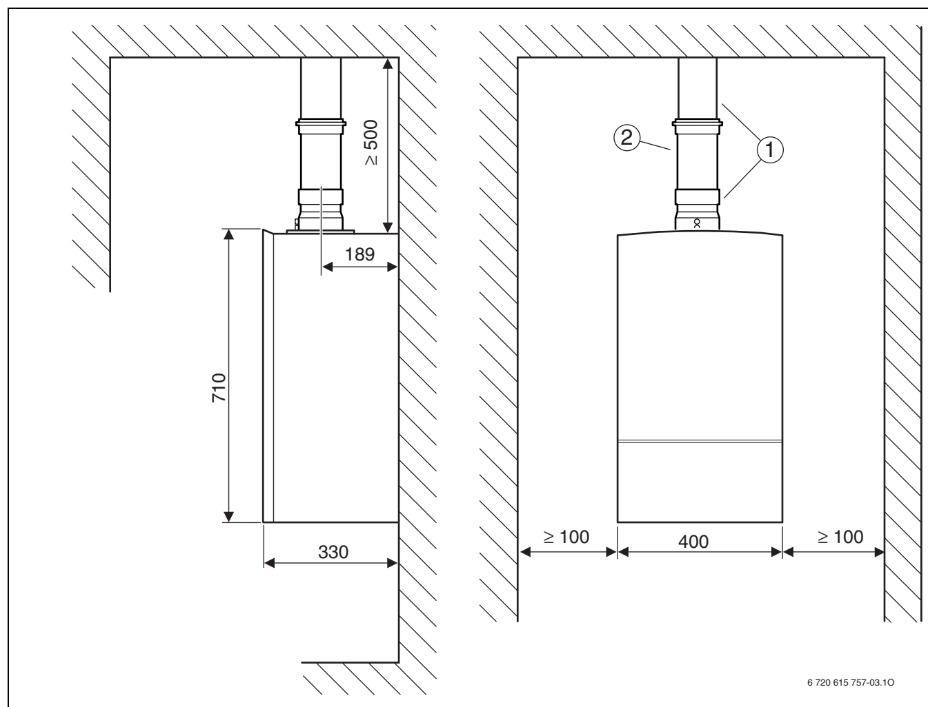
Fig. 7 Conducción de gases Ø 60/100 mm o Ø 80/125 mm, techo plano
