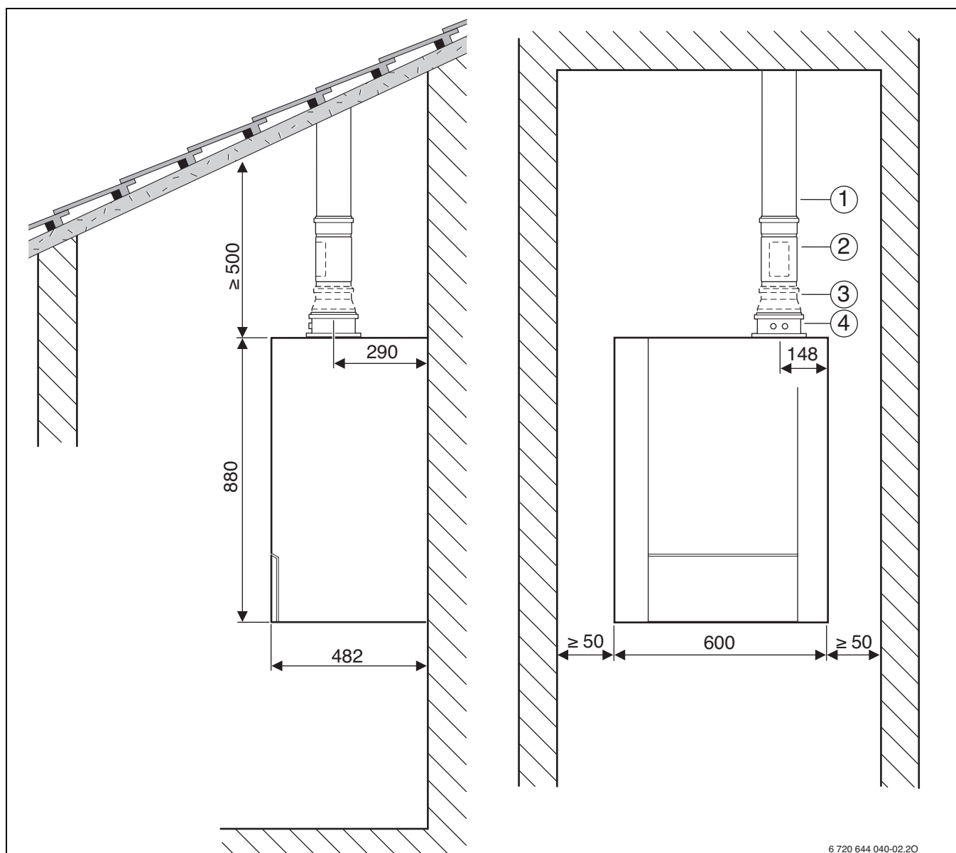
Fig. 8 Tejado inclinado
