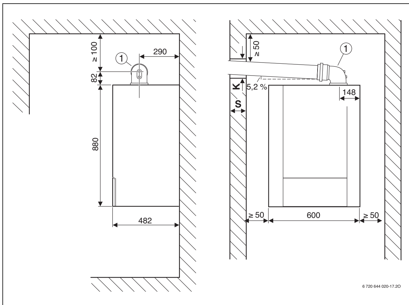
Fig. 6 Conducción de gases Ø 60/100 mm
