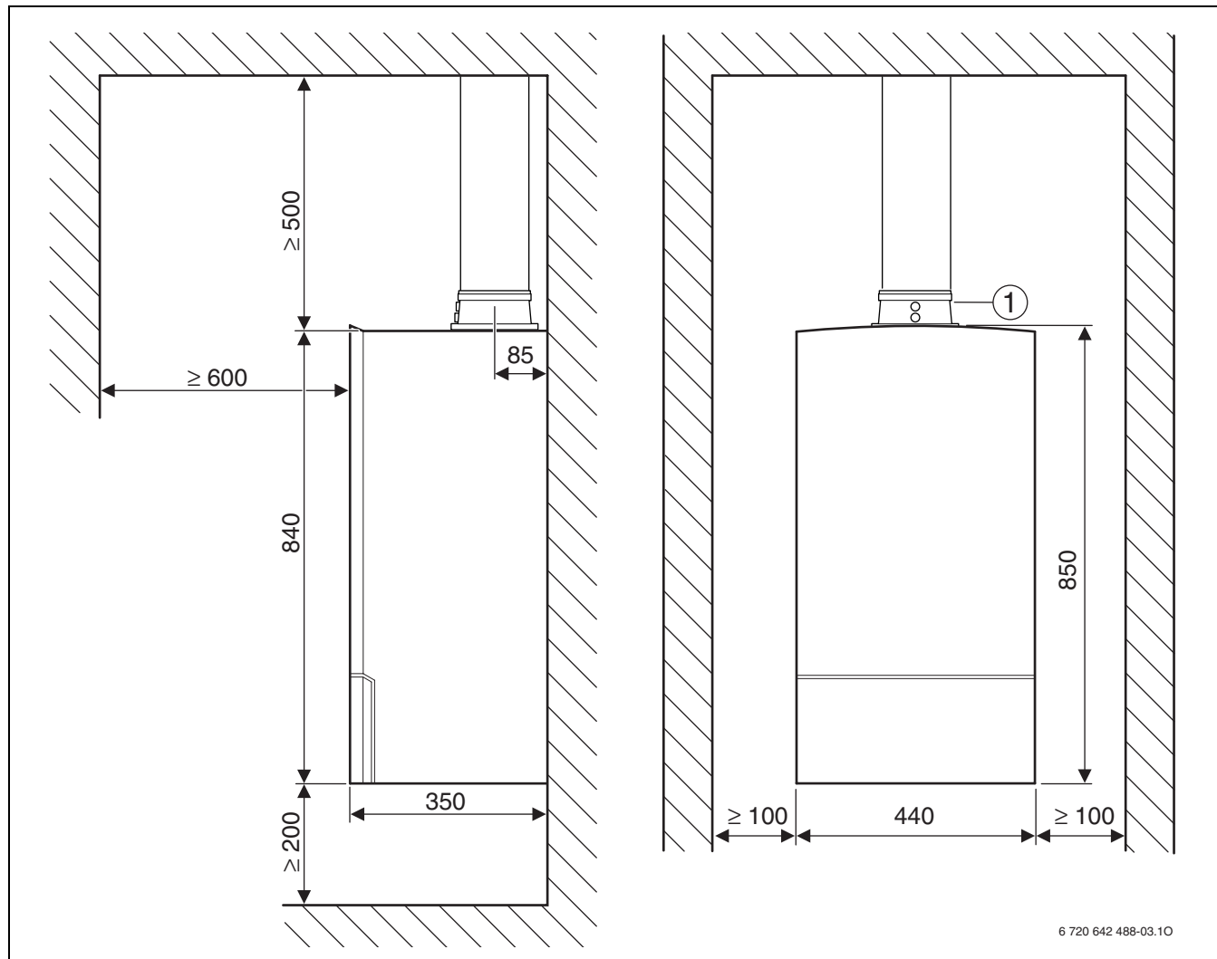
Fig. 7 Techo plano
