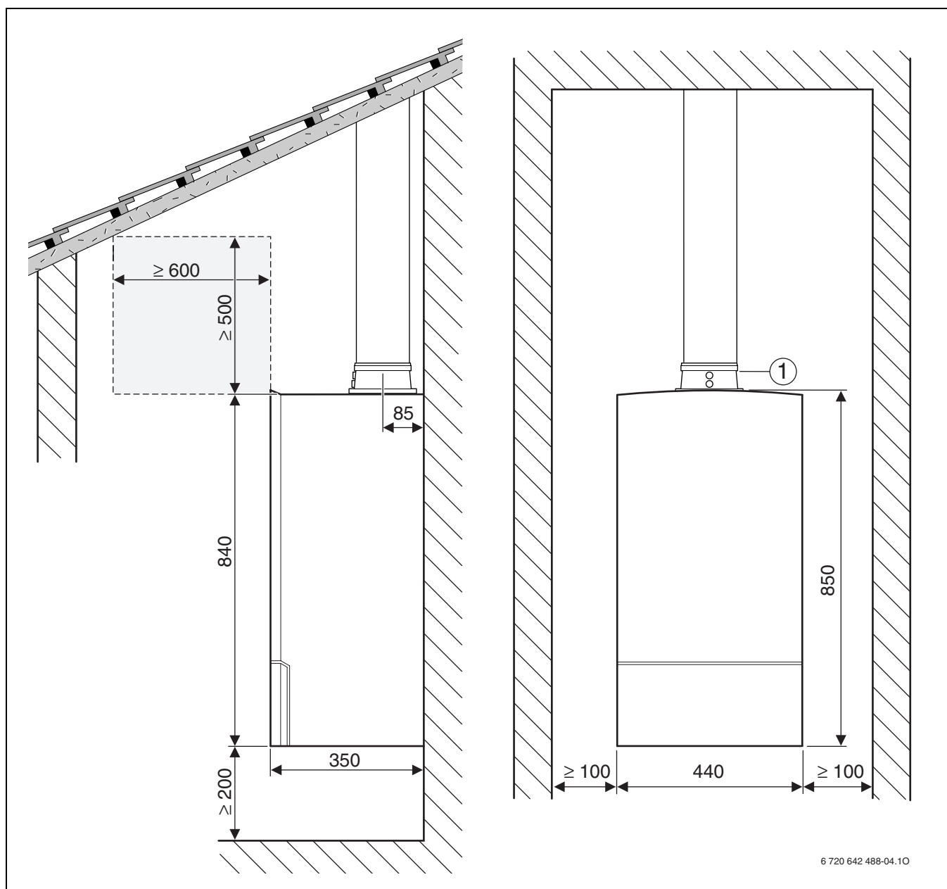
Fig. 8 Techo inclinado
