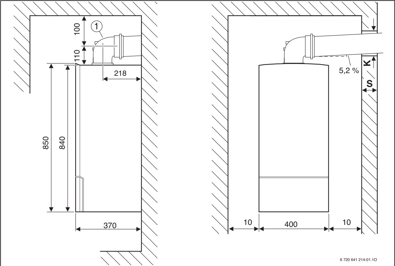
Fig. 5 Ø 80/125 mm
