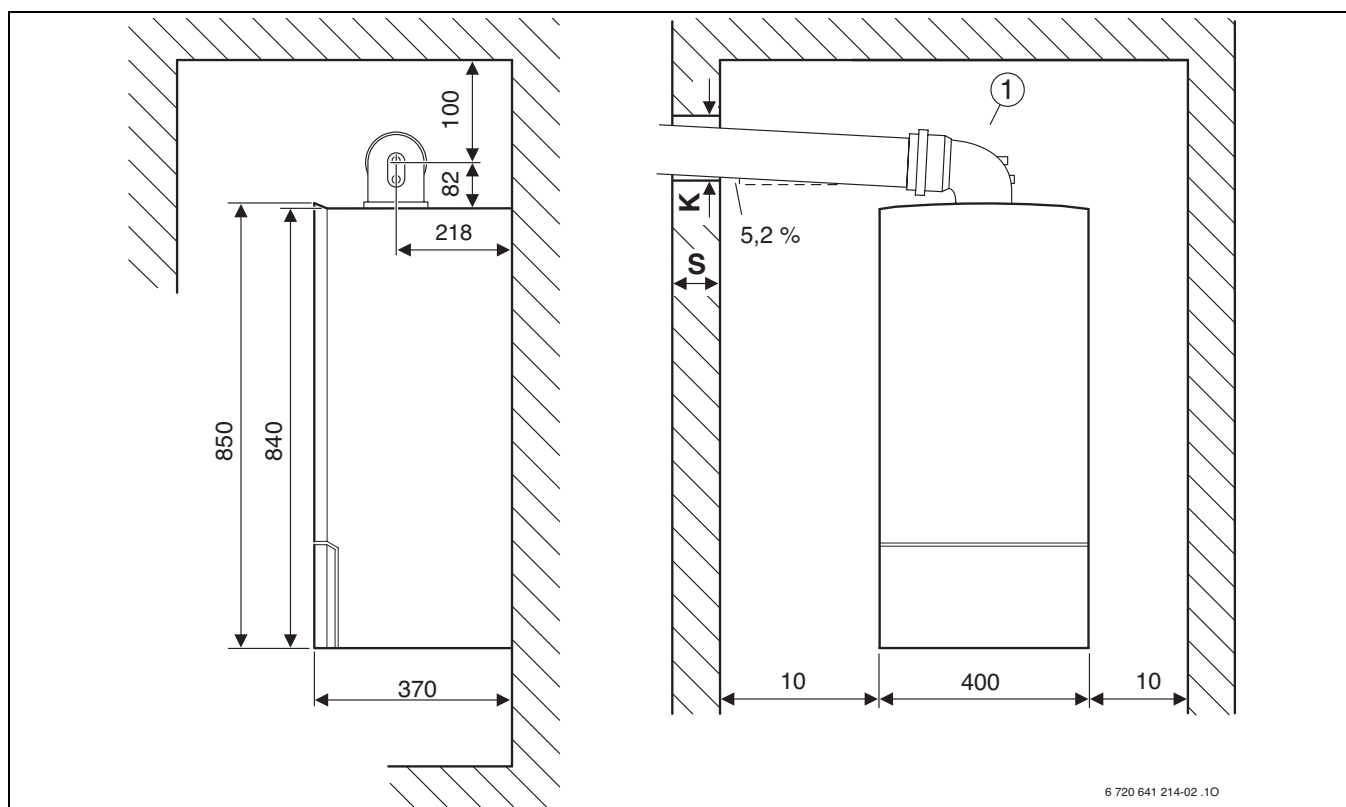
Fig. 6 Ø 60/100 mm
