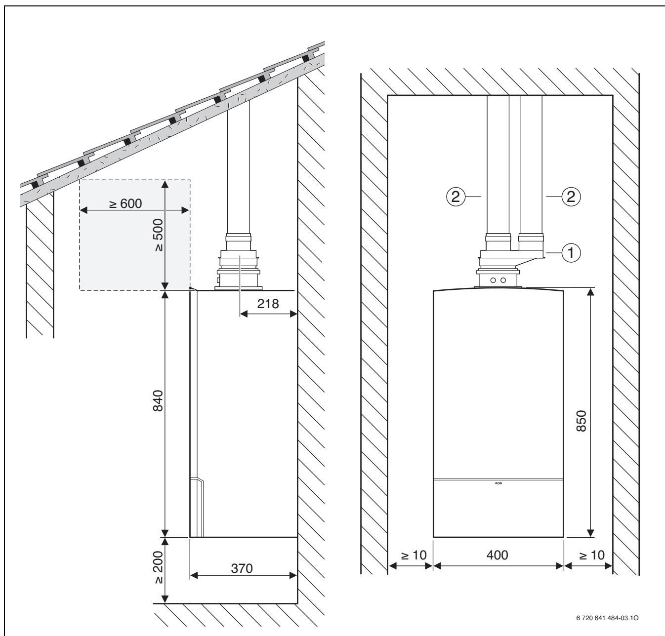
Fig. 11 Salida paralela Ø 80/80 mm, techo inclinado
