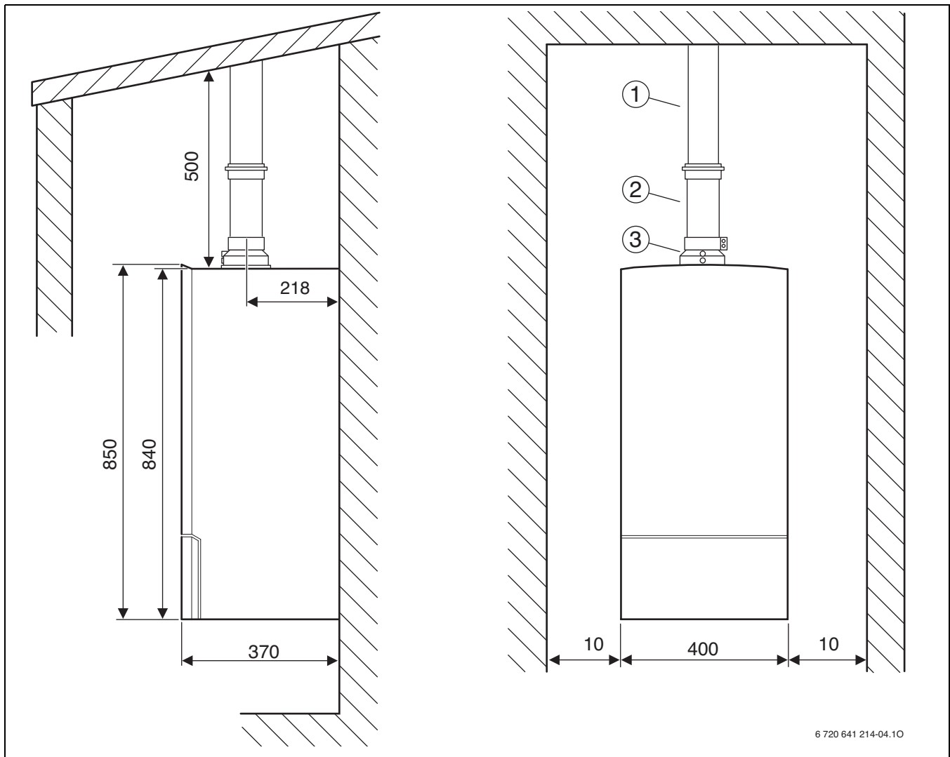
Fig. 10 Techo inclinado
