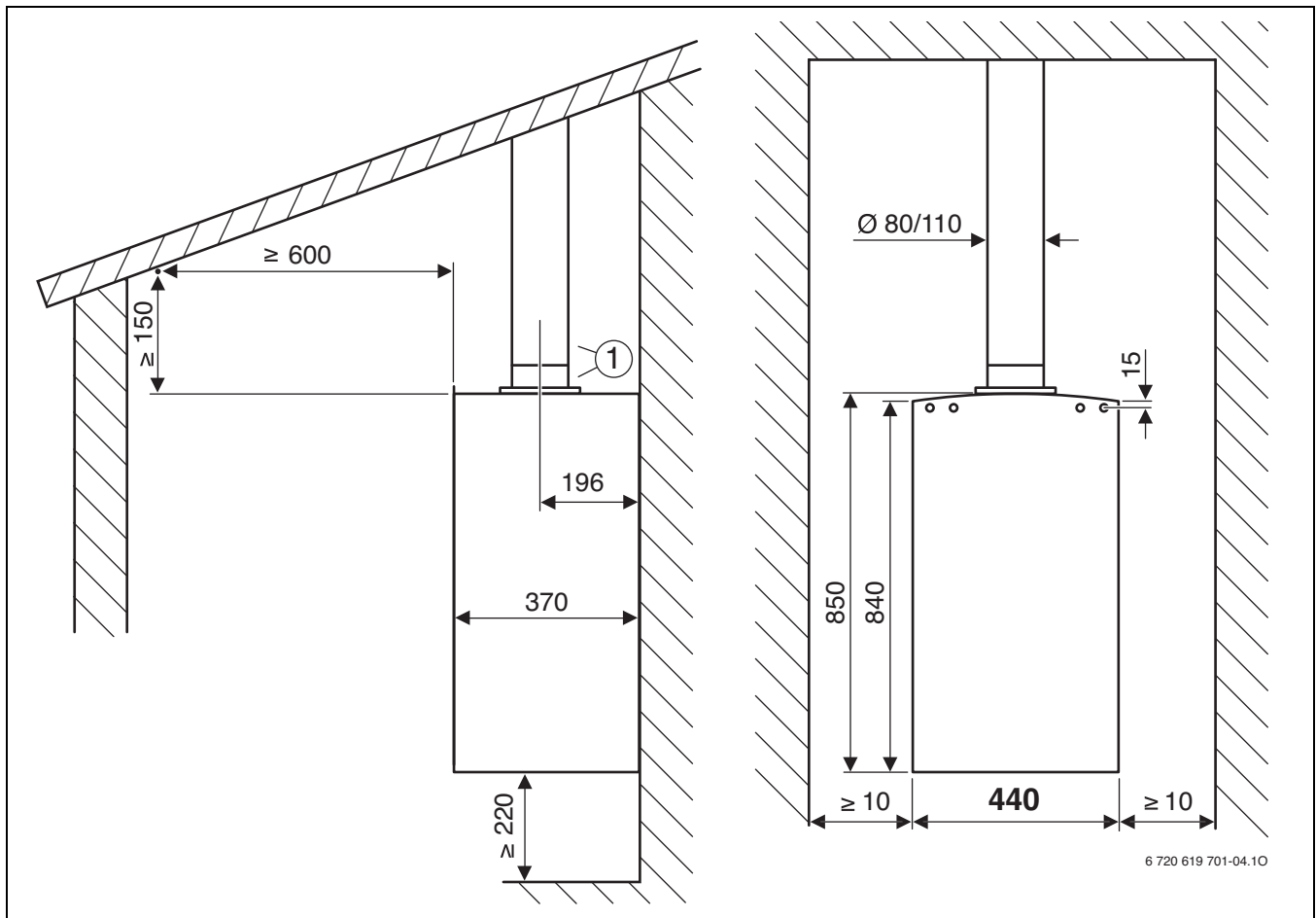
Fig. 5 Tejado inclinado
