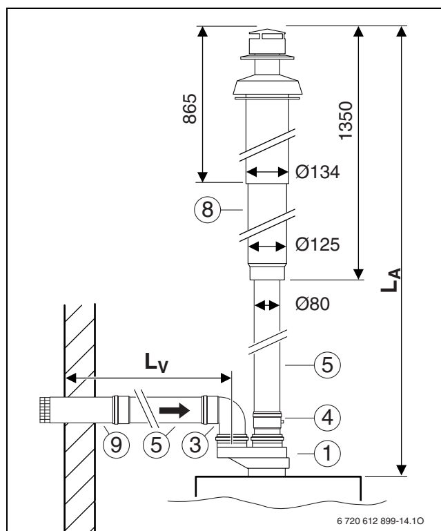
Fig. 15 Conducto de evacuación-admisión según C 52
