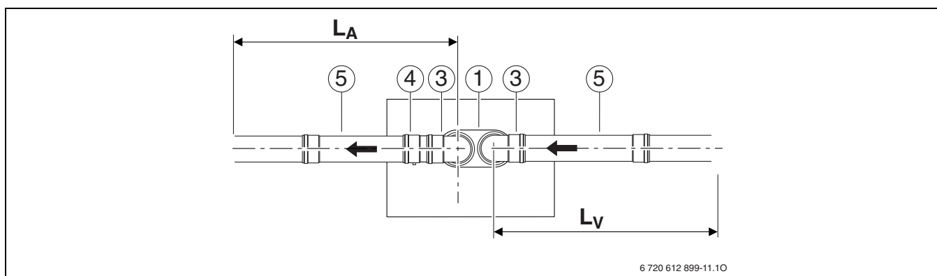
Fig. 13 Conducto de evacuación-admisión según C 42 , C 52 y C 82
