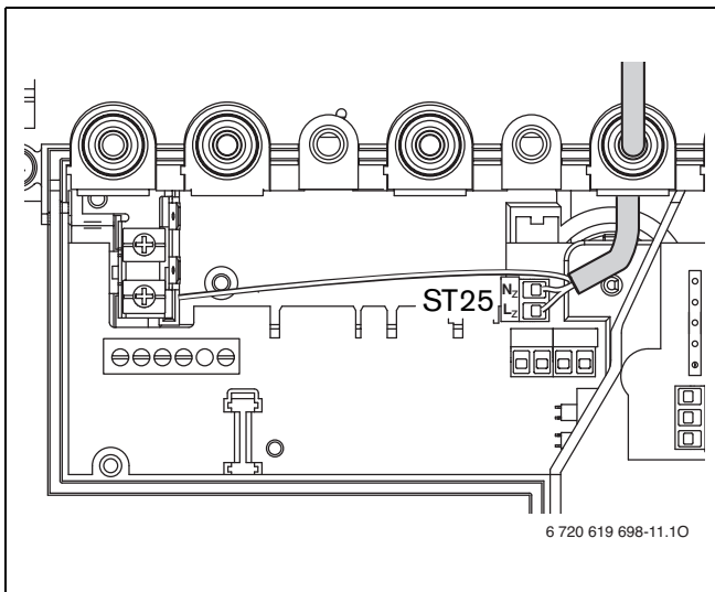
Fig. 21 Conexión de la bomba de recirculación
