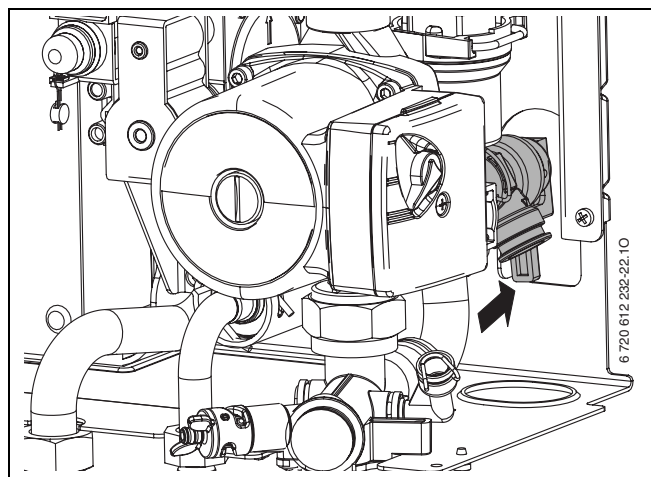
Fig. 58 Válvula de seguridad de la calefacción
