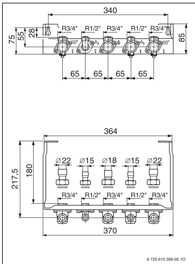
Fig. 6 Conexiones para las tuberías
