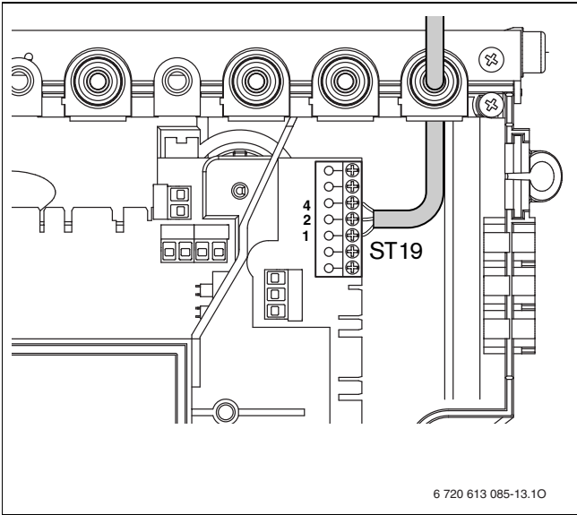
Fig. 20 Conexión del regulador de 24 V
