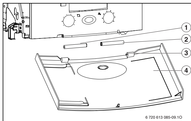
Fig. 10 Montaje de la tapa
