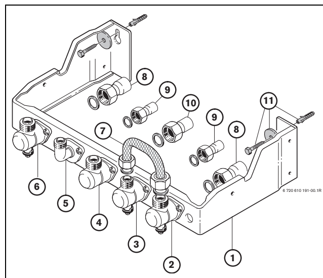
Fig. 7 Plantilla de montaje
