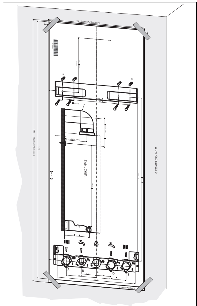
Fig. 5 Plantilla de montaje
