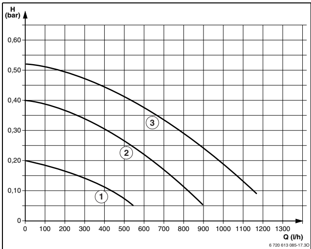
Fig. 33 Curvas características de la bomba (sin placa de conexión para montaje)
