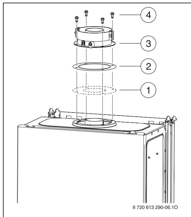
Fig. 12 Colocar el adaptador
