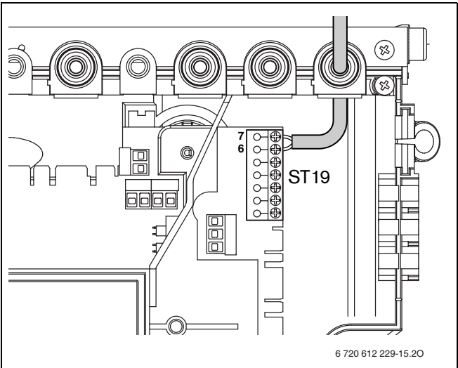
Fig. 18 Conexión del regulador
