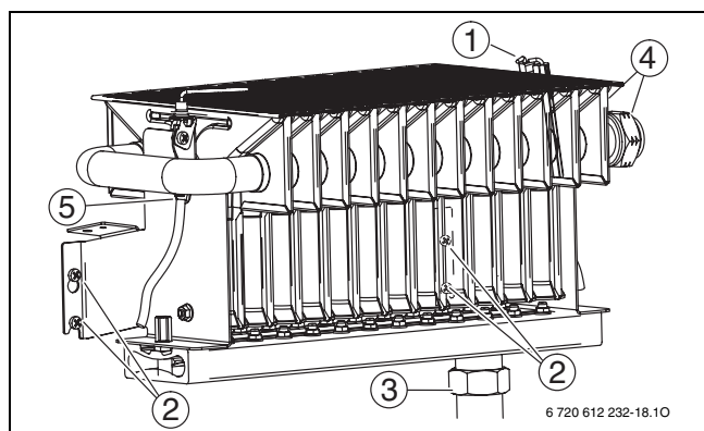
Fig. 49 Módulo de quemador
