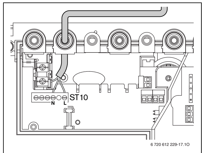
Fig. 22 Regleta de conexión de tensión de alimentación ST10
