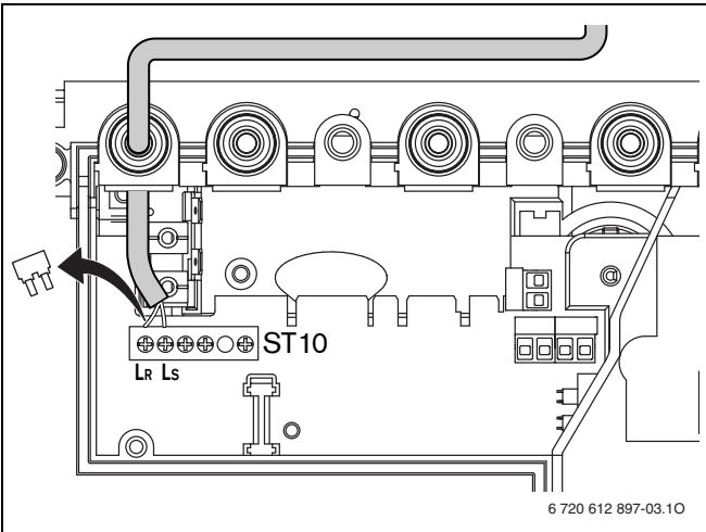
Fig. 17 Conexión (230 V AC, retirar el puente entre L S y L R )
