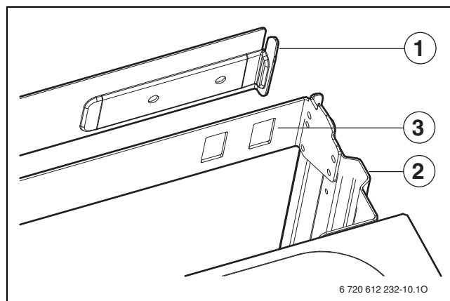
Fig. 9 Enganche del aparato a la pletina de sujeción
