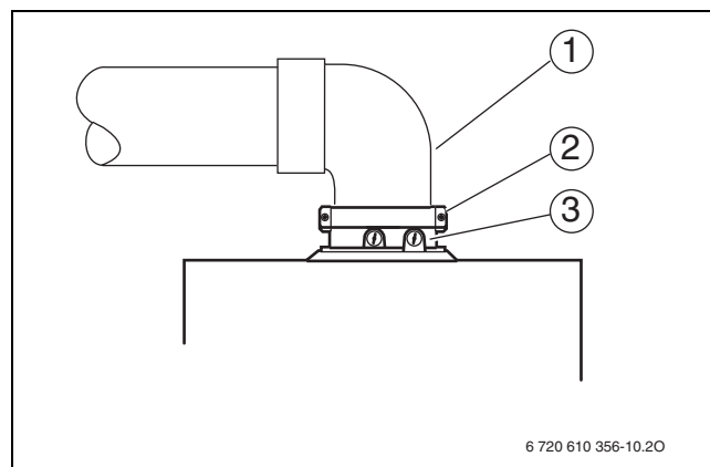
Fig. 13 Sujeción del codo de evacuación con abrazadera
