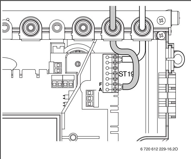
Fig. 19 Conexión de la sonda de temperatura exterior
