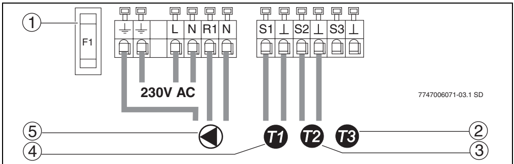
Fig. 6 Esquema de ligações
