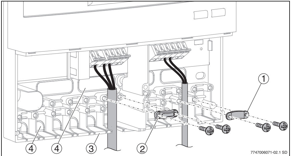
Fig. 5 Passaggio e fissaggio dei cavi
