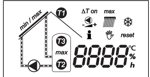
Fig. 2 Possíveis mensagens no visor
