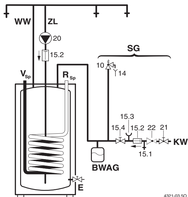
Fig. 4 Esquema de conexión al ramal de agua potable
