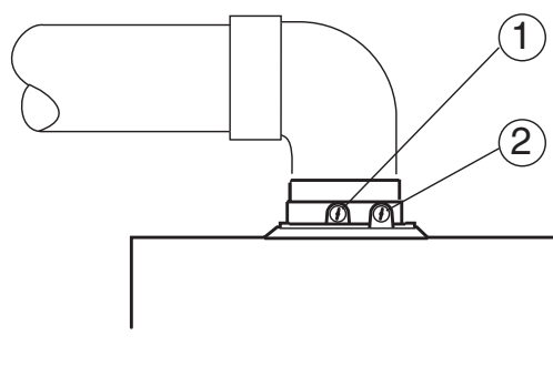
Fig. 56 Medición de los productos de la combustión
