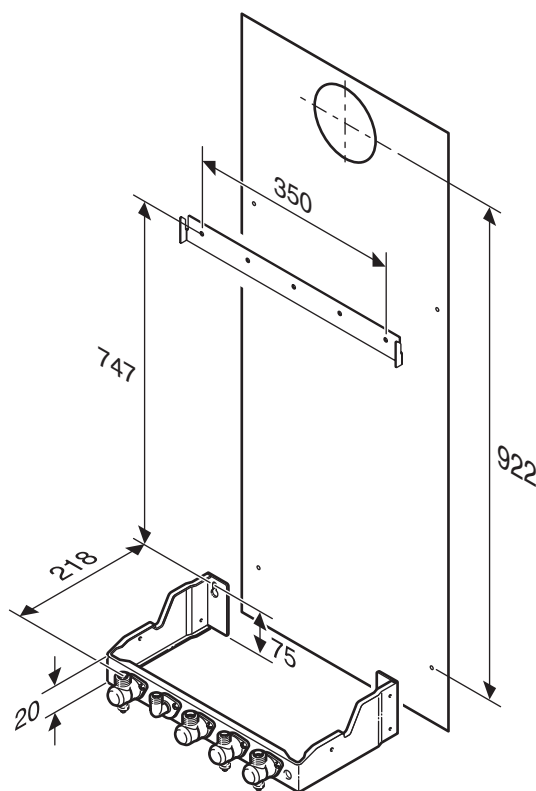
Fig. 4 (en mm)
