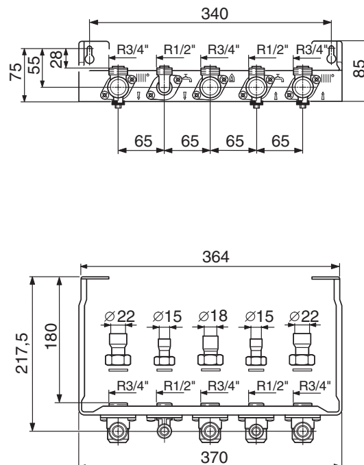
Fig. 5 Conexiones para las tubería (en mm)
