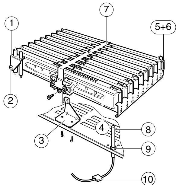
Fig. 41 Unidad de quemador
