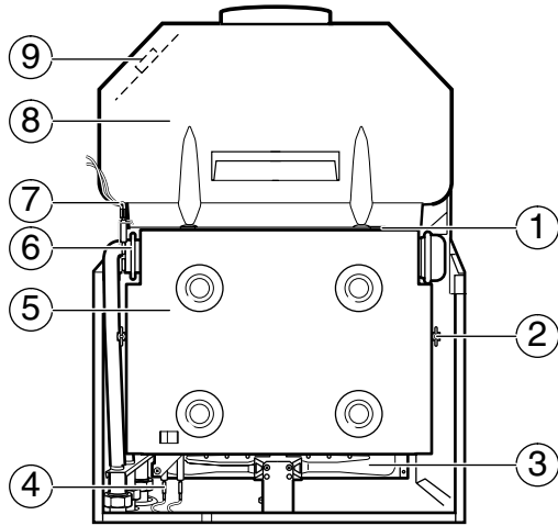
Fig. 39 Componentes situados detrás de la cubierta termoaislante
