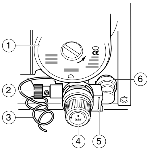
Fig. 22 Válvula de seguridad
