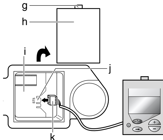
Fig. 18 Tapa falsa
