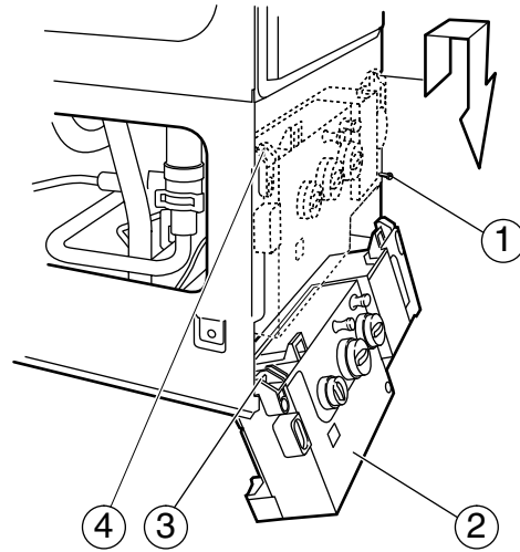
Fig. 38 Colocación de la Eurotronic en posición de servicio
