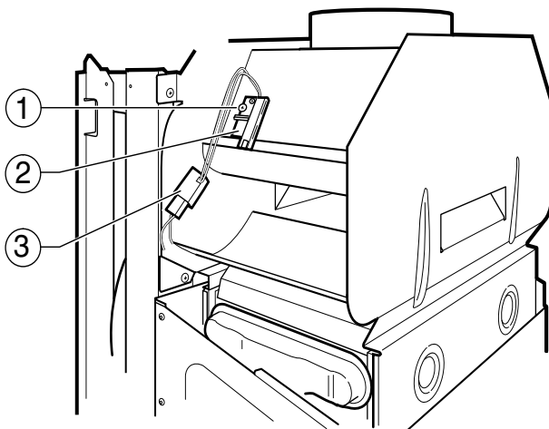
Fig. 40 Sonda de control de los gases de evacuación
