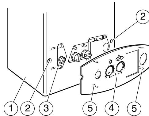
Fig. 36 Carcasa – panel de mandos
