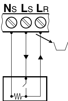
Fig. 15 Conexión del termostato ambiente 230 V (retirar el puente entre L_S y L_R )
