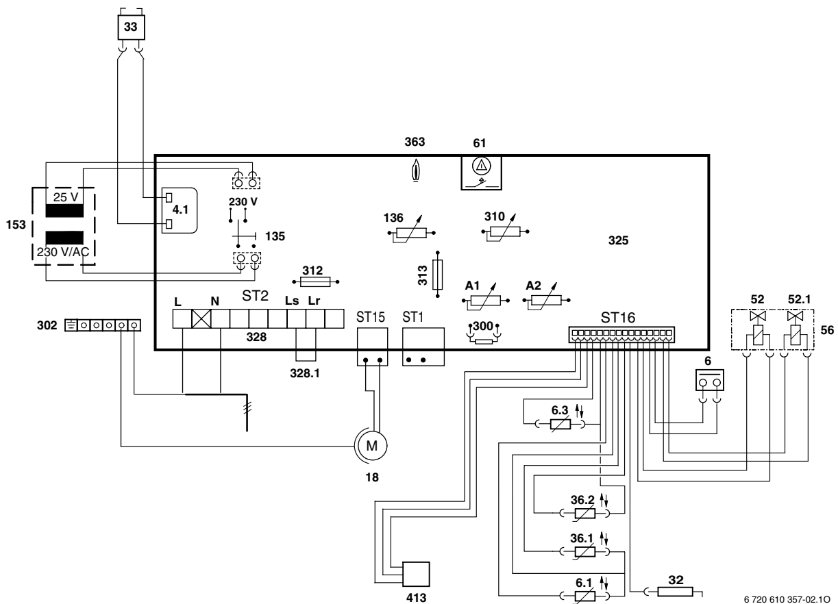
Fig. 2 Cableado eléctrico
