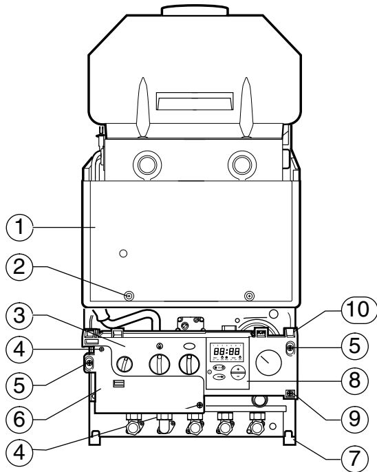
Fig. 37 Sujeción de la cubierta termoaislante y de la Eurotronic
