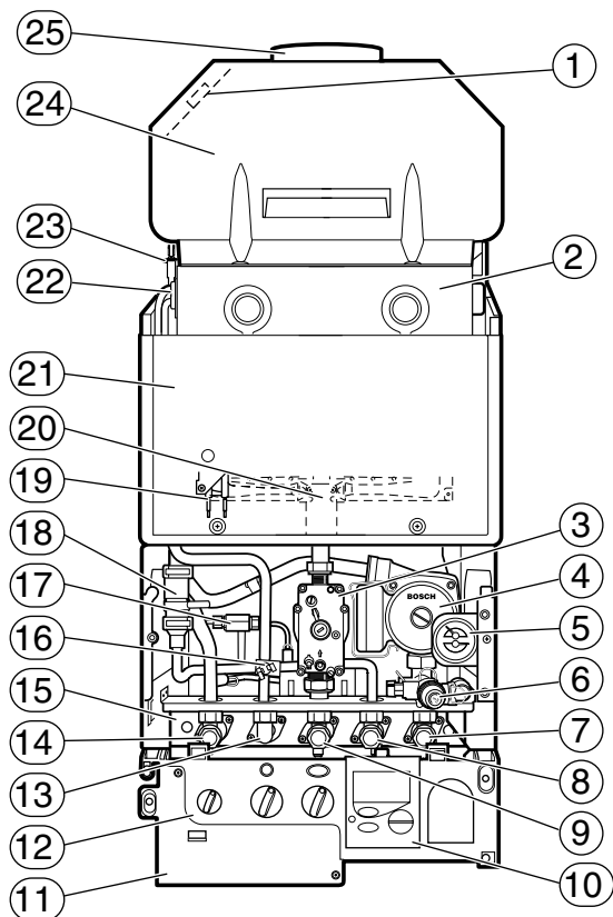
Fig. 19 Componentes del aparato; Eurotronic en posición de servicio
