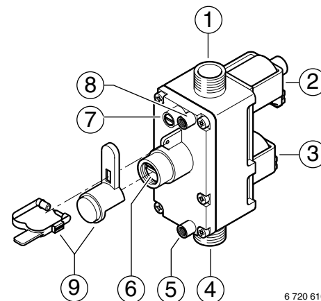
Fig. 24 Cuerpo de gas
