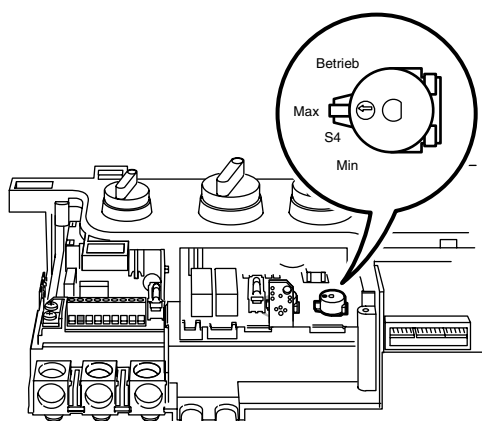
Fig. 27 Selección del modo de operación
