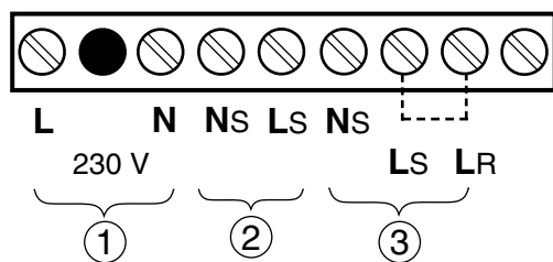
Fig. 15 Regleta para conexión de la tensión de alimentación
