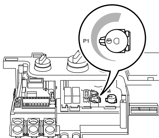
Fig. 28 Ajuste de la potencia máxima de calefacción
