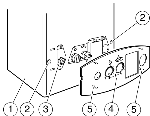
Fig. 39 Carcasa – panel de mandos
