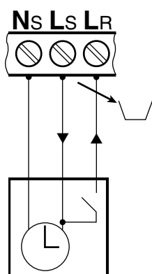
Fig. 18 Conexión del reloj programador 230 V (retirar el puente entre L_S y L_R )
