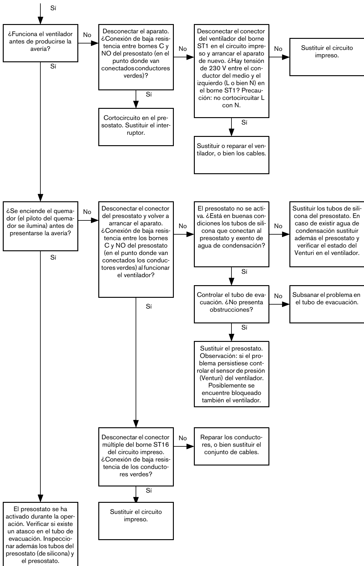
Fig. 55 Prueba E (Capítulo 2 de 2)
