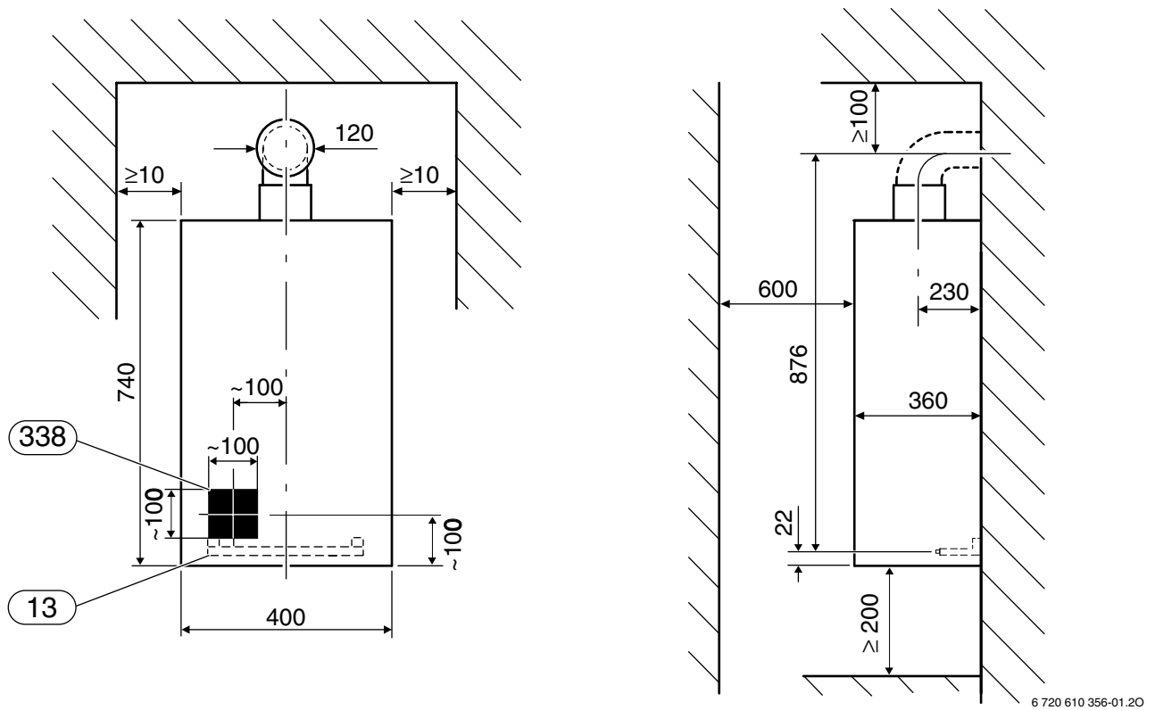
Fig. 1 Vista frontal y lateral
