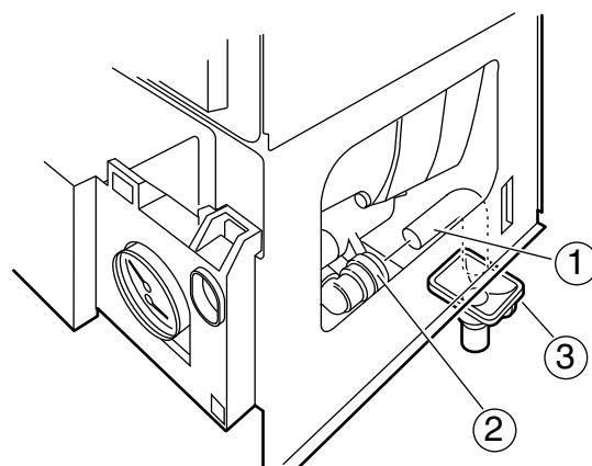
Fig. 10 Montaje de la tubería de desagüe
