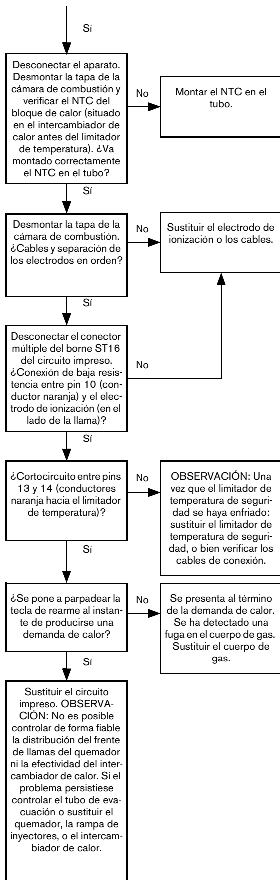
Fig. 53 Prueba D (Capítulo 2 de 2)
