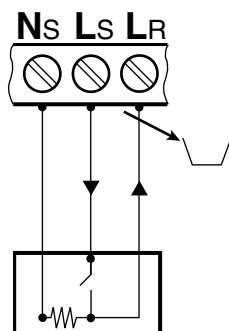
Fig. 17 Conexión del termostato ambiente 230 V (retirar el puente entre L_S y L_R )
