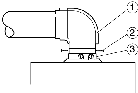
Fig. 12 Sujeción del codo de evacuación con tornillos
