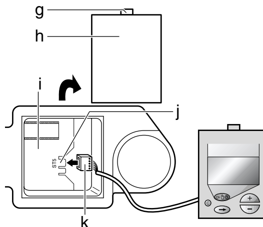
Fig. 20 Tapa falsa
