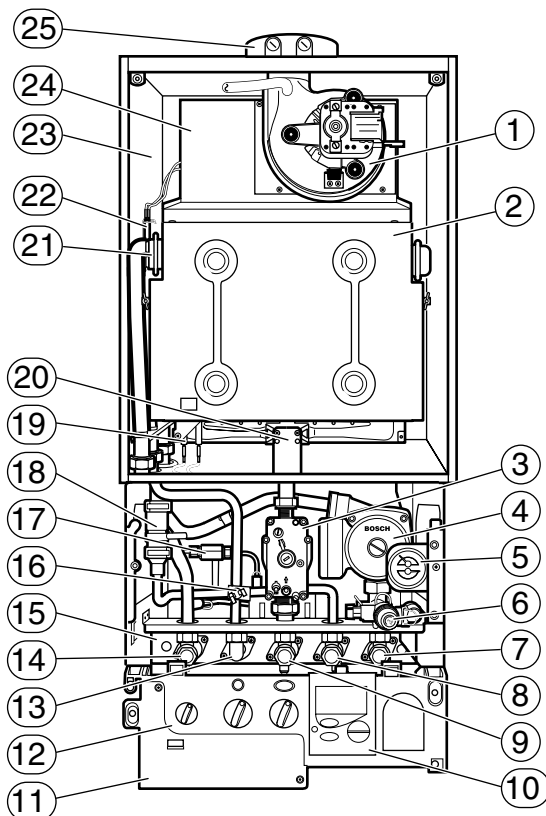
Fig. 21 Componentes del aparato; Eurotronic en posición de servicio
