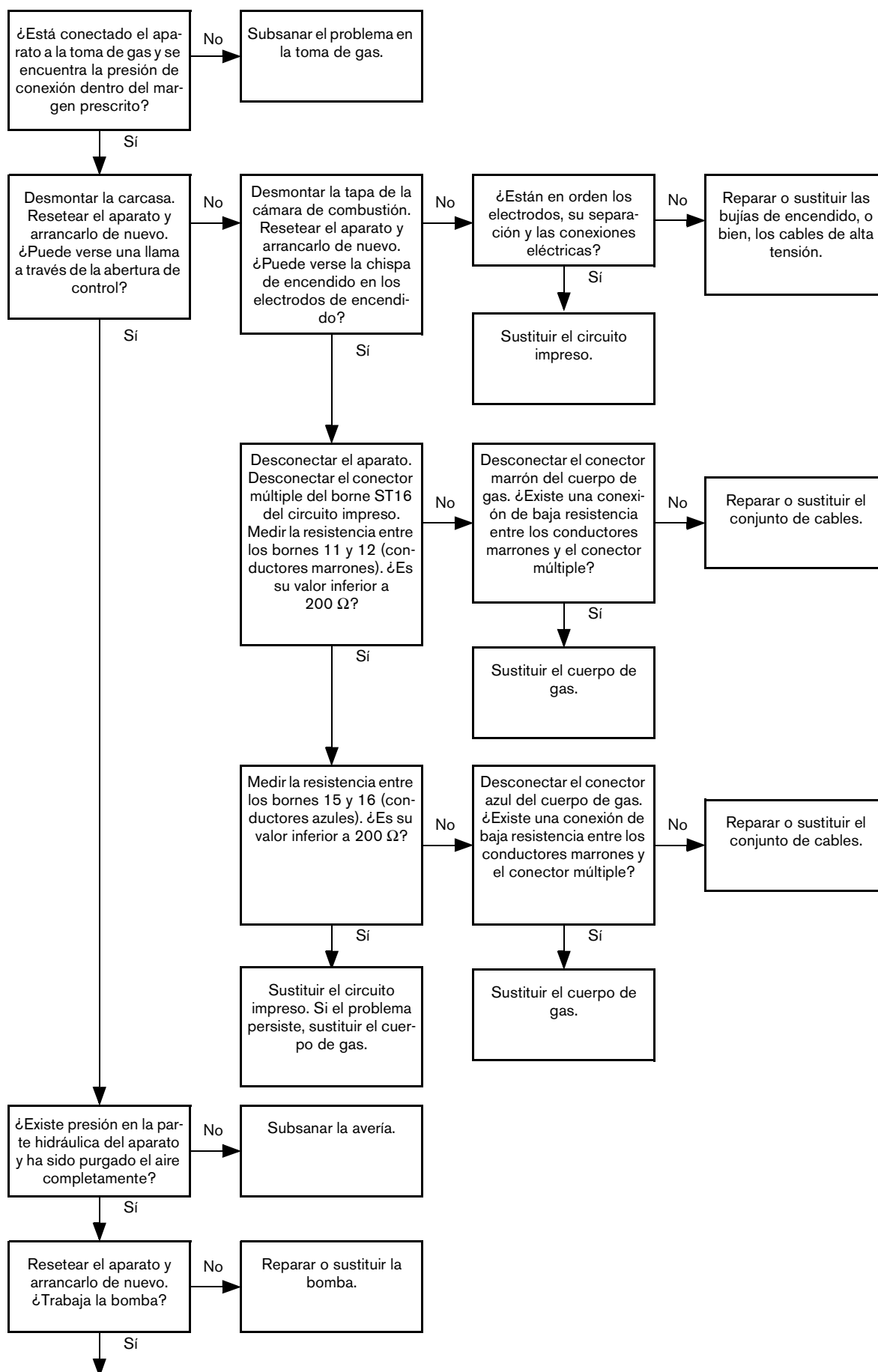
Fig. 52 Prueba D (Capítulo 1 de 2)
