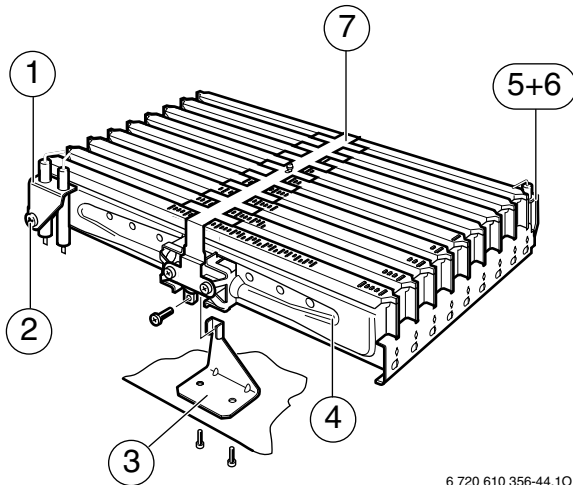
Fig. 46 Unidad de quemador
