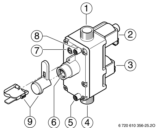
Fig. 26 Cuerpo de gas
