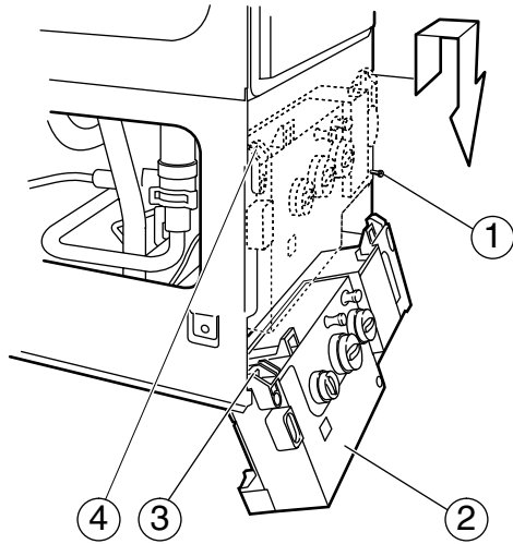
Fig. 41 Colocación de la Eurotronic en posición de servicio
