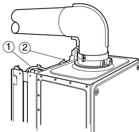
Fig. 22 Purgador automático
