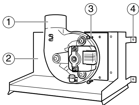
Fig. 43 Ventilador
