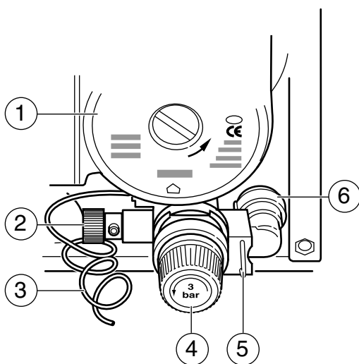
Fig. 24 Válvula de seguridad
