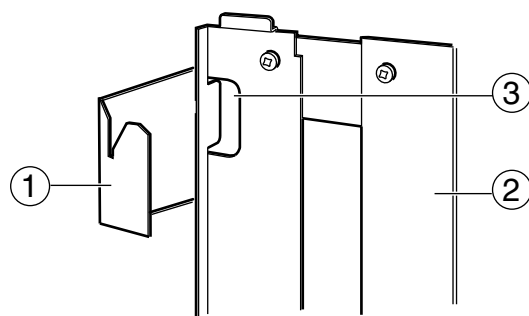
Fig. 9 Sujeción del aparato a la placa de sujeción
