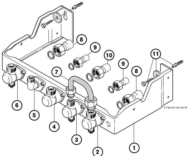
Fig. 7 Plantilla de montaje
