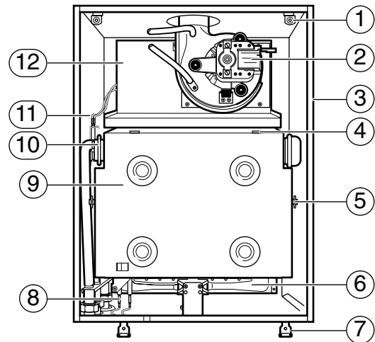
Fig. 42 Componentes en la cámara de combustión
