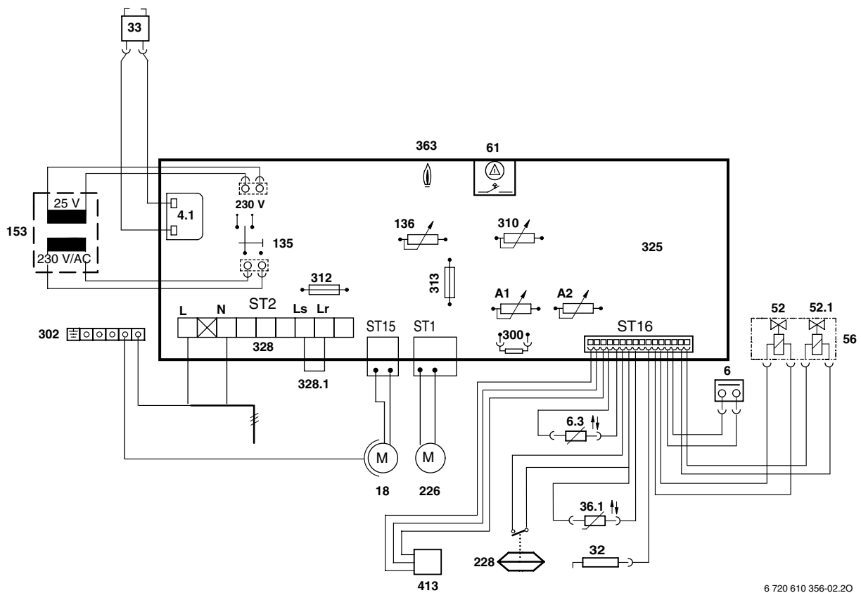
Fig. 2 Cableado eléctrico
