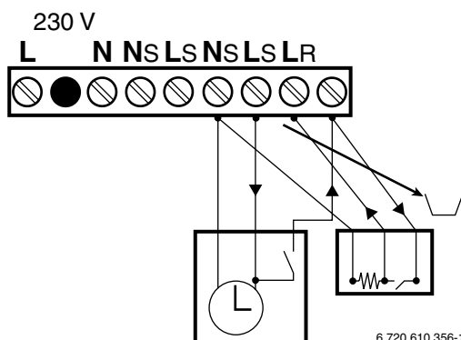
Fig. 19 Conexión del termostato ambiente 230 V y del reloj programador 230 V (retirar el puente entre L_S y L_R )
