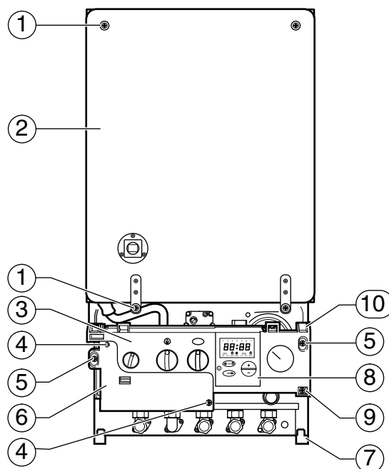
Fig. 40 Sujeción de la cámara de combustión y de la Eurotronic
