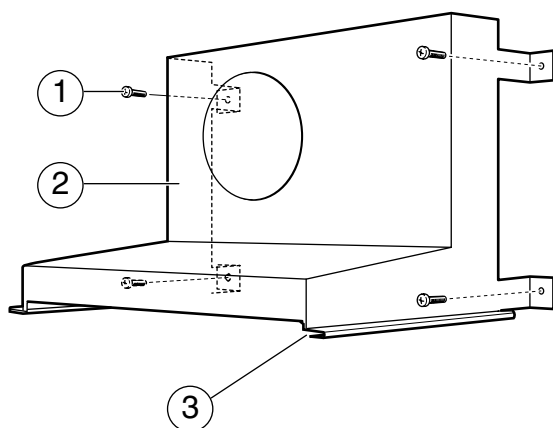
Fig. 44 Campana de evacuación
