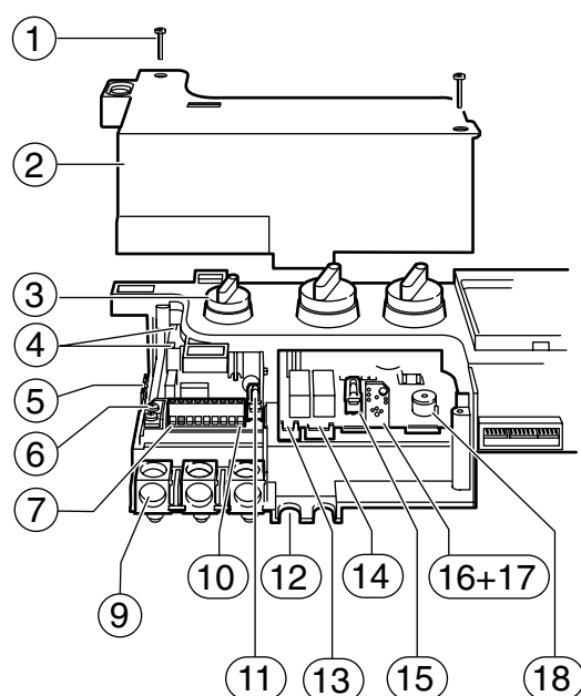
Fig. 13 Conexiones en la Eurotronic
