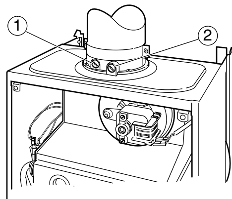
Fig. 38 Medición de los productos de la combustión
