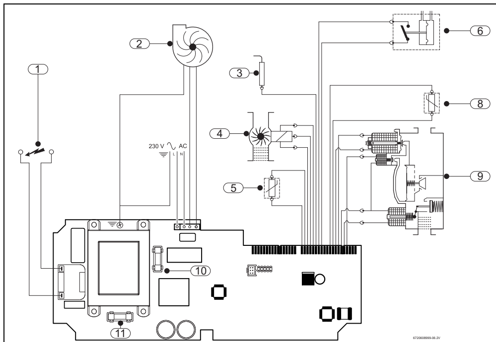
Fig. 4 Esquema eléctrico
