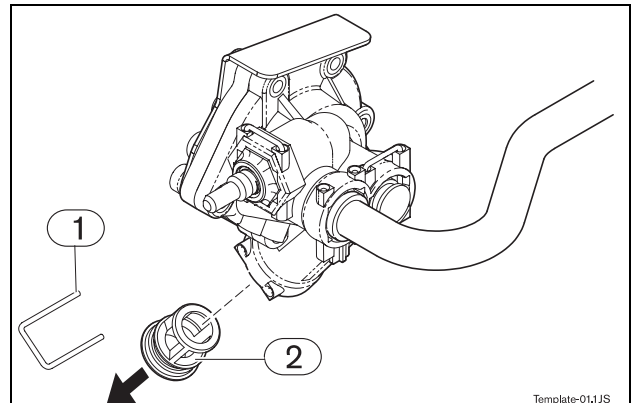
Fig. 13 Purga
