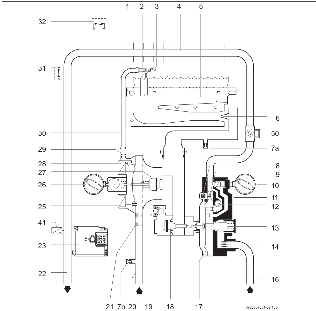
Fig. 2 Esquema técnico
