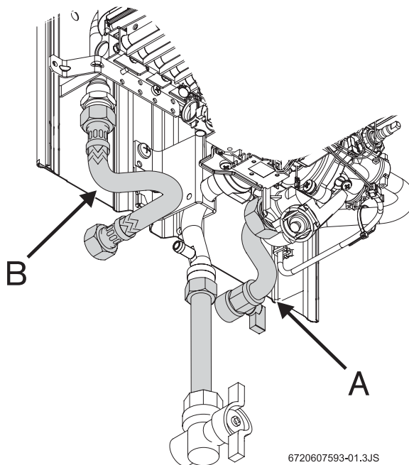
Fig. 5 Conexión del agua
