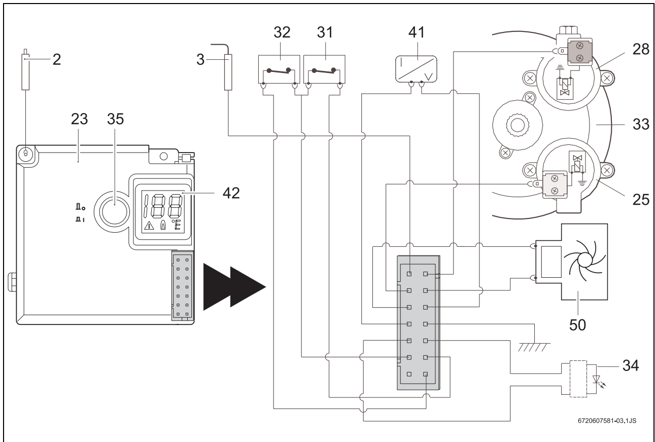
Fig. 3 Esquema eléctrico
