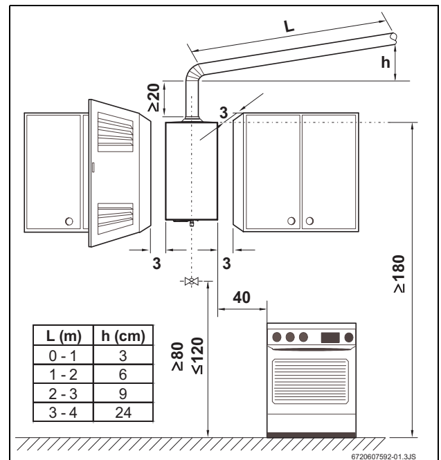
Fig. 4 Separaciones mínimas (en cm)
