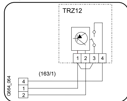
Fig. 8 - Conexión del cronotermóstato. (Previamente eliminar puente entre 1 y 4, fig. 7, pos. 163/1)
