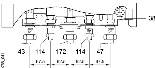
Plantilla de montaje sobre pared
