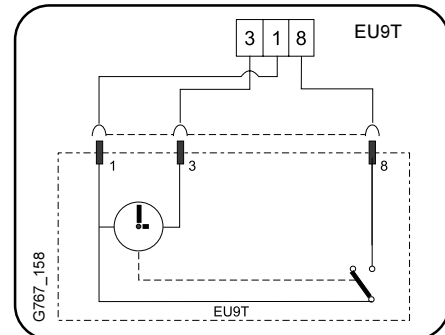
Fig. 9 - Conexión del reloj (Previamente eliminar puente entre 1 y 8, fig. 7, pos. 315)
