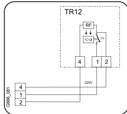
Fig. 7 - Conexión del termostato ambiente. (Previamente eliminar puente entre 1 y 4, fig 7, pos 163/1).
