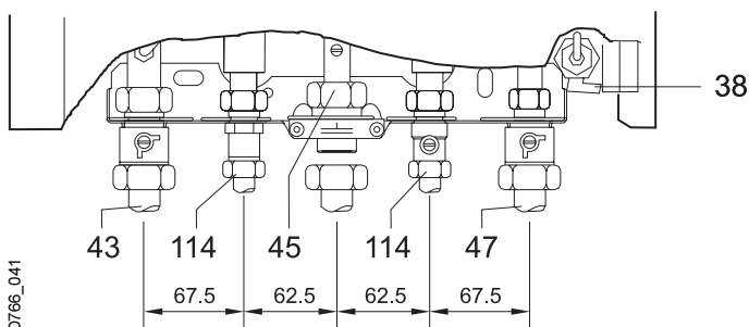
Plantilla de montaje sobre pared
