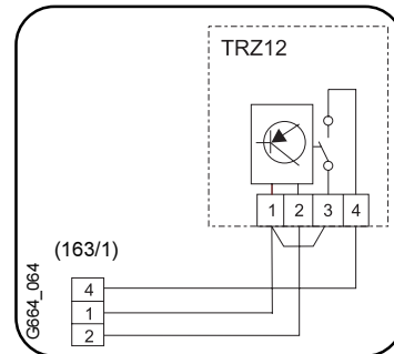
Fig. 8 - Conexión del cronotermostato. (Previamente eliminar puente entre 1 y 4, fig. 6, pos. 163/1)
