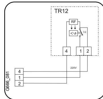
Fig. 7 - Conexión del termostato ambiente. (Previamente eliminar puente entre 1 y 4, fig 6, pos 163/1).
