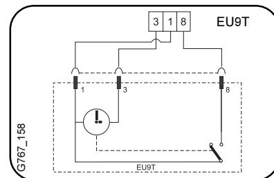
Fig. 9 - Conexión del reloj (Previamente eliminar puente entre 1 y 8, fig. 6, pos. 315)
