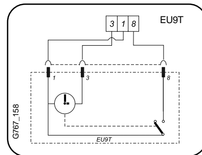
Fig. 9 - Conexión del reloj (Previamente eliminar puente entre 1 y 8, fig. 6, pos. 315)
